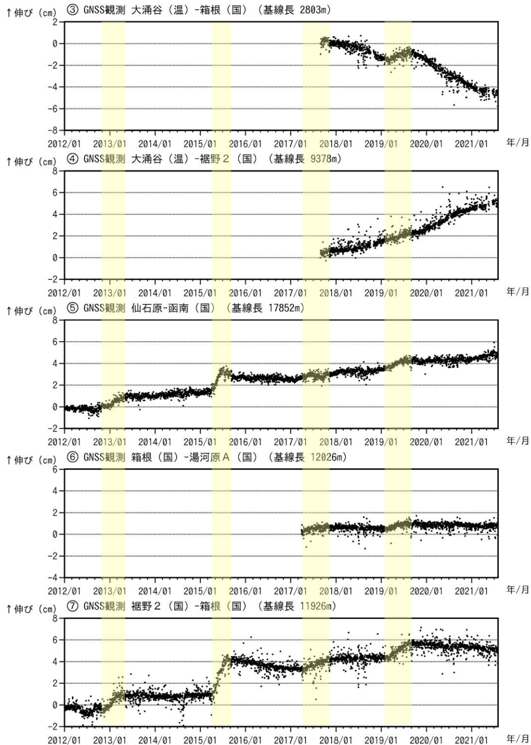
図5-2 箱根山 火山活動経過図（2012年1月1日～2021年7月31日）
