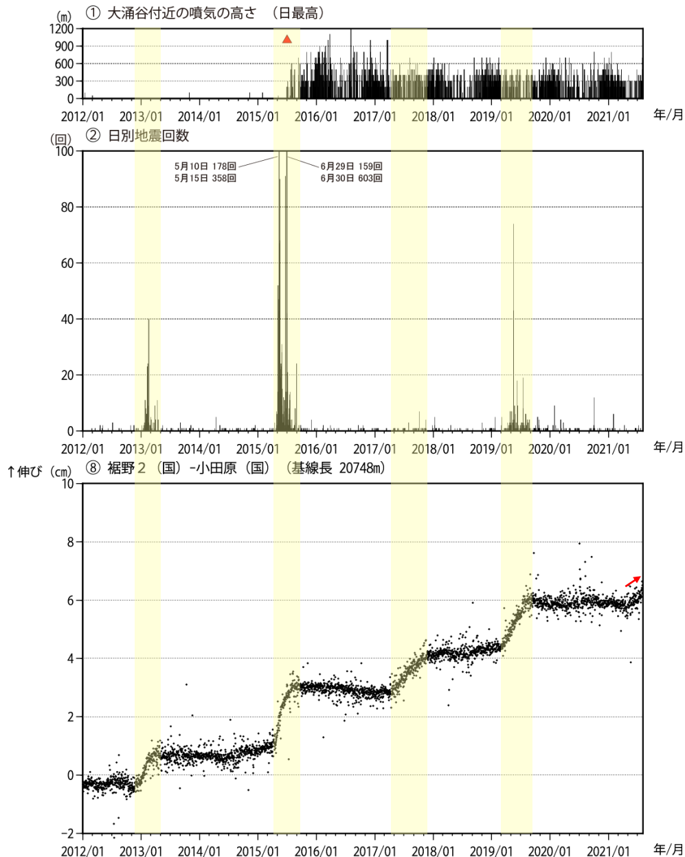
図5-1 箱根山 火山活動経過図（2012年1月1日～2021年7月31日）
