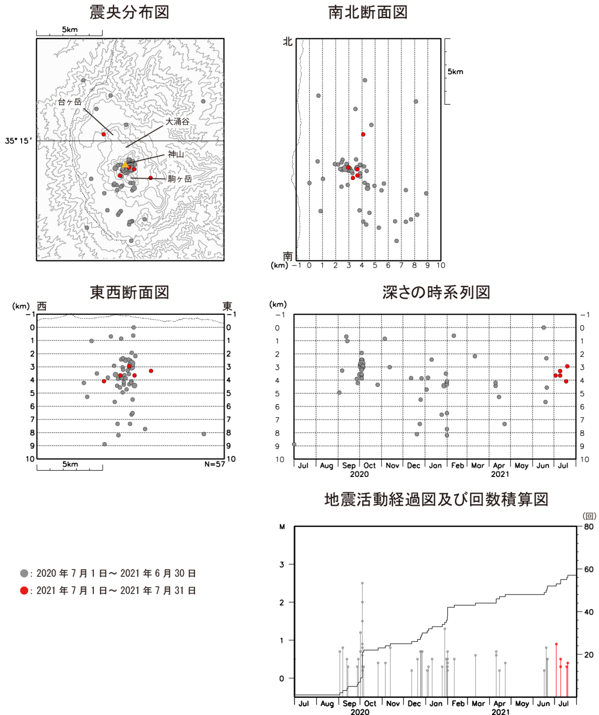
図6 箱根山 広域地震観測網による山体周辺の震源分布図（2020年7月1日～2021年7月31日）
