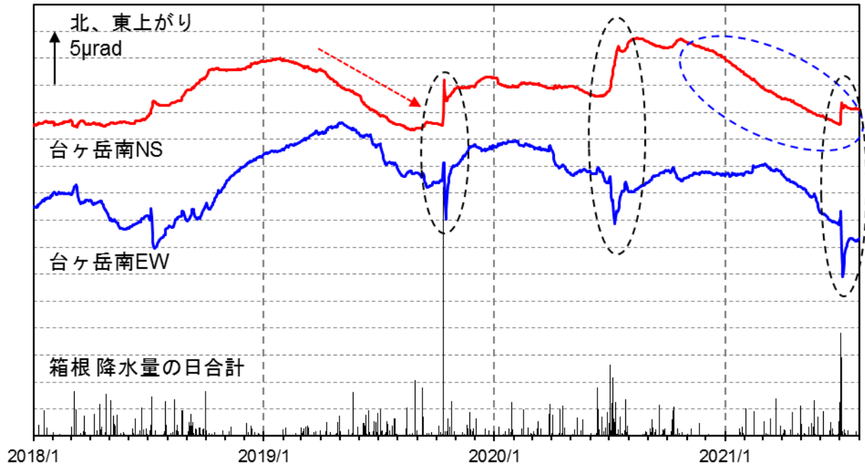
図7 箱根山 台ヶ岳南観測点における傾斜データ（2018年1月1日～2021年7月31日）
