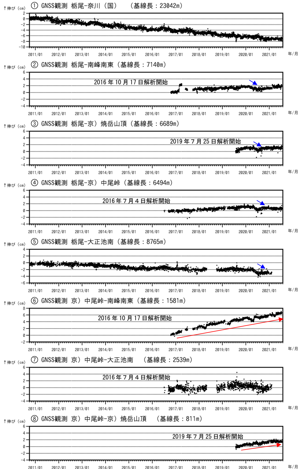
図5 焼岳 GNSS連続観測による基線長変化（2010年10月1日～2021年7月31日）
