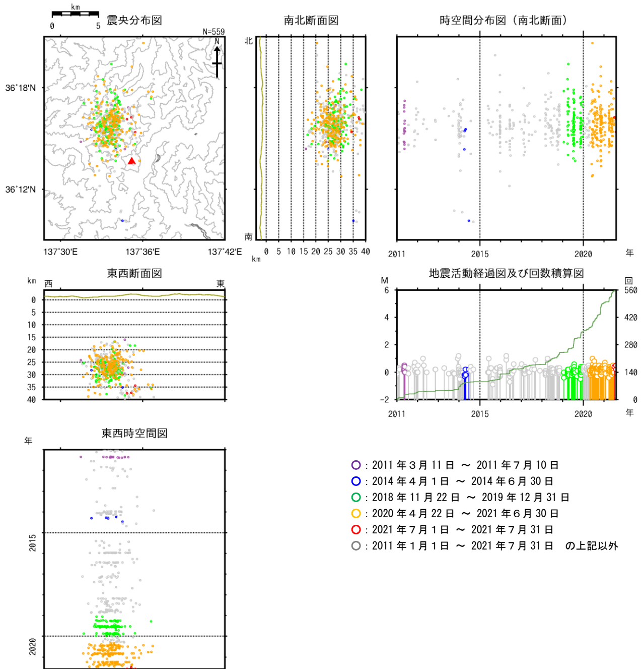
図9 焼岳 広域地震観測網による深部低周波地震の震源分布図（2011年1月1日～2021年7月31日） 広域地震観測網により震源決定したもので、深さは全て海面以下として決定しています。そのため、山頂付近の浅い地震の震源も海面下に決定されています。
