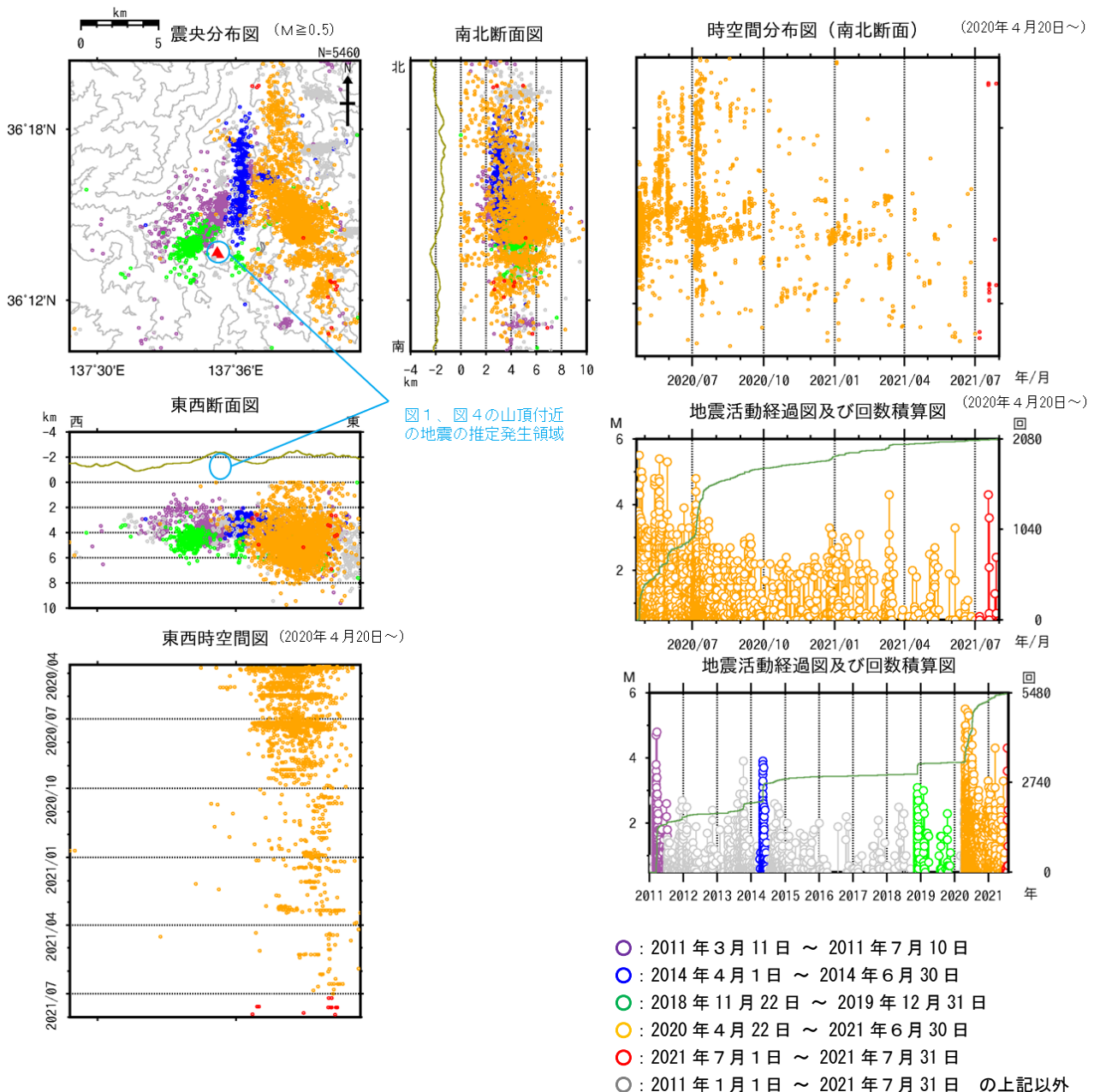
図8 焼岳 広域地震観測網による山体及び周辺の地震活動(2011年1月1日～2021年7月31日)
