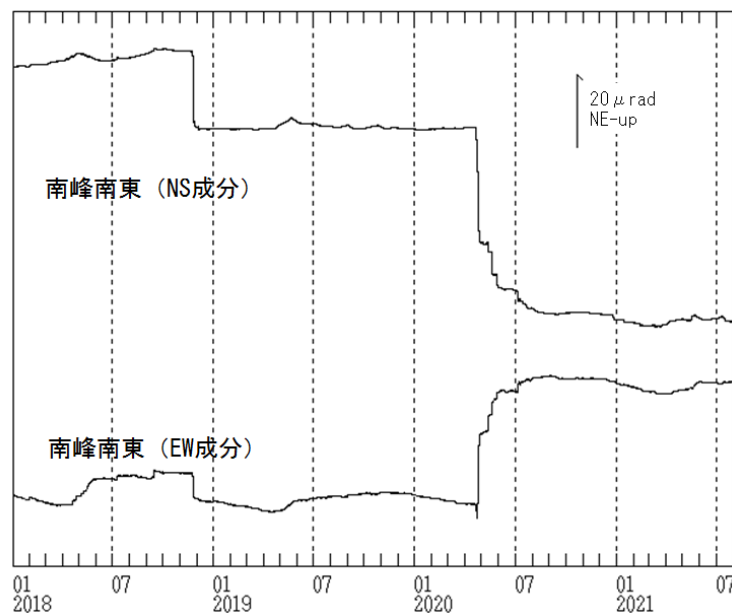
図7 焼岳 南峰南東観測点における傾斜データ（2018年1月1日～2021年7月31日）
