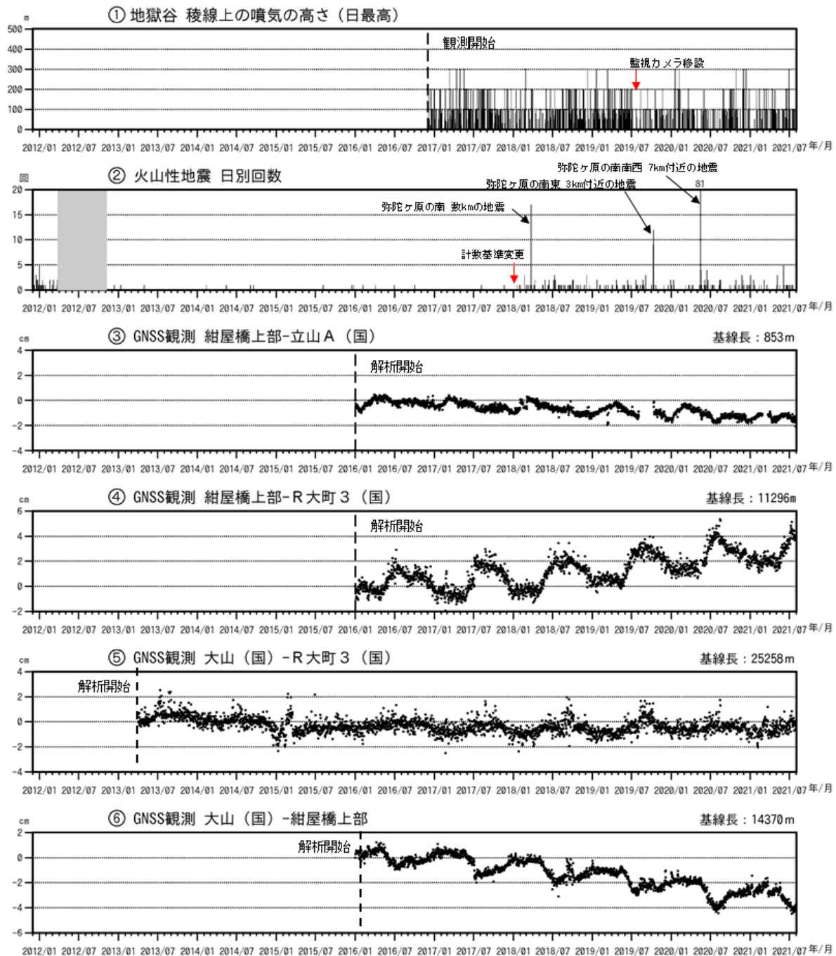
図3 弥陀ヶ原 火山活動経過図（2011年12月1日～2021年7月31日）
