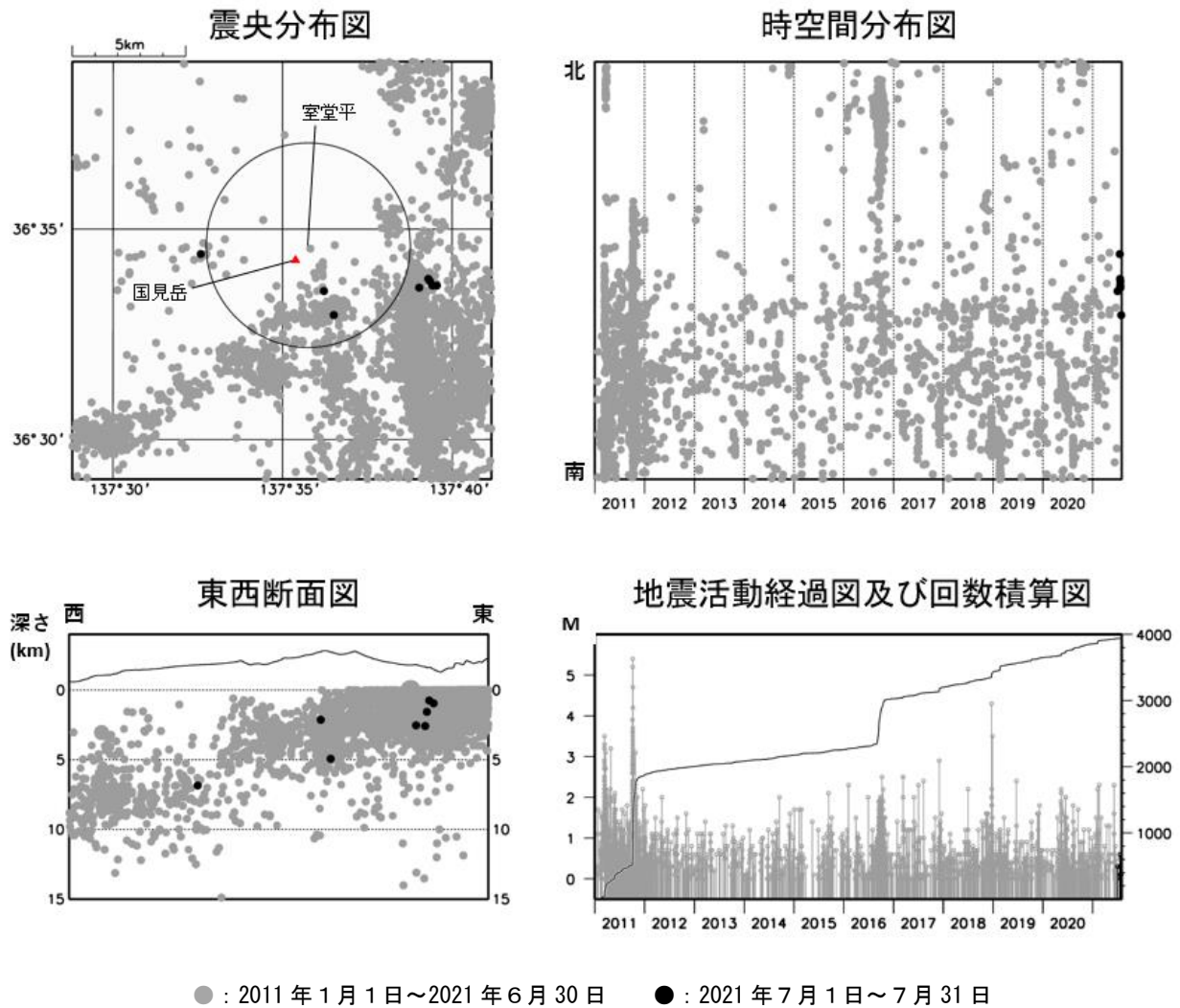
図2 弥陀ヶ原 広域地震観測網による山体・周辺の地震活動（2011年1月1日～2021年7月31日） 震央分布図中の円は弥陀ヶ原の計数対象地震（室堂平でS-P時間1秒以内）のおよその範囲を示しています。 広域地震観測網により震源決定したもので、深さは全て海面以下として決定しています。 図中の震源要素は一部暫定値が含まれており、後日変更することがあります。 この図では、関係機関の地震波形を一元的に処理し、地震観測点の標高を考慮する等した新手法で得られた震源を用いています（ただし、2020年8月以前の地震については火山活動評価のための参考震源です）。 2021年8月10日現在、次の期間の地震について、暫定的に震源精査の基準を変更しているため、その前後の期間と比較して微小な地震での震源決定数の変化（増減）が見られます。 (1) 2020年4月18日から10月23日まで、(2) 2021年1月9日から3月7日まで、(3) 2021年4月19日以降
