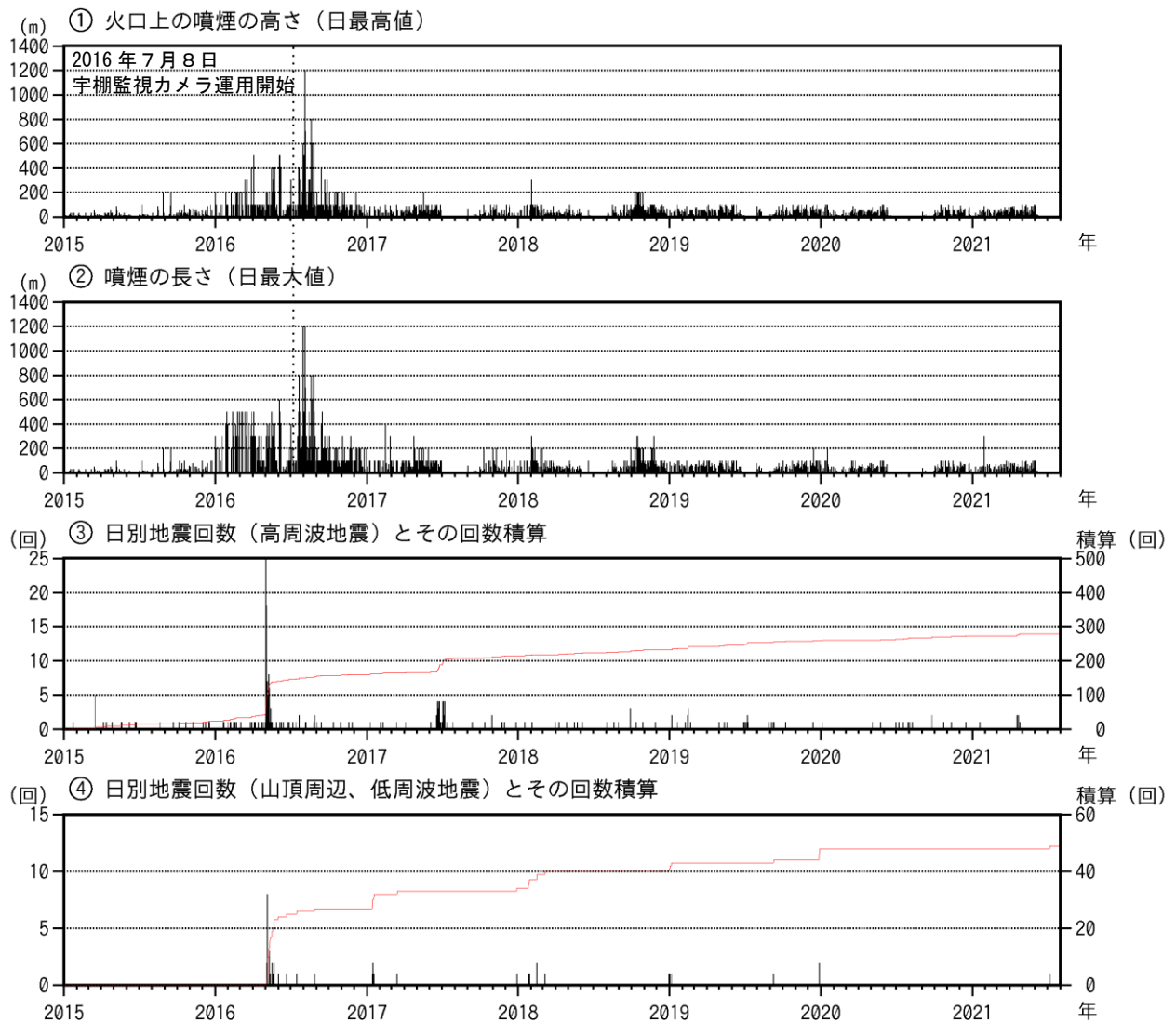
図3 新潟焼山 火山活動経過図（短期）（2015年1月1日～2021年7月31日）
