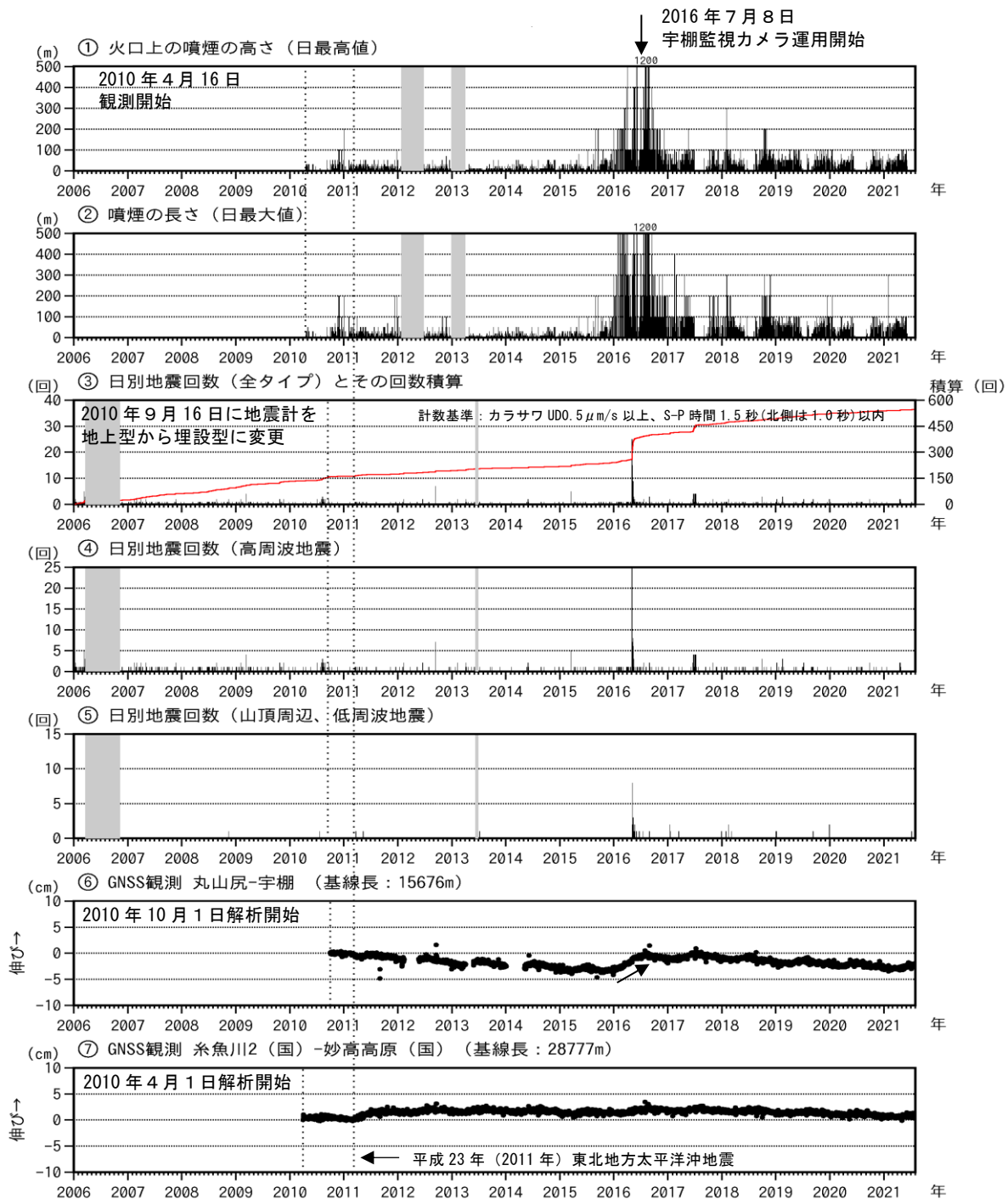
図2 新潟焼山 火山活動経過図（2006年1月1日～2021年7月31日）
