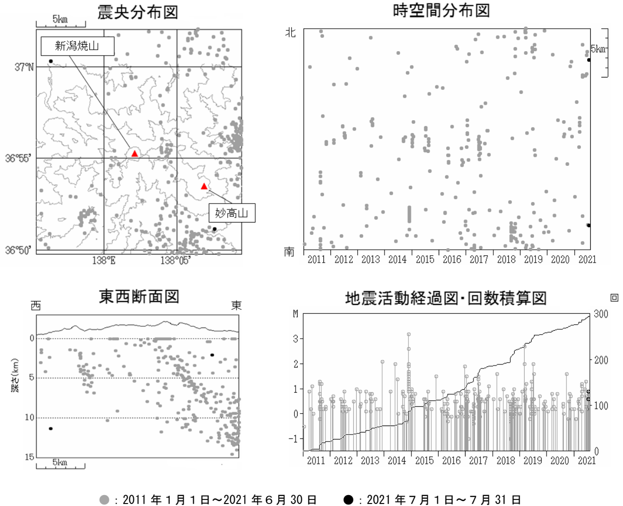
図4 新潟焼山 広域地震観測網による山体・周辺の地震活動（2011年1月1日～2021年7月31日）
