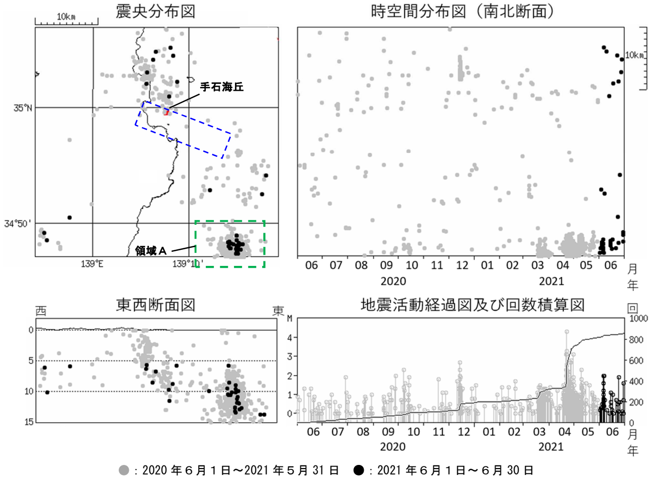
図2 伊豆東部火山群 広域地震観測網による震源分布図（2020年6月1日～2021年6月30日） □の領域は群発地震活動の発生する可能性がある範囲（火口が発生する可能性のある範囲）を示しています。 https://www.data.jma.go.jp/svd/vois/data/tokyo/STOCK/level/PDF/level_316.pdf 広域地震観測網により震源決定したもので、深さは全て海面以下として決定しています。 M（マグニチュード）は地震の規模を表し、M0.0以上を表示しています。 図中の震源要素は一部暫定値が含まれており、後日変更することがあります。 この図では、関係機関の地震波形を一元的に処理し、地震観測点の標高を考慮する等した新手法で得られた震源を用いています（ただし、2020年8月以前の地震については火山活動評価のための参考震源です）。 2021年7月8日現在、次の期間の地震について、暫定的に震源精査の基準を変更しているため、その前後の期間と比較して微小な地震での震源決定数の変化（増減）が見られます。 (1)2020年4月18日から10月23日まで、(2)2021年1月9日から3月7日まで、(3)2021年4月19日以降
