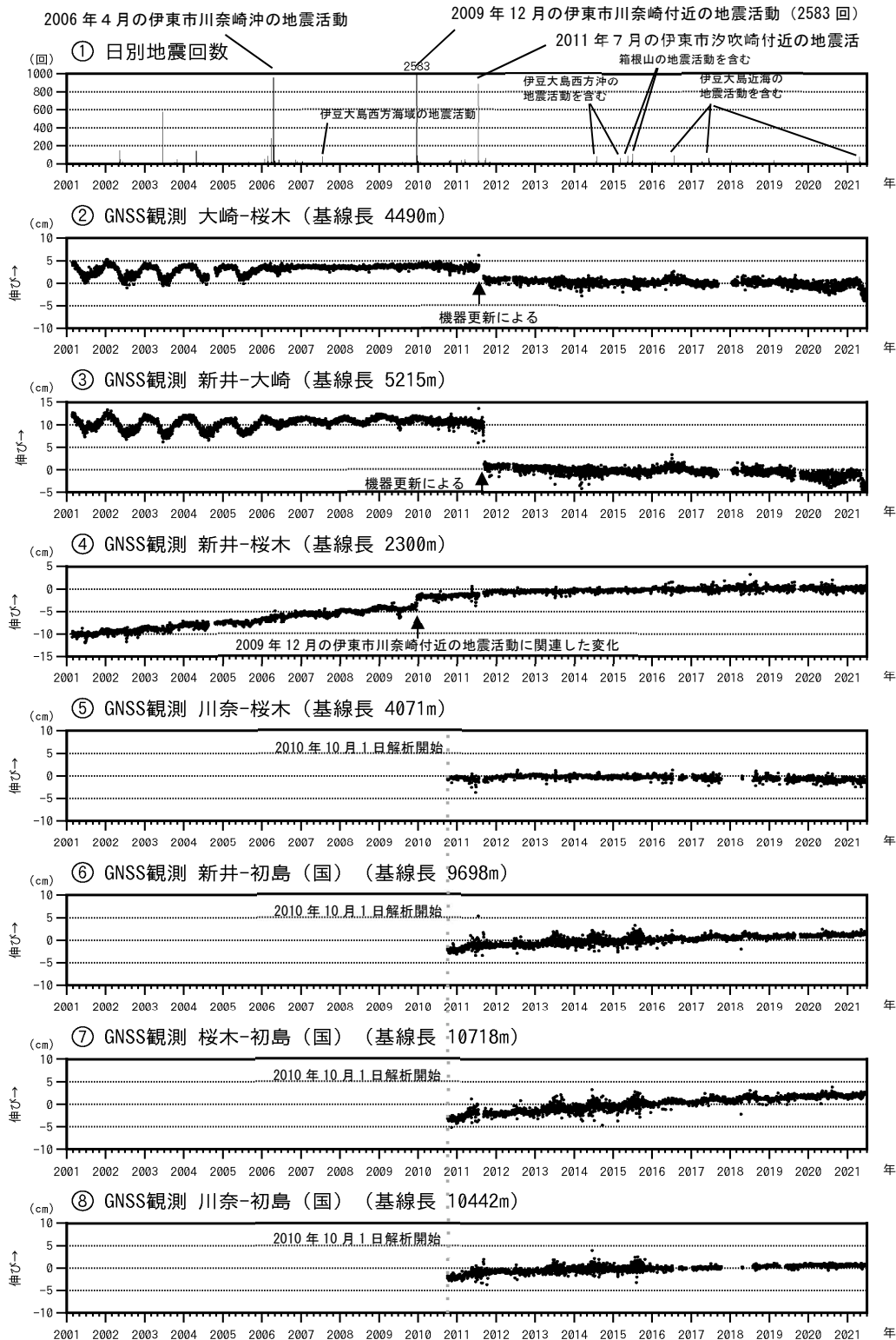
図3 伊豆東部火山群 火山活動経過図（2001年1月1日～2021年6月30日）
