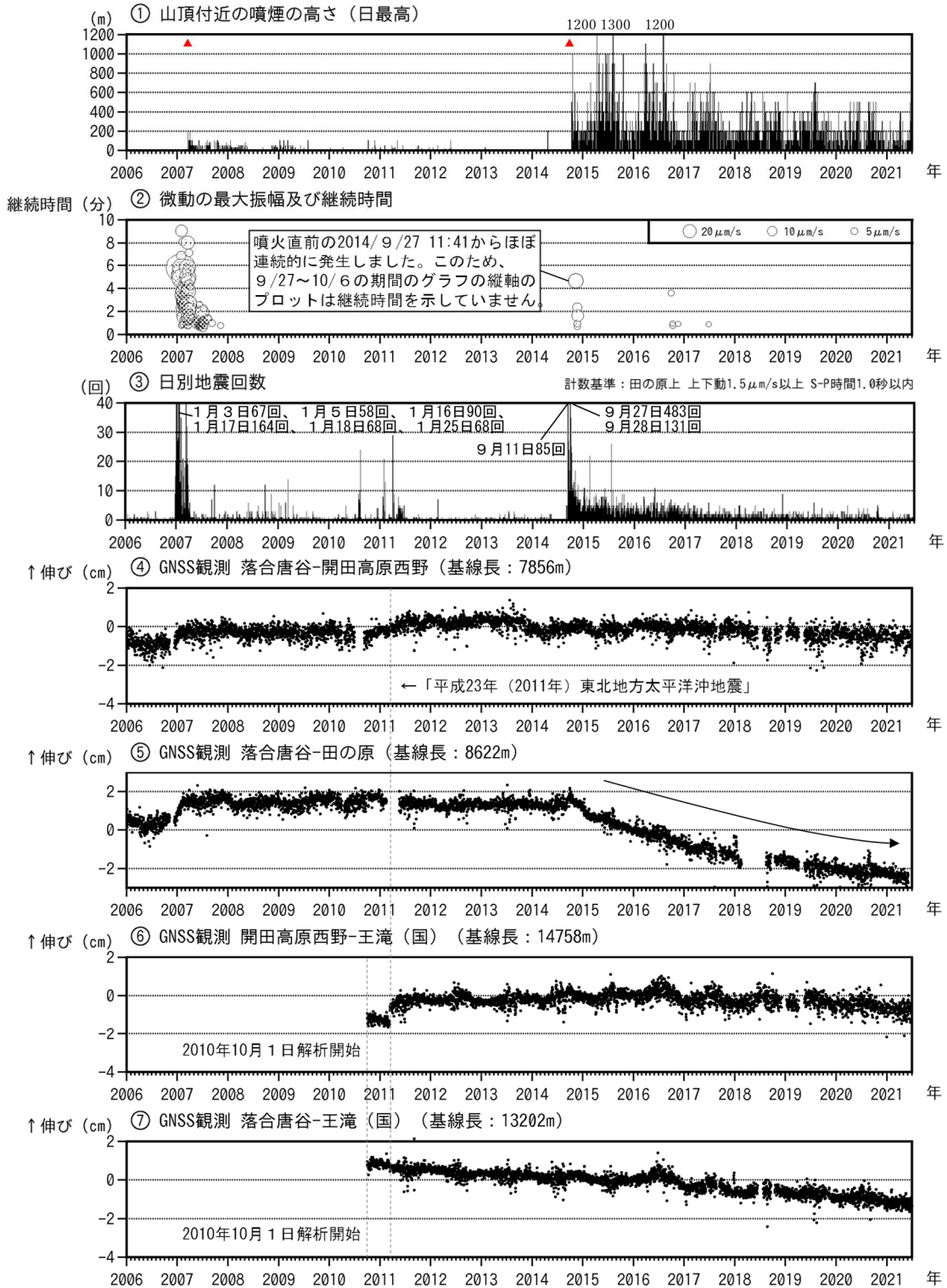
図5 御嶽山 長期間の火山活動経過図（2006年1月1日～2021年6月30日）
