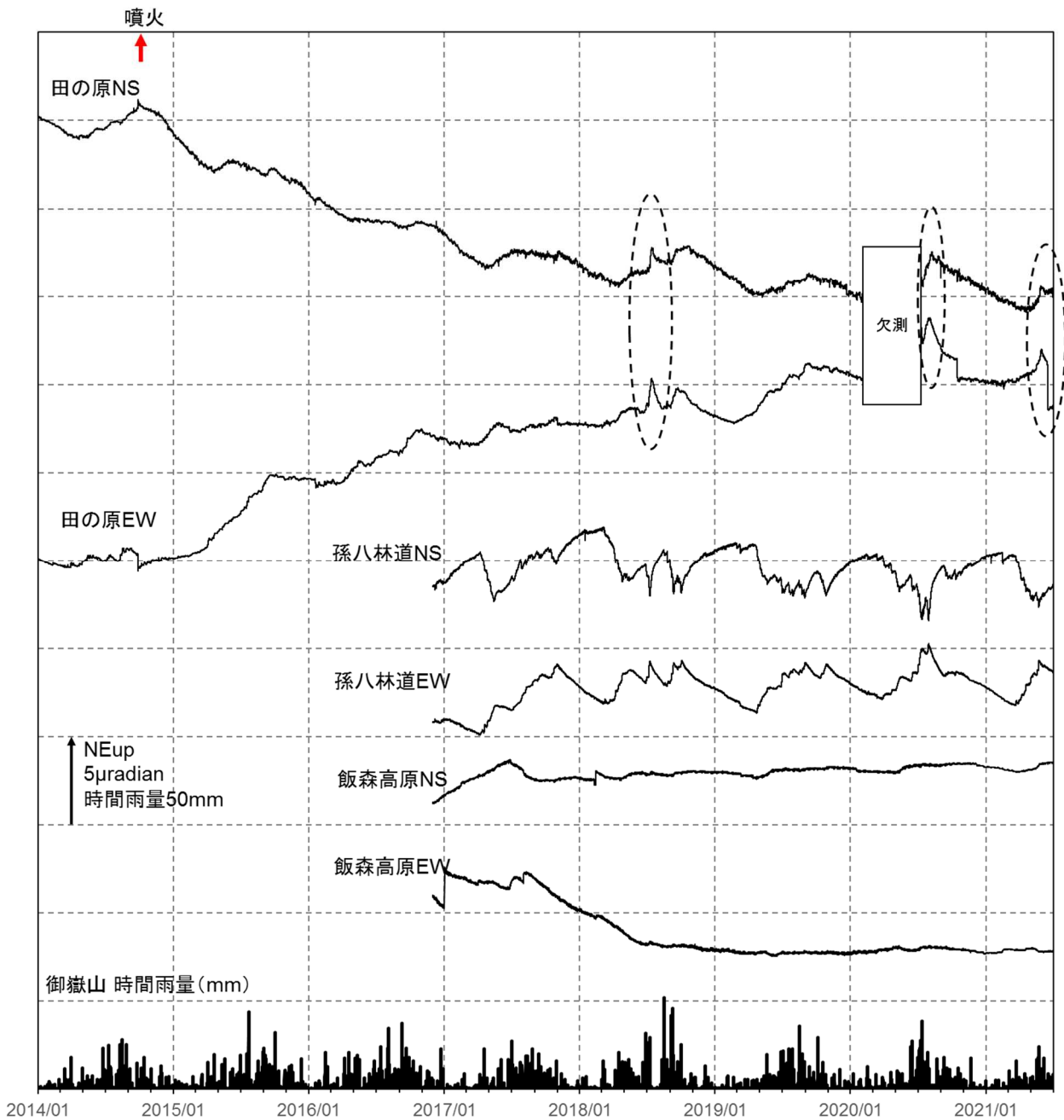
図7 御嶽山 傾斜変動（2014年1月1日～2021年6月30日）
