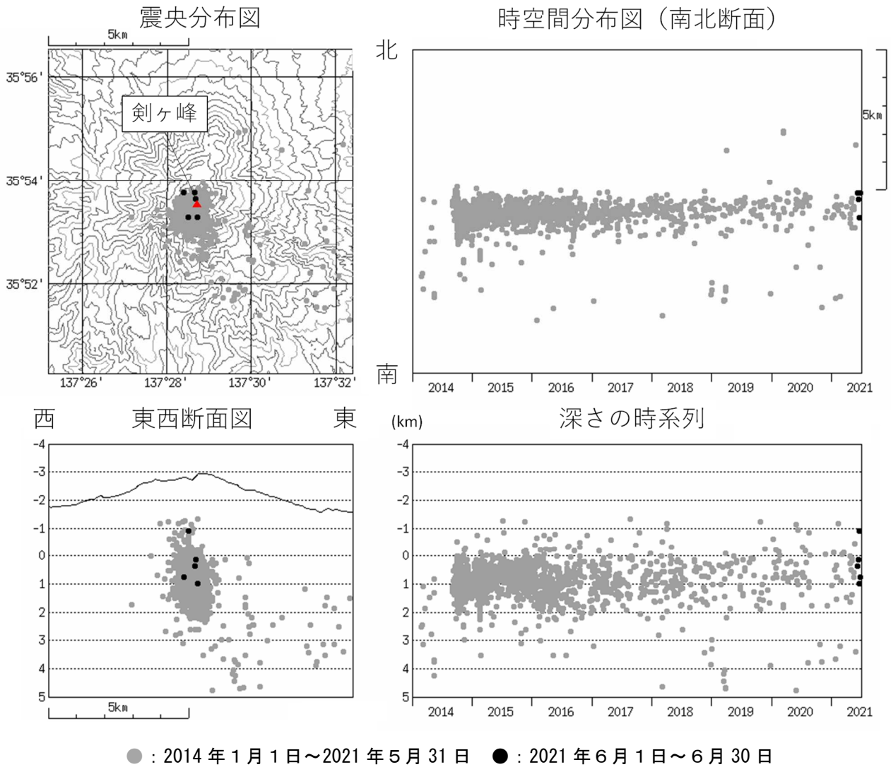
図3 御嶽山 震源分布図（2014年1月1日～2021年6月30日）
