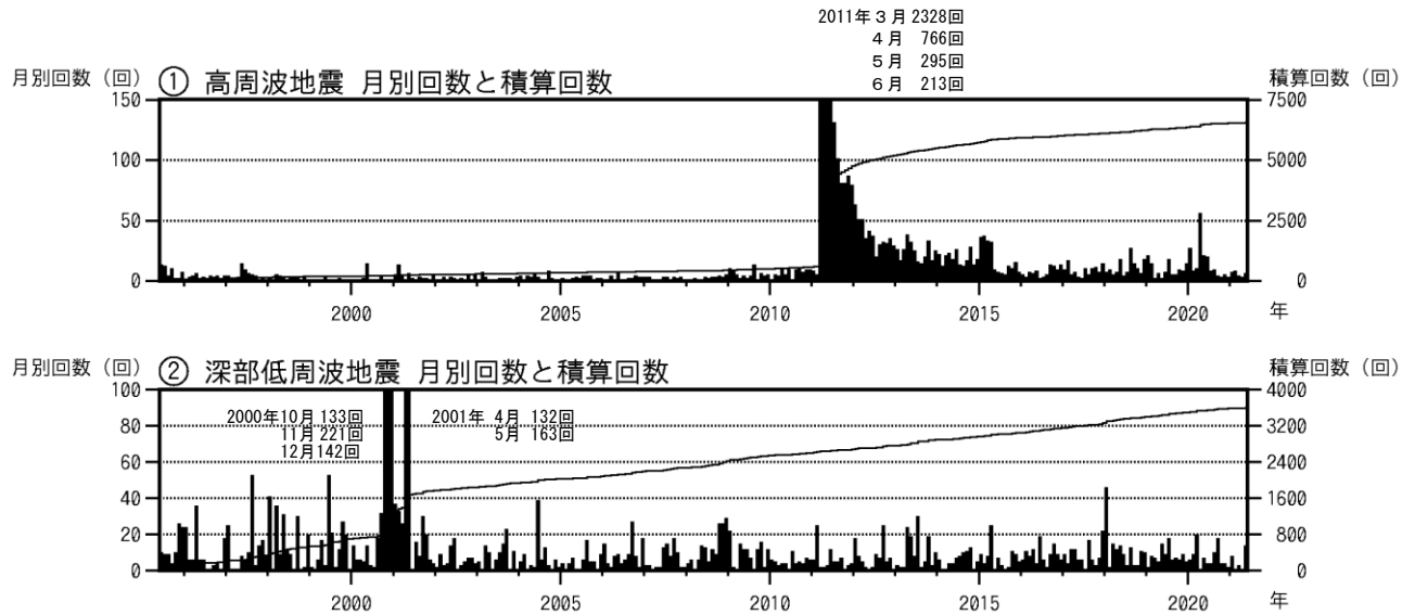
図2 富士山 月別地震回数（1995年6月1日～2021年5月31日）
