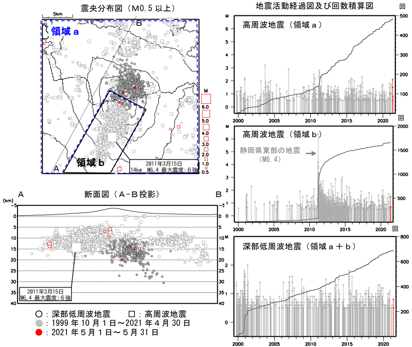
図3 富士山 広域地震観測網による山体及び周辺の地震活動(1999年10月1日~2021年5月31日)
