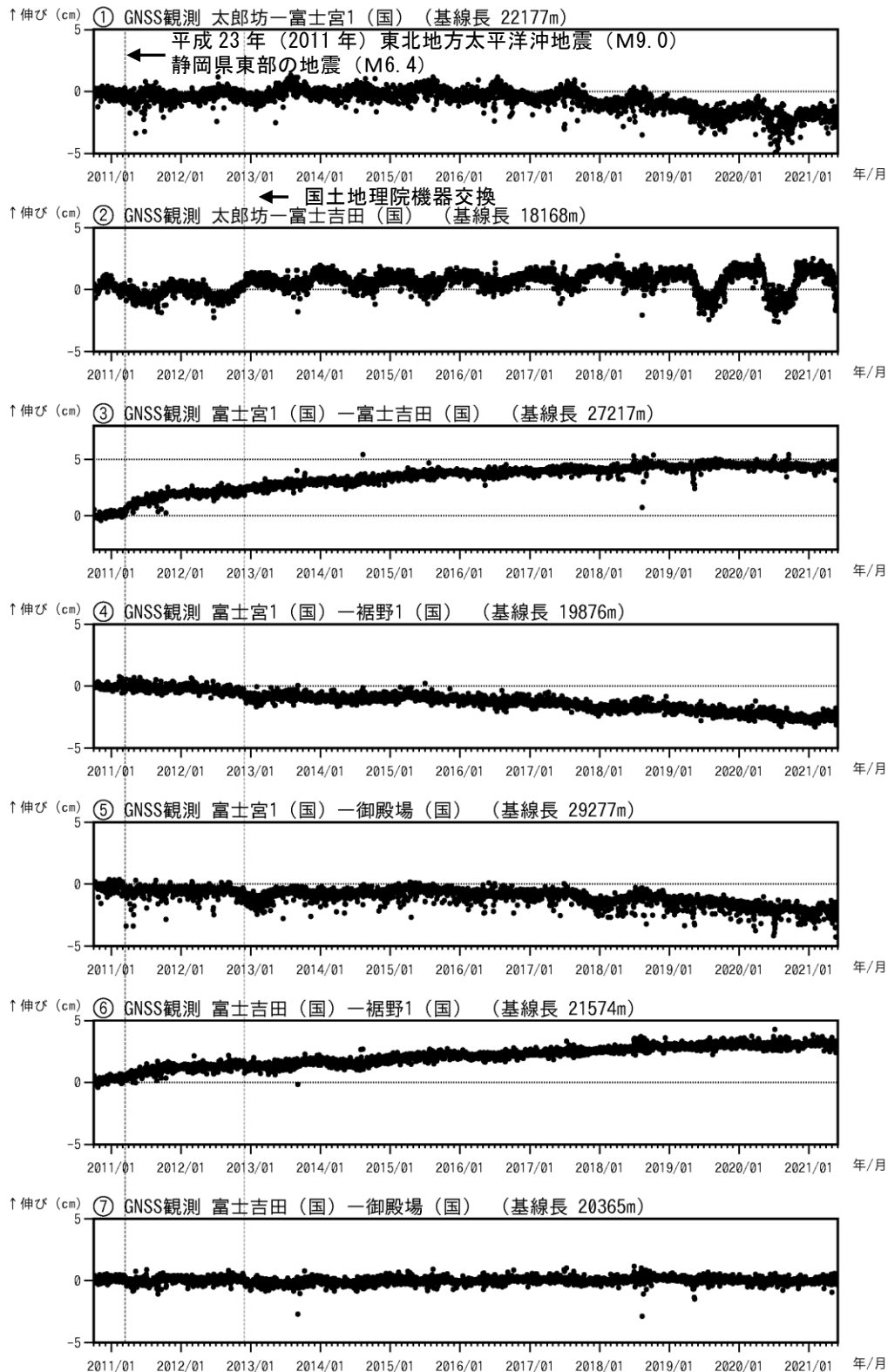
図4 富士山 GNSS 連続観測による基線長変化 (2010 年 10 月 1 日～2021 年 5 月 31 日) (国): 国土地理院 「平成 23 年 (2011 年) 東北地方太平洋沖地震」及び 2011 年 3 月 15 日に発生した静岡県東部の地震 (M 6.4) によるステップ状の変化を補正しています。 ①～⑦は図5の GNSS 基線①～⑦に対応しています。 ・火山活動によるとみられる変動は認められません。
