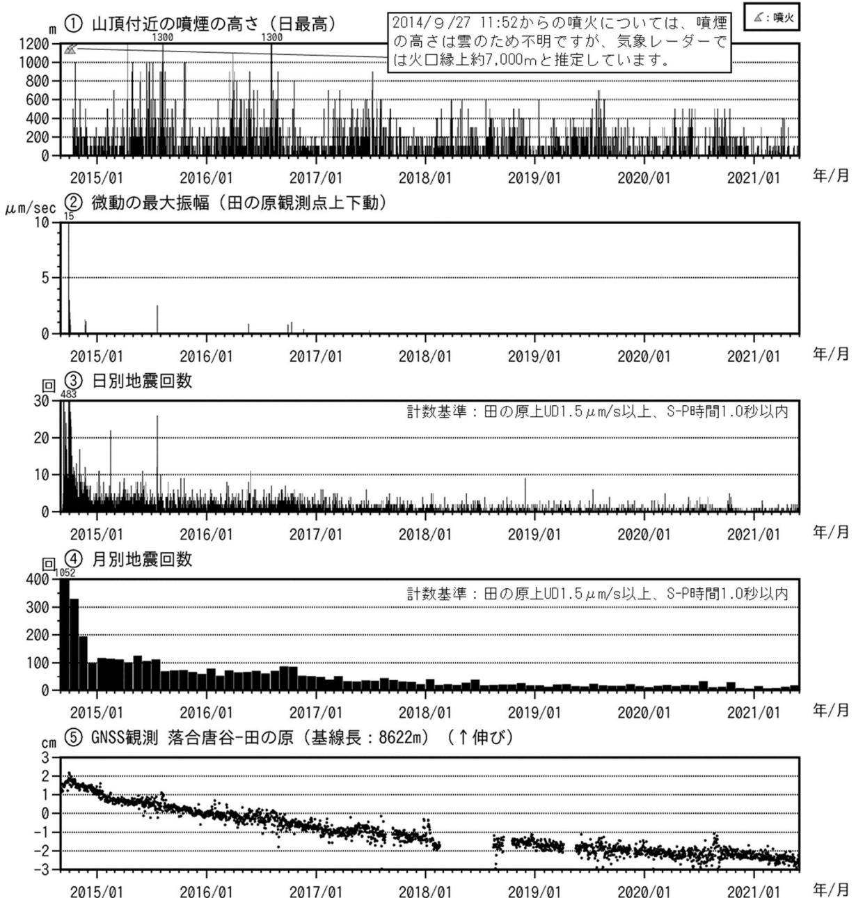
図4 御嶽山 最近の火山活動経過図（2014年9月1日～2021年5月31日）
