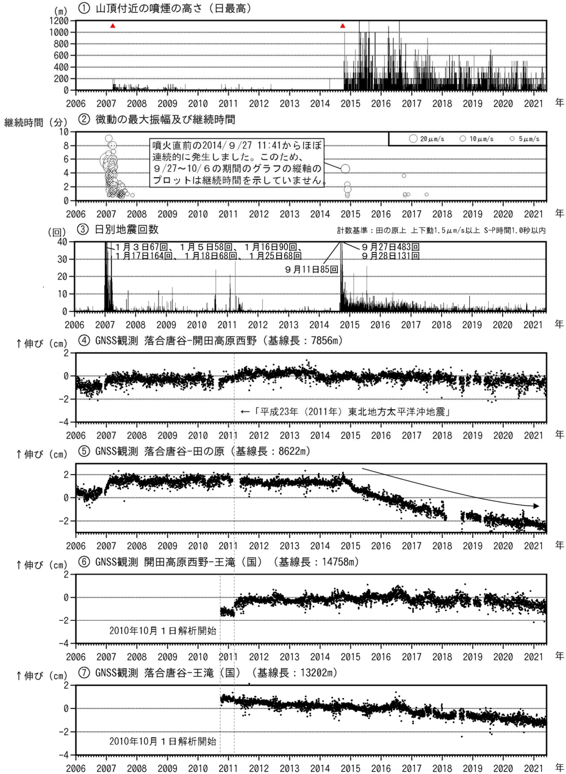
図5 御嶽山 長期間の火山活動経過図（2006年1月1日～2021年5月31日）
