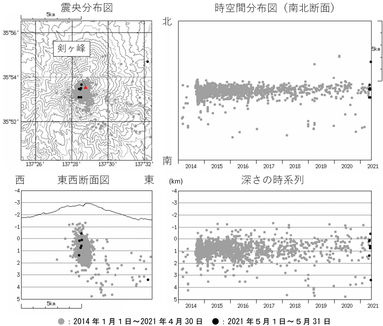
図3 御嶽山 震源分布図（2014年1月1日～2021年5月31日）
