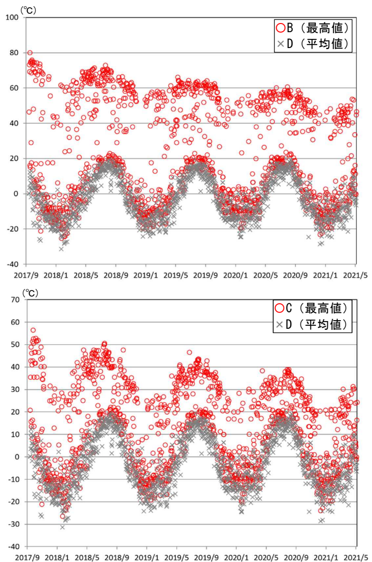
図2 御嶽山 奥の院赤外熱映像カメラによる剣ヶ峰南西側における最高温度の推移
