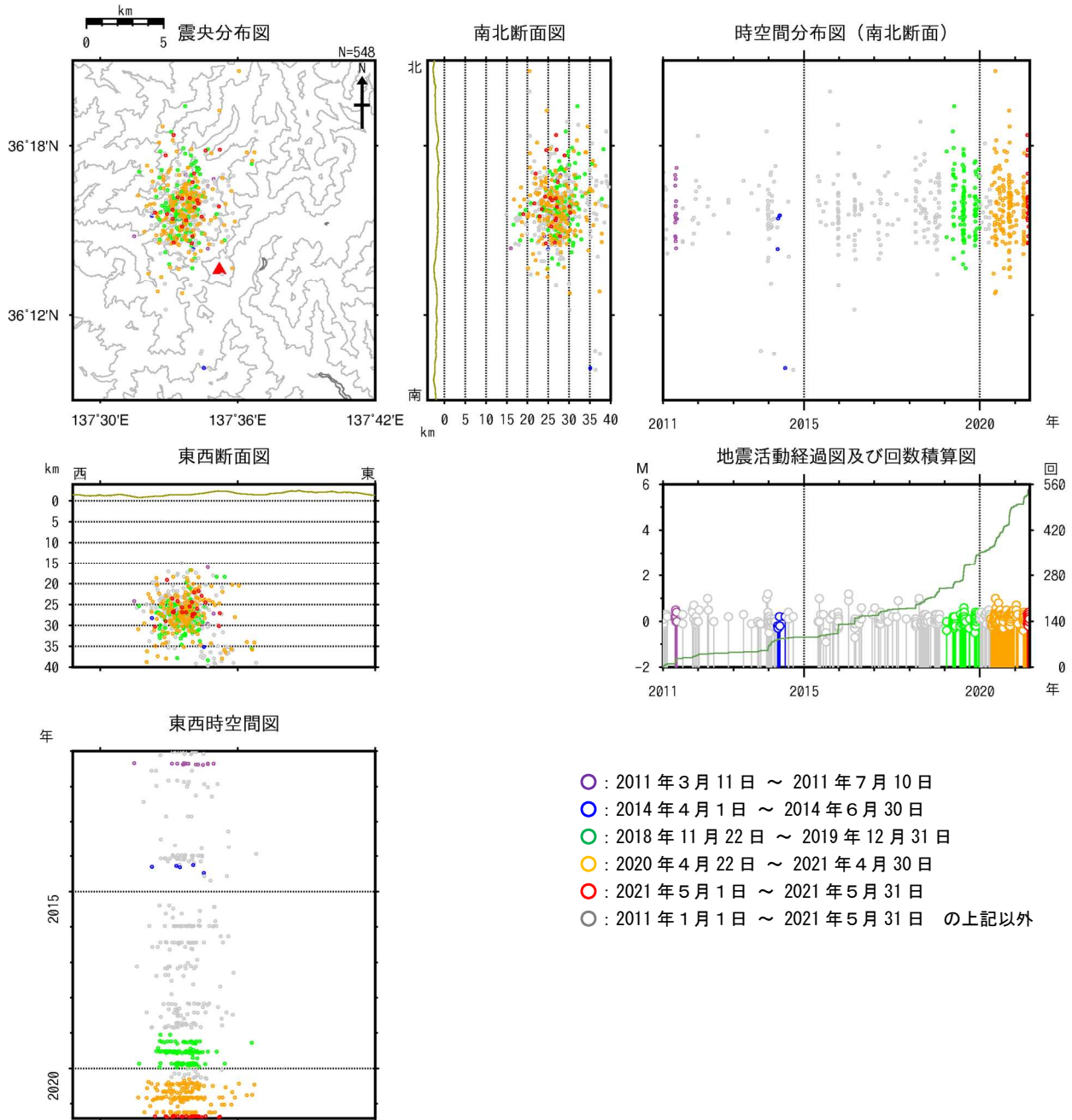
図3 焼岳 広域地震観測網による深部低周波地震の震源分布図（2011年1月1日～2021年5月31日） 広域地震観測網により震源決定したもので、深さは全て海面以下として決定しています。そのため、山頂付近の浅い地震の震源も海面下に決定されています。
