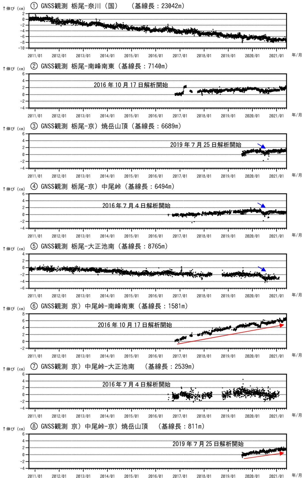
図7 焼岳 GNSS連続観測による基線長変化（2010年10月1日～2021年5月31日）
