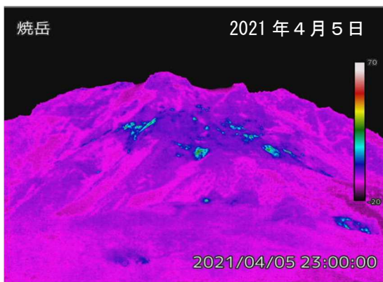
図5 焼岳 中尾峠赤外熱映像カメラによる焼岳の北側斜面の地表面温度分布と可視画像
