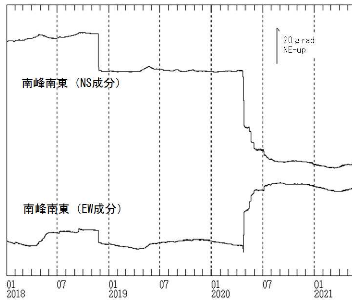
図9 焼岳 南峰南東観測点における傾斜データ（2018年1月1日～2021年5月31日）
