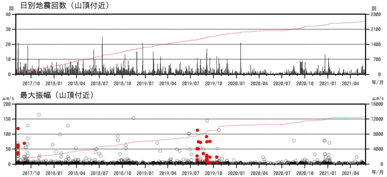
図1 焼岳 山頂付近の地震回数、及び南峰南東観測点上下動最大振幅 （2017年8月1日～2021年5月31日）
