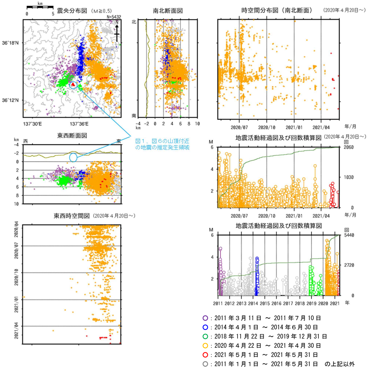
図2 焼岳 広域地震観測網による山体及び周辺の地震活動(2011年1月1日～2021年5月31日)
