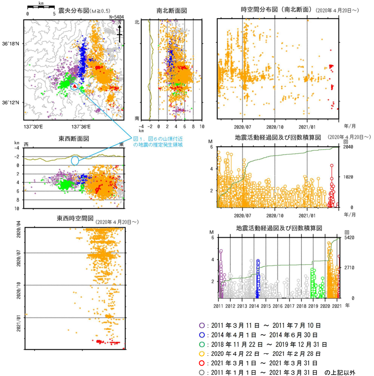
図2 焼岳 広域地震観測網による山体及び周辺の地震活動(2011年1月1日～2021年3月31日)
