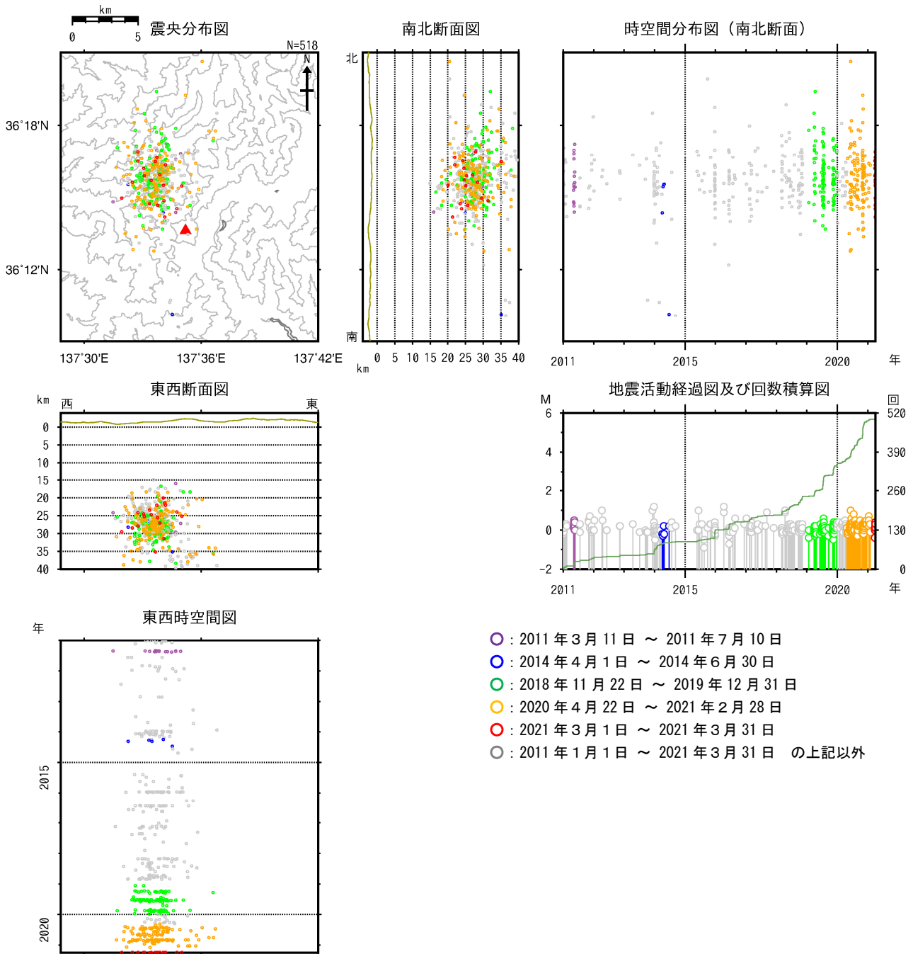
図3 焼岳 広域地震観測網による深部低周波地震の震源分布図（2011年1月1日～2021年3月31日） 広域地震観測網により震源決定したもので、深さは全て海面以下として決定しています。そのため、山頂付近の浅い地震の震源も海面下に決定されています。 M（マグニチュード）は地震の規模を表します。 図中の震源要素は一部暫定値が含まれており、後日変更することがあります。 2021年4月8日現在、2020年4月18日から10月23日まで、及び2021年1月9日から3月7日までの地震について、暫定的に震源精査の基準を変更しているため、それらの前後の期間と比較して微小な地震での震源決定数の変化（増減）が見られます。 ・ 焼岳の北西側の深い所を震源とする低周波地震は引き続き観測されています。この活動に伴う火山活動の活発化はみられません。 ・ 過去には、図2に示したような焼岳周辺の地震活動の活発化がみられた期間付近で、深部低周波地震が増加したことがあります。
