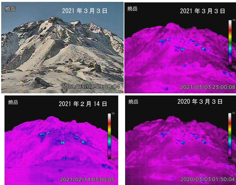
図5 焼岳 中尾峠赤外熱映像カメラによる焼岳の北側斜面の地表面温度分布と可視画像 撮影場所と撮影方向は図10を参照下さい。
