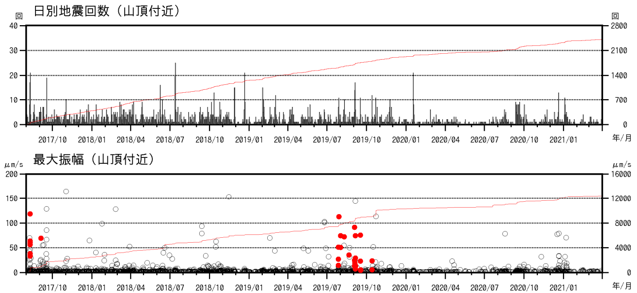
図1 焼岳 山頂付近の地震回数、及び南峰南東観測点上下動最大振幅 (2017年8月1日～2021年3月31日)
