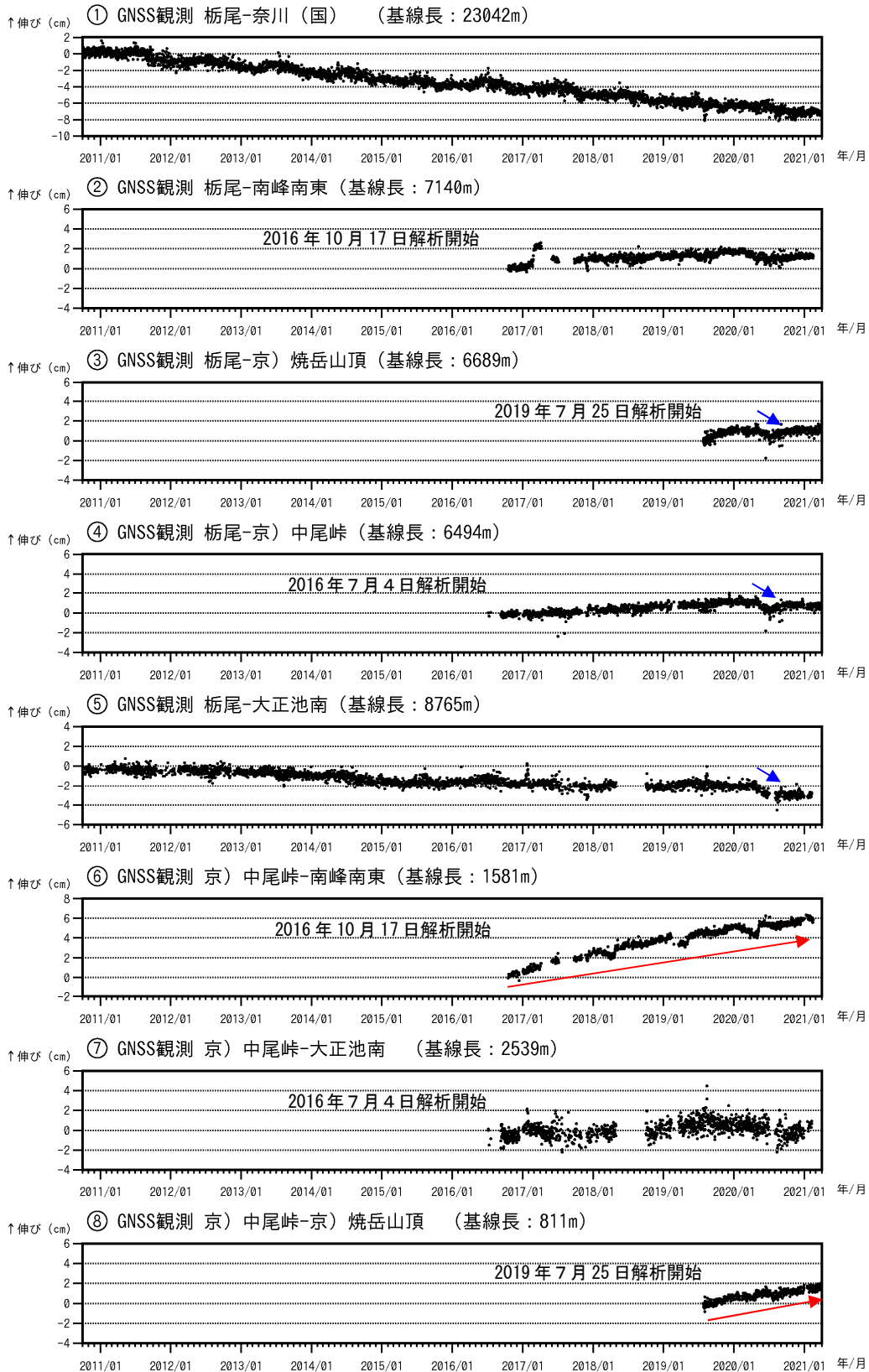
図7 焼岳 GNSS連続観測による基線長変化（2010年10月1日～2021年3月31日）
