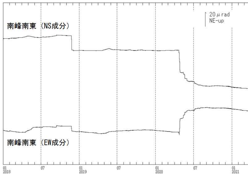
図9 焼岳 南峰南東観測点における傾斜データ（2018年1月1日～2021年2月28日）
