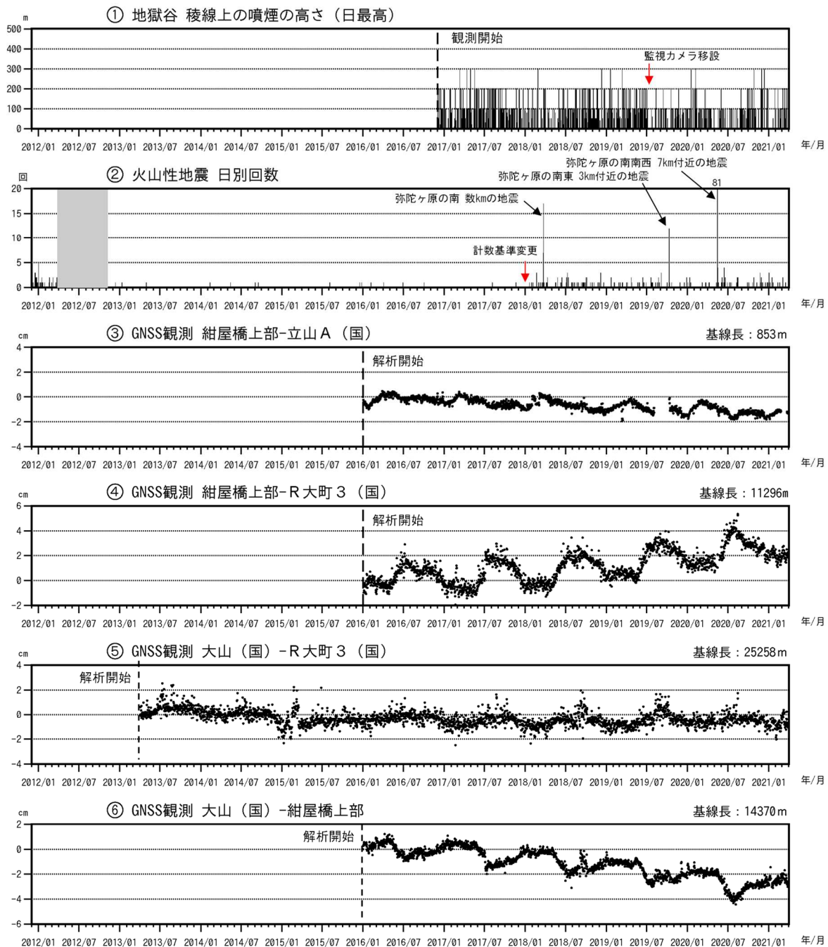
図3 弥陀ヶ原 火山活動経過図（2011年12月1日～2021年3月31日）
