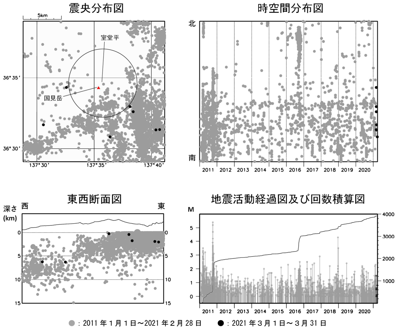
図2 弥陀ヶ原 広域地震観測網による山体・周辺の地震活動（2011年1月1日～2021年3月31日） 震央分布図中の円は弥陀ヶ原の計数対象地震（室堂平でS-P時間1秒以内）のおよその範囲を示しています。 広域地震観測網により震源決定したもので、深さは全て海面以下として決定しています。 図中の震源要素は一部暫定値が含まれており、後日変更することがあります。 この図では、関係機関の地震波形を一元的に処理し、地震観測点の標高を考慮する等した新手法で得られた震源を用いています（ただし、2020年8月以前の地震については火山活動評価のための参考震源です）。 2021年4月8日現在、2020年4月18日から10月23日まで、及び2021年1月9日から3月7日までの地震について、暫定的に震源精査の基準を変更しているため、それらの前後の期間と比較して微小な地震での震源決定数の変化（増減）が見られます。
