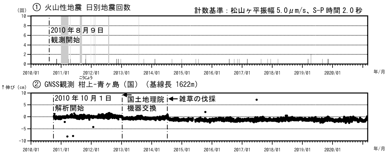
図3 青ヶ島 火山活動経過図(2010年8月9日~2021年2月28日) ① グラフの灰色部分は機器障害による欠測を示す。 ② (国): 国土地理院、図5のGNSS基線②に対応。グラフの空白部分は欠測を示す。
