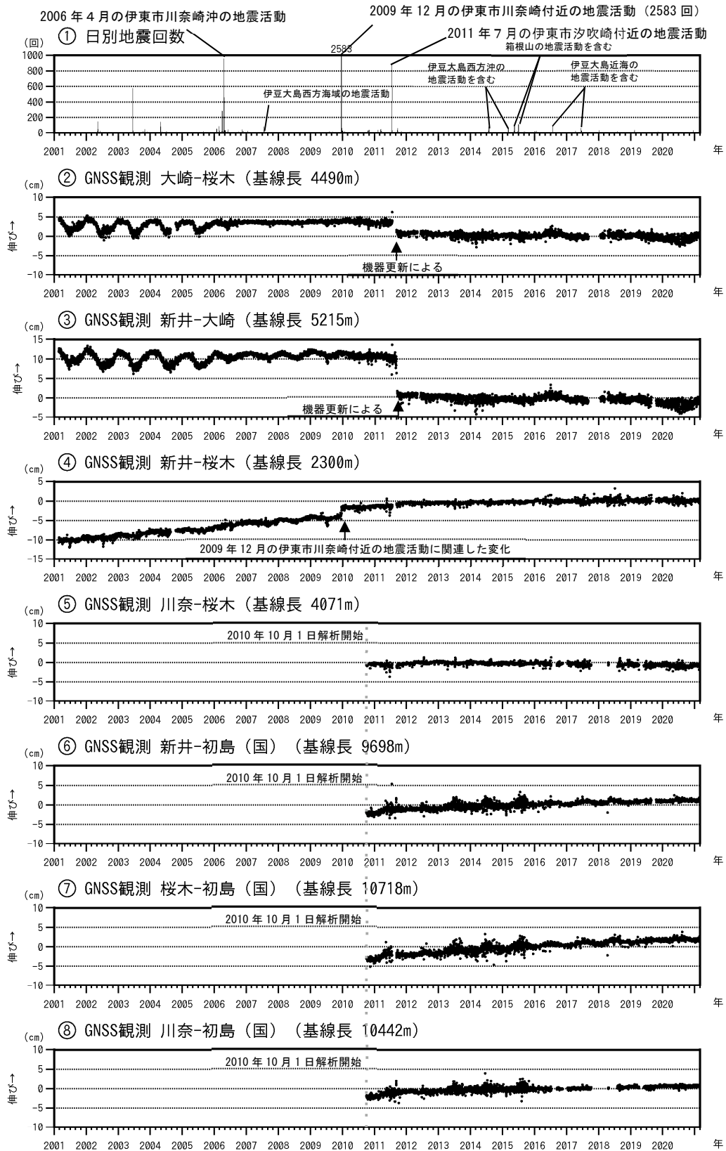
図3 伊豆東部火山群 火山活動経過図（2001年1月1日～2021年2月28日）
