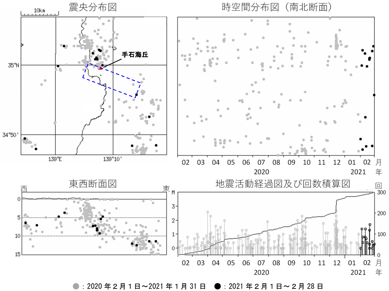
図2 伊豆東部火山群 広域地震観測網による震源分布図（2020年2月1日～2021年2月28日） □の領域は群発地震活動の発生する可能性がある範囲（火口が発生する可能性のある範囲）を示しています。 https://www.data.jma.go.jp/svd/vois/data/tokyo/STOCK/level/PDF/level_316.pdf 広域地震観測網により震源決定したもので、深さは全て海面以下として決定しています。 M（マグニチュード）は地震の規模を表し、M0.0以上を表示しています。 図中の震源要素は一部暫定値が含まれており、後日変更することがあります。 この図では、関係機関の地震波形を一元的に処理し、地震観測点の標高を考慮する等した新手法で得られた震源を用いています（ただし、2020年8月以前の地震については火山活動評価のための参考震源です）。 2021年3月8日現在、2020年4月18日から10月23日まで、及び2021年1月9日以降の地震について、暫定的に震源精査の基準を変更しているため、その前後の期間と比較して微小な地震での震源決定数の変化（増減）が見られます。
