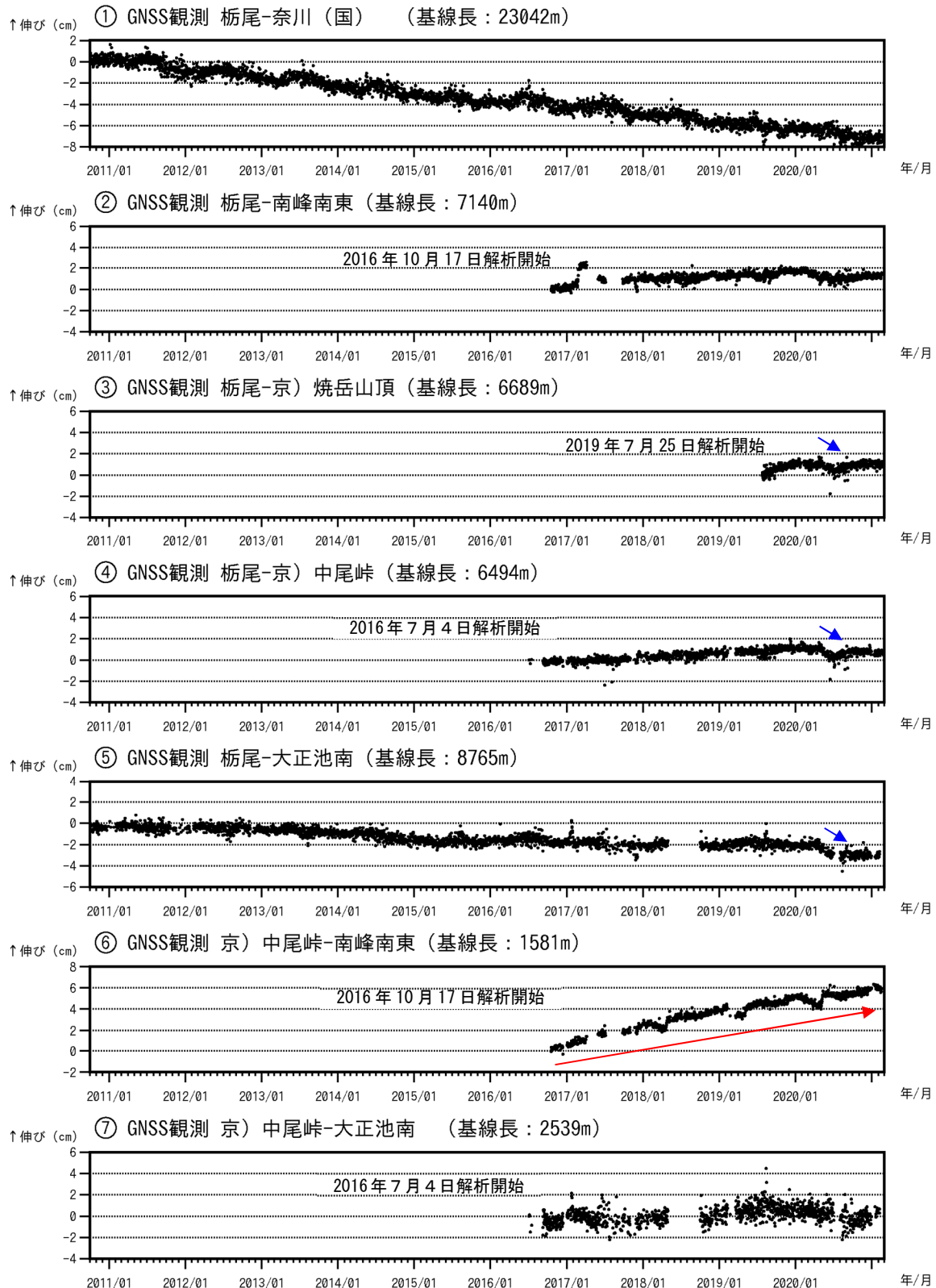
図7 焼岳 GNSS 連続観測による基線長変化 (2010年10月1日～2021年2月28日)
