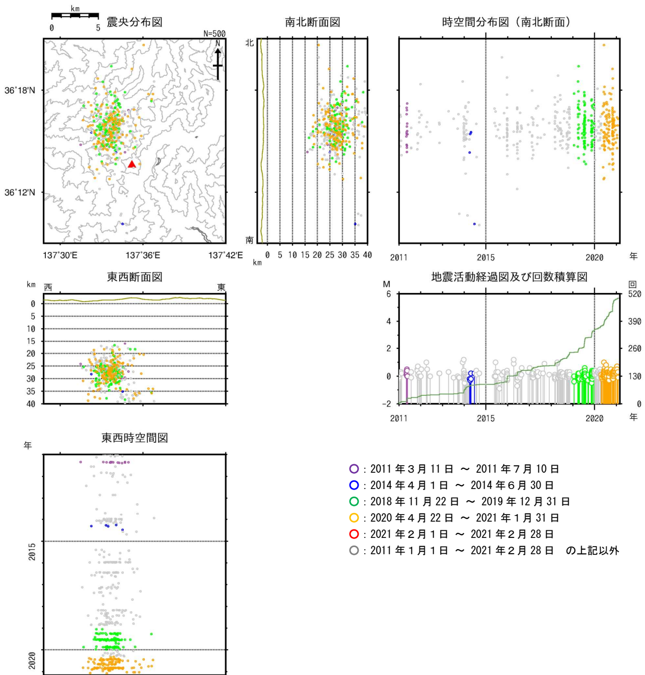
図3 焼岳 広域地震観測網による深部低周波地震の震源分布図（2011年1月1日～2021年2月28日） 広域地震観測網により震源決定したもので、深さは全て海面以下として決定しています。そのため、山頂付近の浅い地震の震源も海面下に決定されています。 M（マグニチュード）は地震の規模を表します。 図中の震源要素は一部暫定値が含まれており、後日変更することがあります。 2021年3月8日現在、2020年4月18日から10月23日まで、及び2021年1月9日以降の地震について、暫定的に震源精査の基準を変更しているため、その前後の期間と比較して微小な地震での震源決定数の変化（増減）が見られます。 ・焼岳の北西側の深い所を震源とする低周波地震は、今期間、観測されませんでした。 ・過去には、図2に示したような焼岳周辺の地震活動の活発化がみられた期間付近で、深部低周波地震が増加したことがあります。
