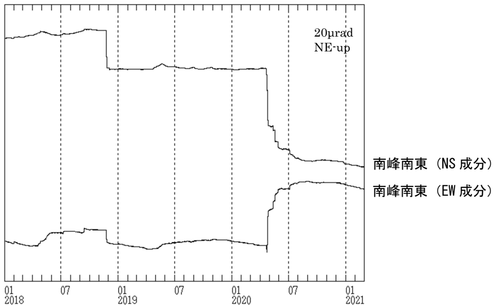
図9 焼岳 南峰南東観測点における傾斜データ（2018年1月1日～2021年2月28日）
