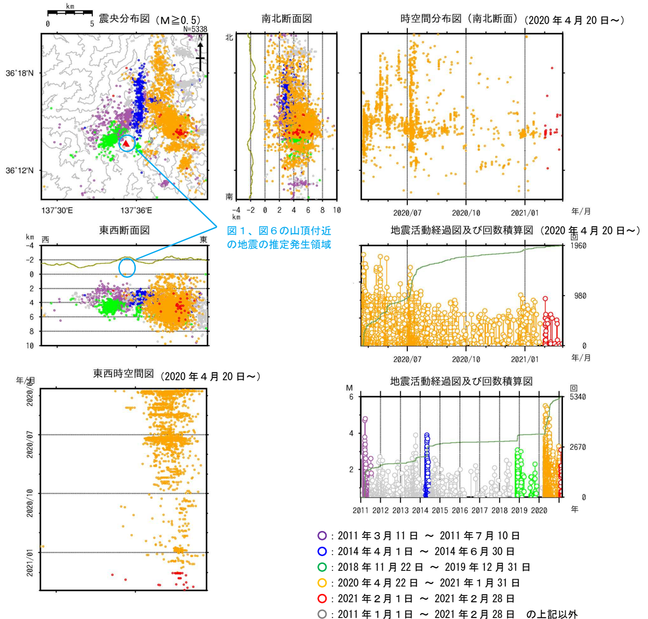
図2 焼岳 広域地震観測網による山体及び周辺の地震活動(2011年1月1日～2021年2月28日)
