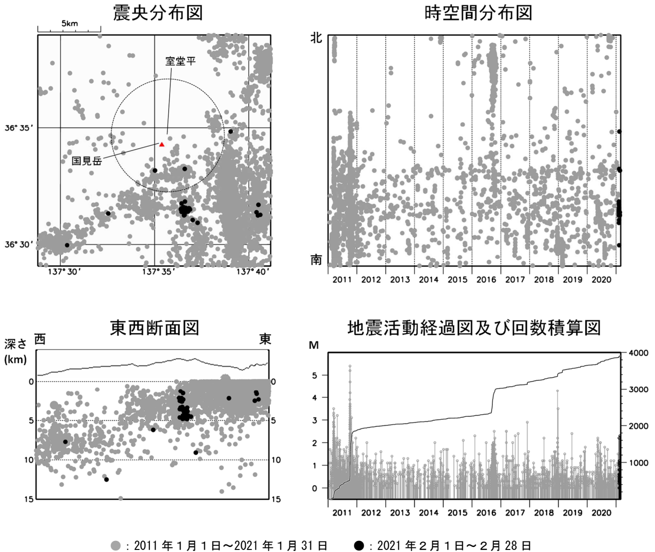
図2 弥陀ヶ原 広域地震観測網による山体・周辺の地震活動（2011 年 1 月 1 日～2021 年 2 月 28 日） 震央分布図中の円は弥陀ヶ原の計数対象地震（室堂平で S-P 時間 1 秒以内）のおよその範囲を示しています。 広域地震観測網により震源決定したもので、深さは全て海面以下として決定しています。 図中の震源要素は一部暫定値が含まれており、後日変更することがあります。 この図では、関係機関の地震波形を一元的に処理し、地震観測点の標高を考慮する等した新手法で得られた震源を用いています（ただし、2020 年 8 月以前の地震については火山活動評価のための参考震源です）。 2021 年 3 月 8 日現在、2020 年 4 月 18 日から 10 月 23 日まで、及び 2021 年 1 月 9 日以降の地震について、暫定的に震源精査の基準を変更しているため、その前後の期間と比較して微小な地震での震源決定数の変化（増減）が見られます。
