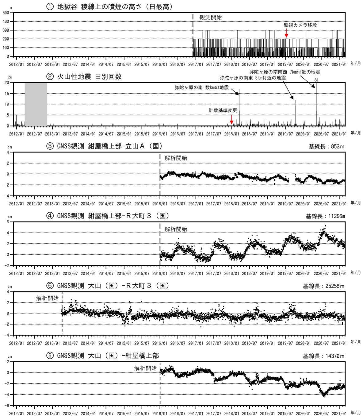
図3 弥陀ヶ原 火山活動経過図（2011年12月1日～2021年2月28日）
