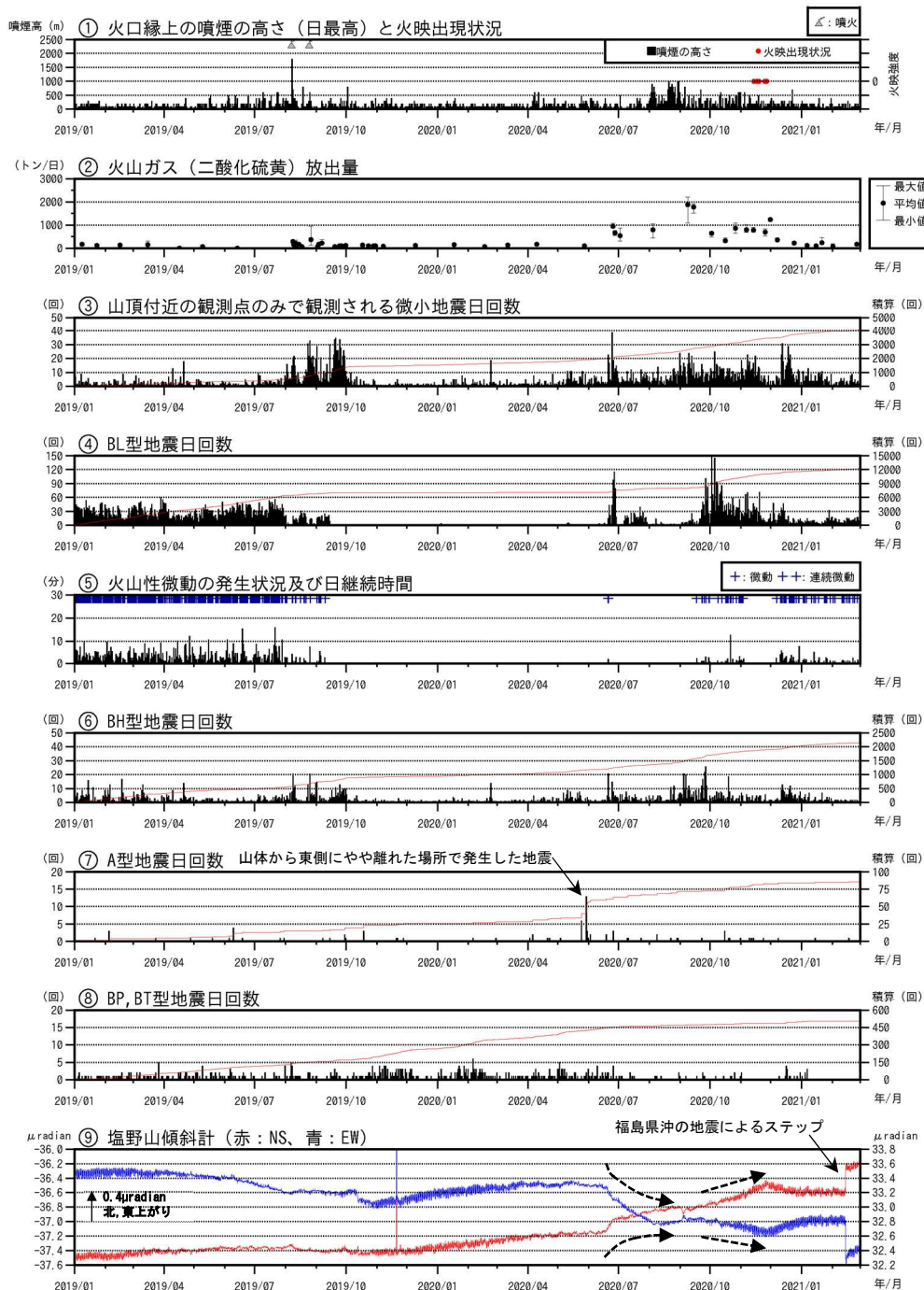
図3 浅間山 火山活動経過図（2019年1月1日～2021年2月28日）
