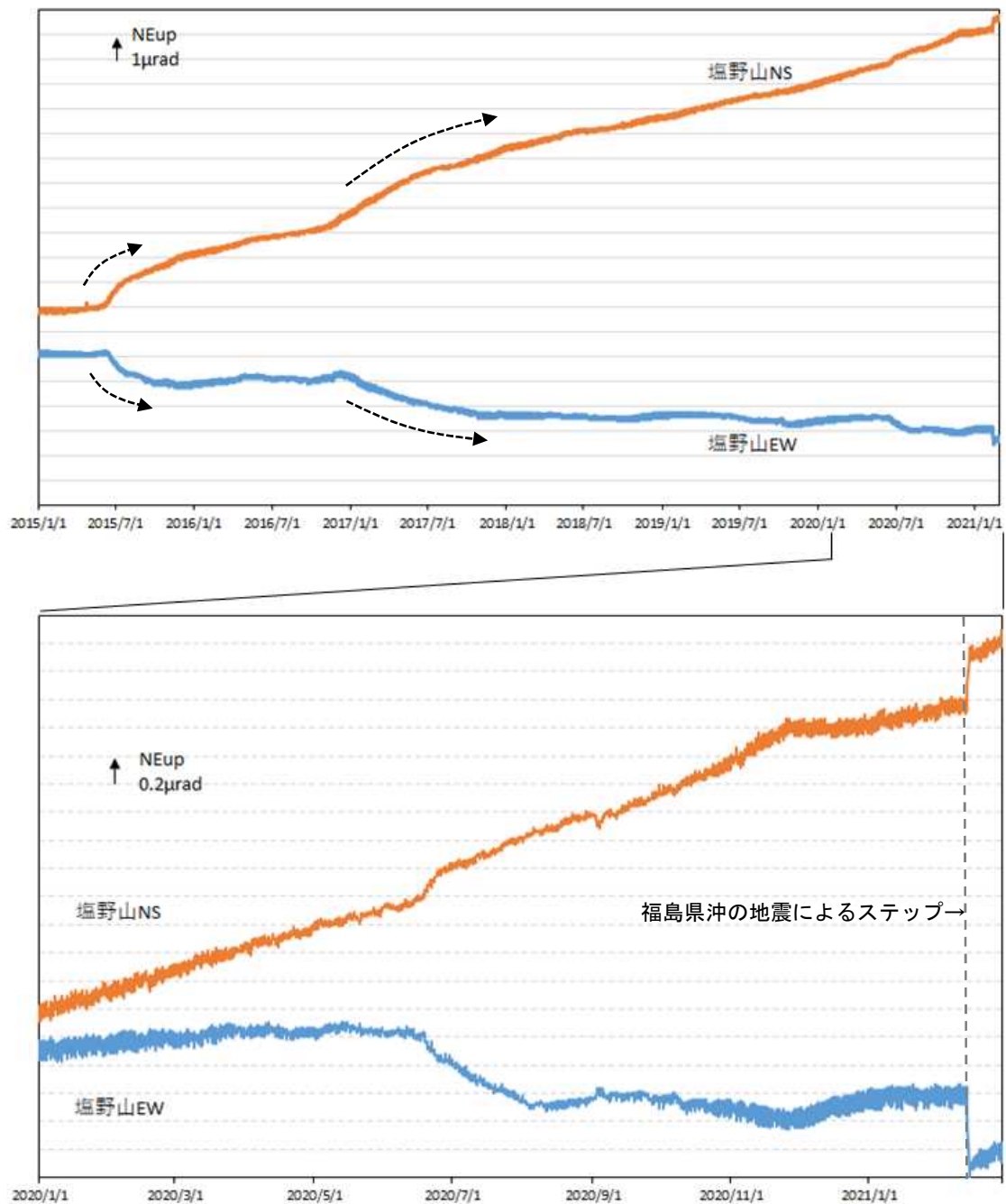
図9 浅間山 塩野山観測点における傾斜データ（2015年1月1日～2021年2月28日） データは時間平均値を使用しており、長期にわたるトレンドを補正しています。 下段は上段に比べて縦軸を拡大しています。
