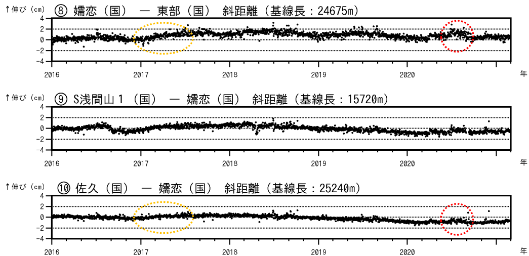
図7-2 浅間山 GNSS 連続観測結果(2016年1月1日~2021年2月28日)
