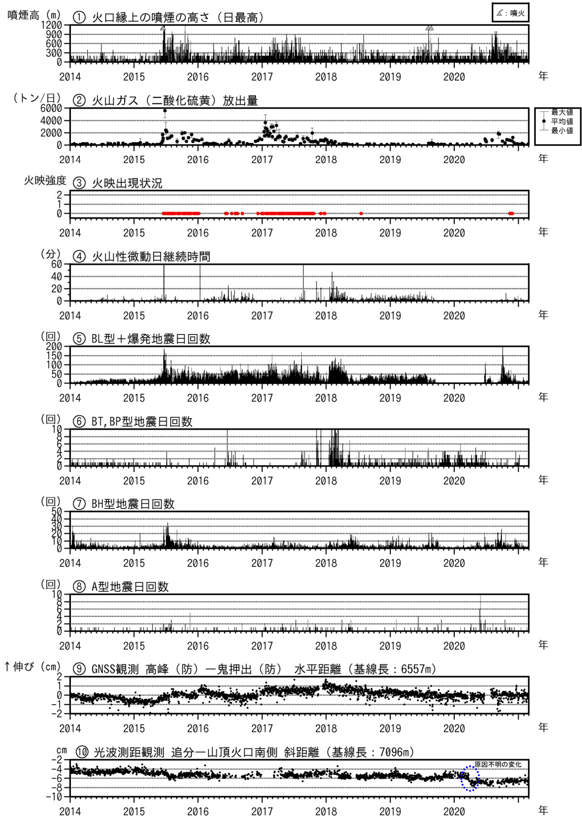
図5 浅間山 最近の火山活動経過図（2014年1月1日～2021年2月28日）
