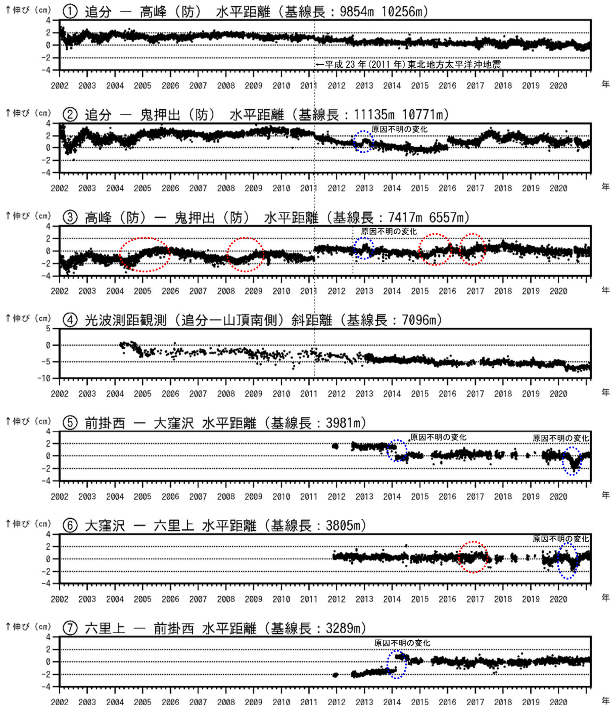
図7-1 浅間山 GNSS連続観測及び光波測距観測の結果(2002年1月1日~2021年2月28日) 2010年10月及び2016年1月に、解析方法を変更しています。
