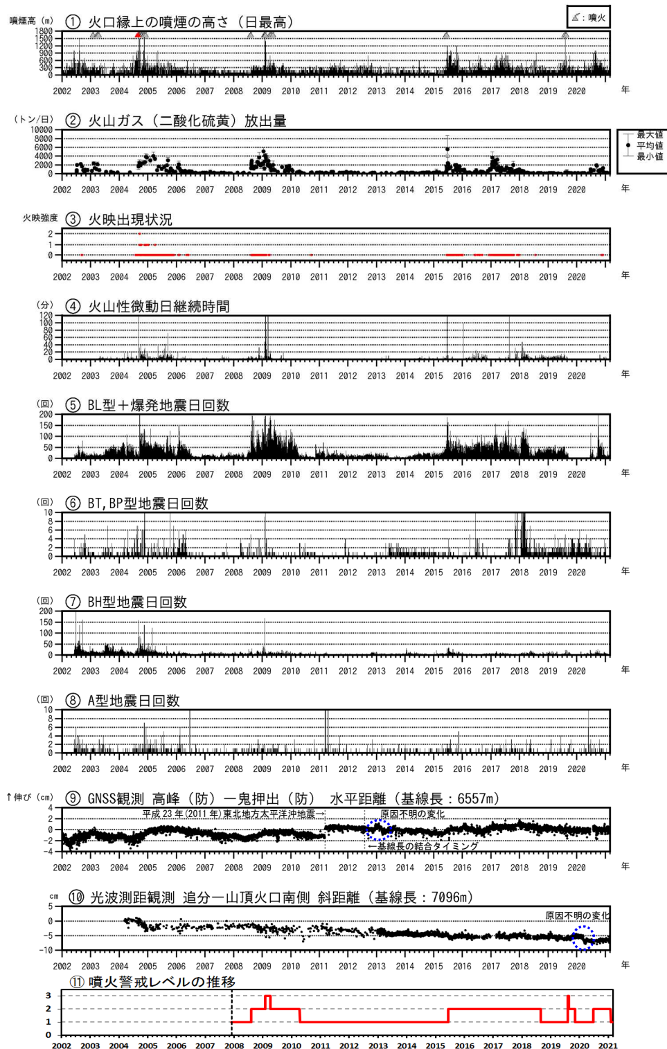
図4 浅間山 火山活動経過図（2002年1月1日～2021年2月28日）
