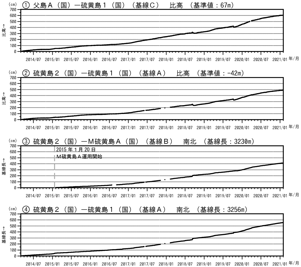
図5 硫黄島 GNSS 連続観測結果 (2014年3月1日~2021年1月31日)
