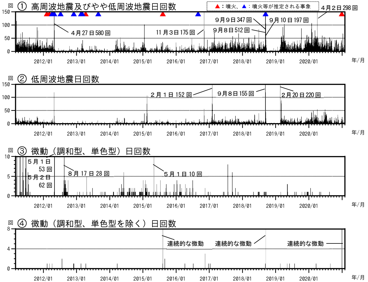
図4 硫黄島 長期火山活動経過図（2011年3月8日～2021年1月31日）
