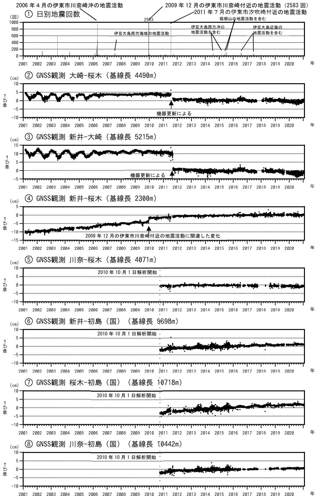
図3 伊豆東部火山群 火山活動経過図（2001年1月1日～2021年1月31日）
