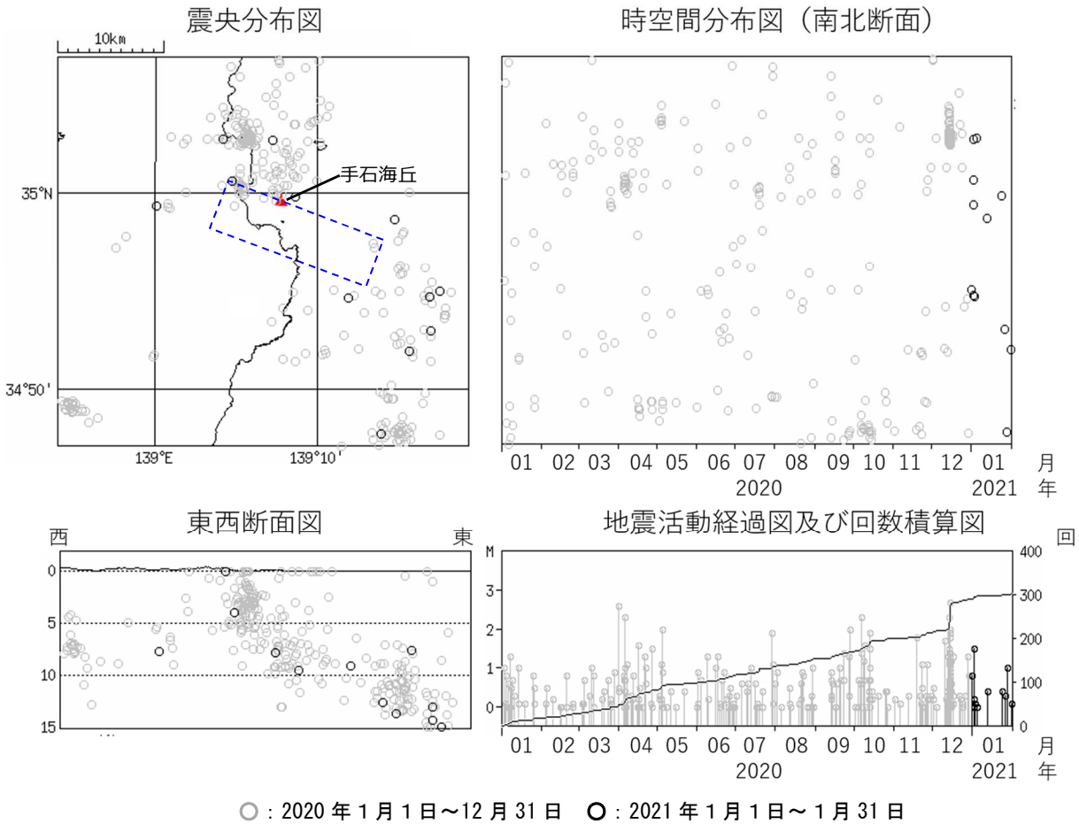
図2 伊豆東部火山群 広域地震観測網による震源分布図（2020年1月1日～2021年1月31日） □の領域は群発地震活動の発生する可能性がある範囲（火口が発生する可能性のある範囲）を示しています。 https://www.data.jma.go.jp/svd/vois/data/tokyo/STOCK/level/PDF/level_316.pdf 広域地震観測網により震源決定したもので、深さは全て海面以下として決定しています。 M（マグニチュード）は地震の規模を表し、M0.0以上を表示しています。 図中の震源要素は一部暫定値が含まれており、後日変更することがあります。 この図では、関係機関の地震波形を一元的に処理し、地震観測点の標高を考慮する等した新手法で得られた震源を用いています（ただし、2020年8月以前の地震については火山活動評価のための参考震源です）。 2021年2月8日現在、2020年4月18日から10月23日まで、及び2021年1月9日以降の地震について、暫定的に震源精査の基準を変更しているため、その前後の期間と比較して微小な地震での震源決定数の変化（増減）が見られます。
