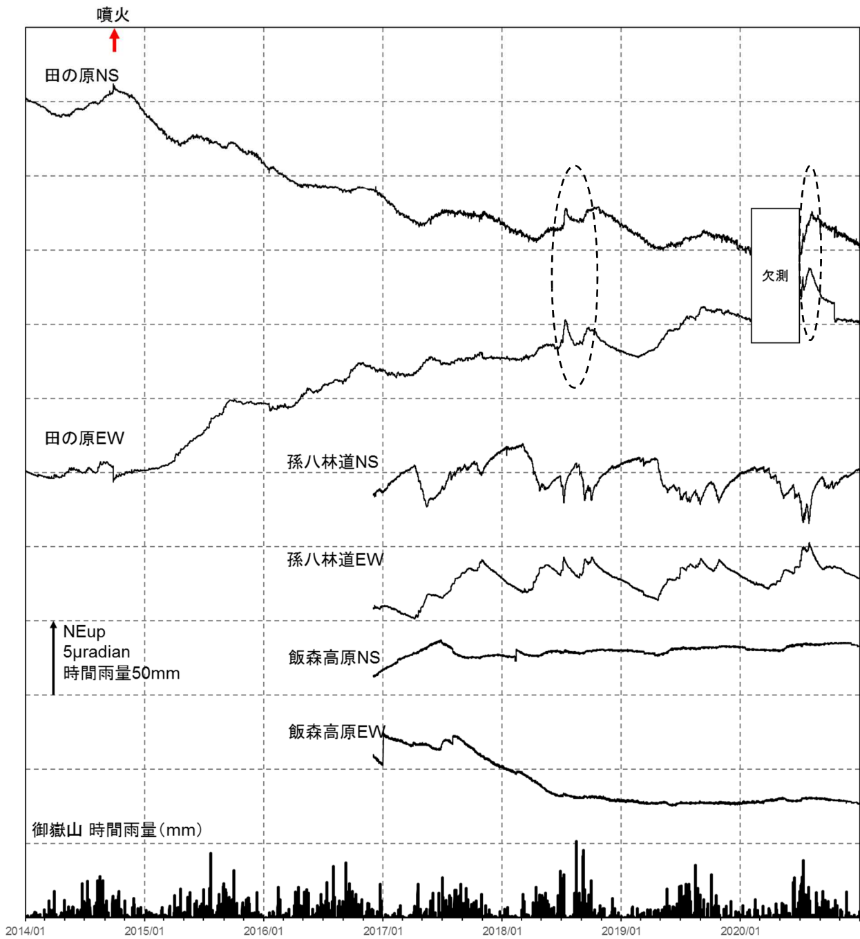
図7 御嶽山 傾斜変動（2014年1月1日～2020年12月31日）
