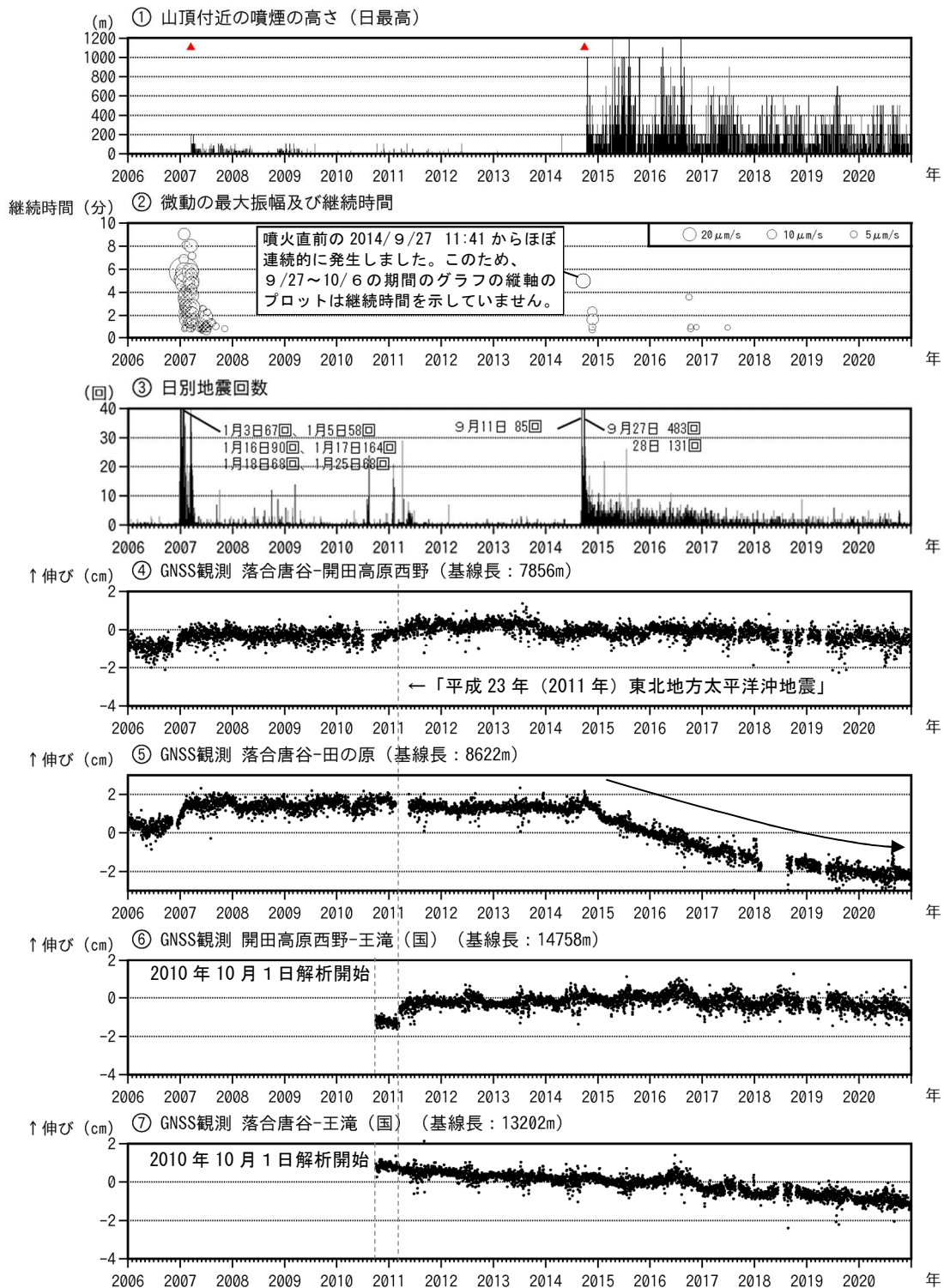
図5 御嶽山 長期間の火山活動経過図（2006年1月1日～2020年12月31日）
