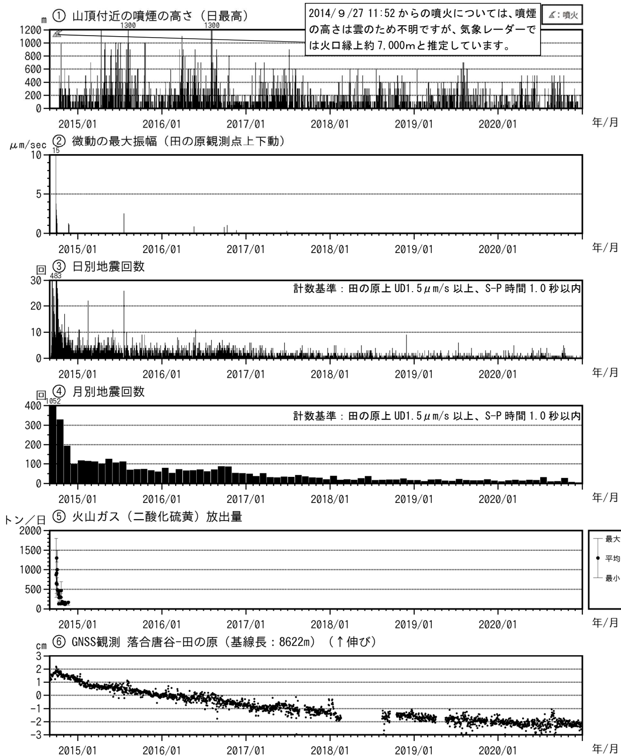
図4 御嶽山 最近の火山活動経過図（2014年9月1日～2020年12月31日）
