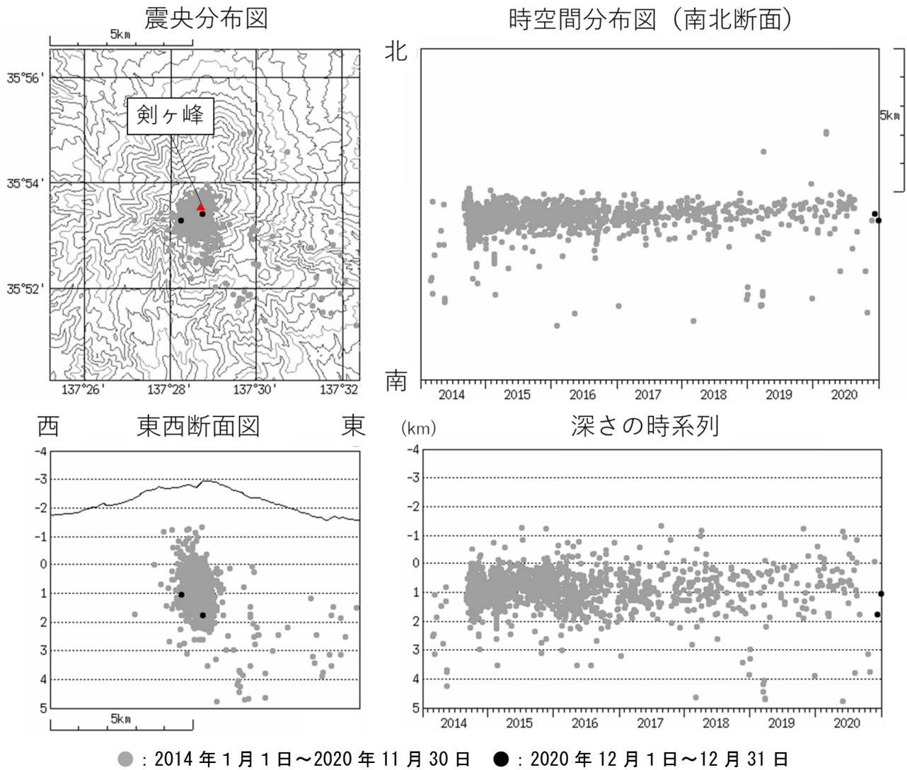
図3 御嶽山 震源分布図（2014年1月1日～2020年12月31日）
