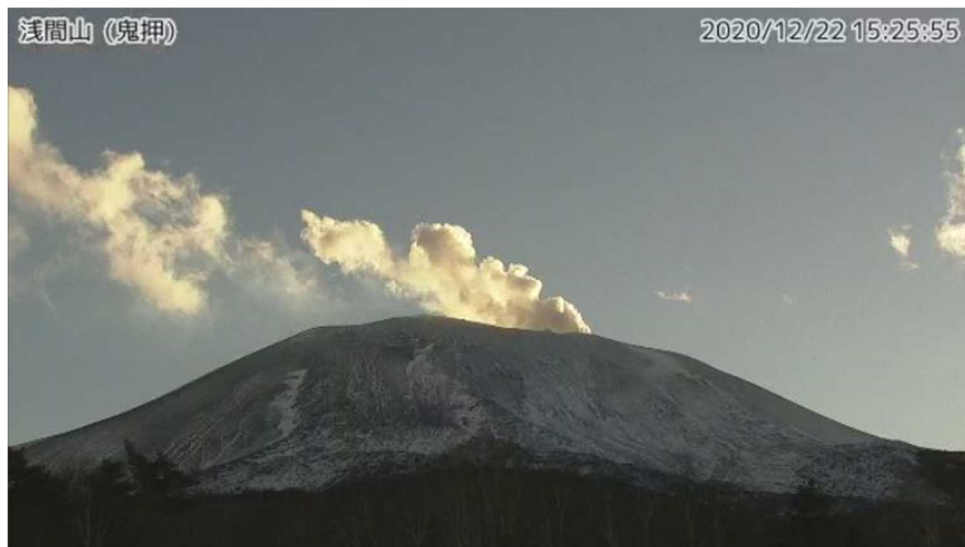
図2 浅間山 山頂部の噴煙の状況 鬼押監視カメラ（12月22日）
