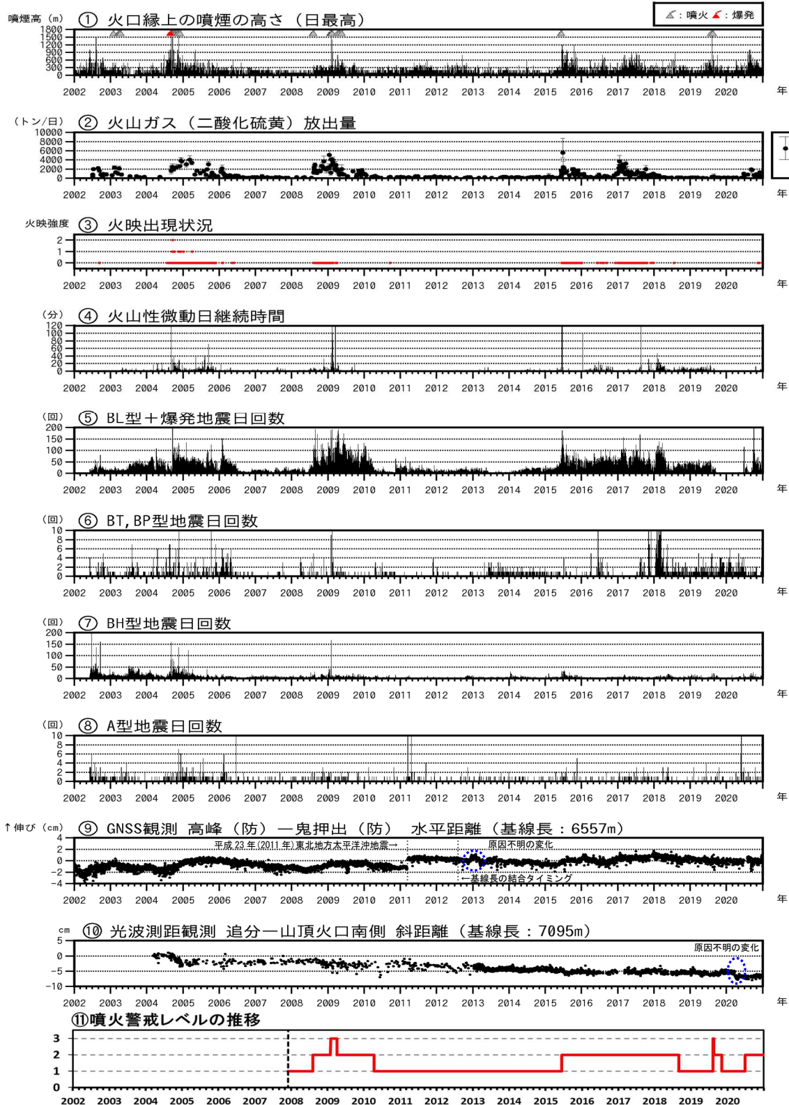
図4 浅間山 火山活動経過図（2002年1月1日～2020年12月31日）
