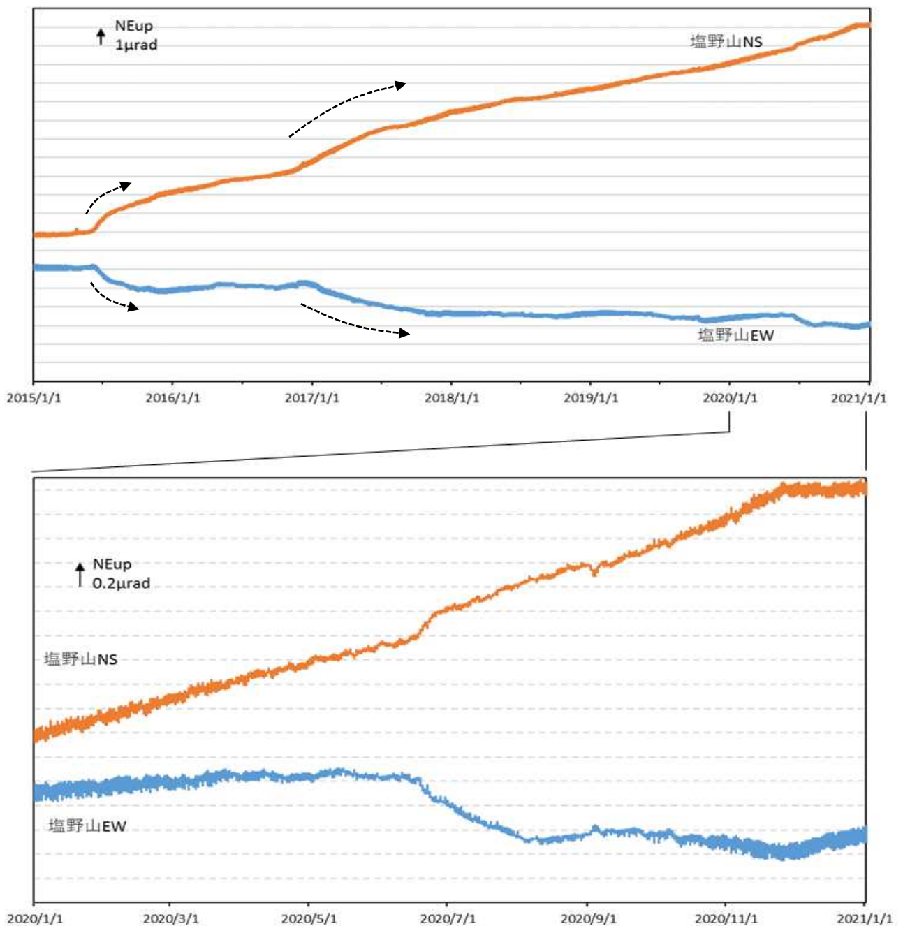
図9 浅間山 塩野山観測点における傾斜データ（2015年1月1日～2020年12月31日）
