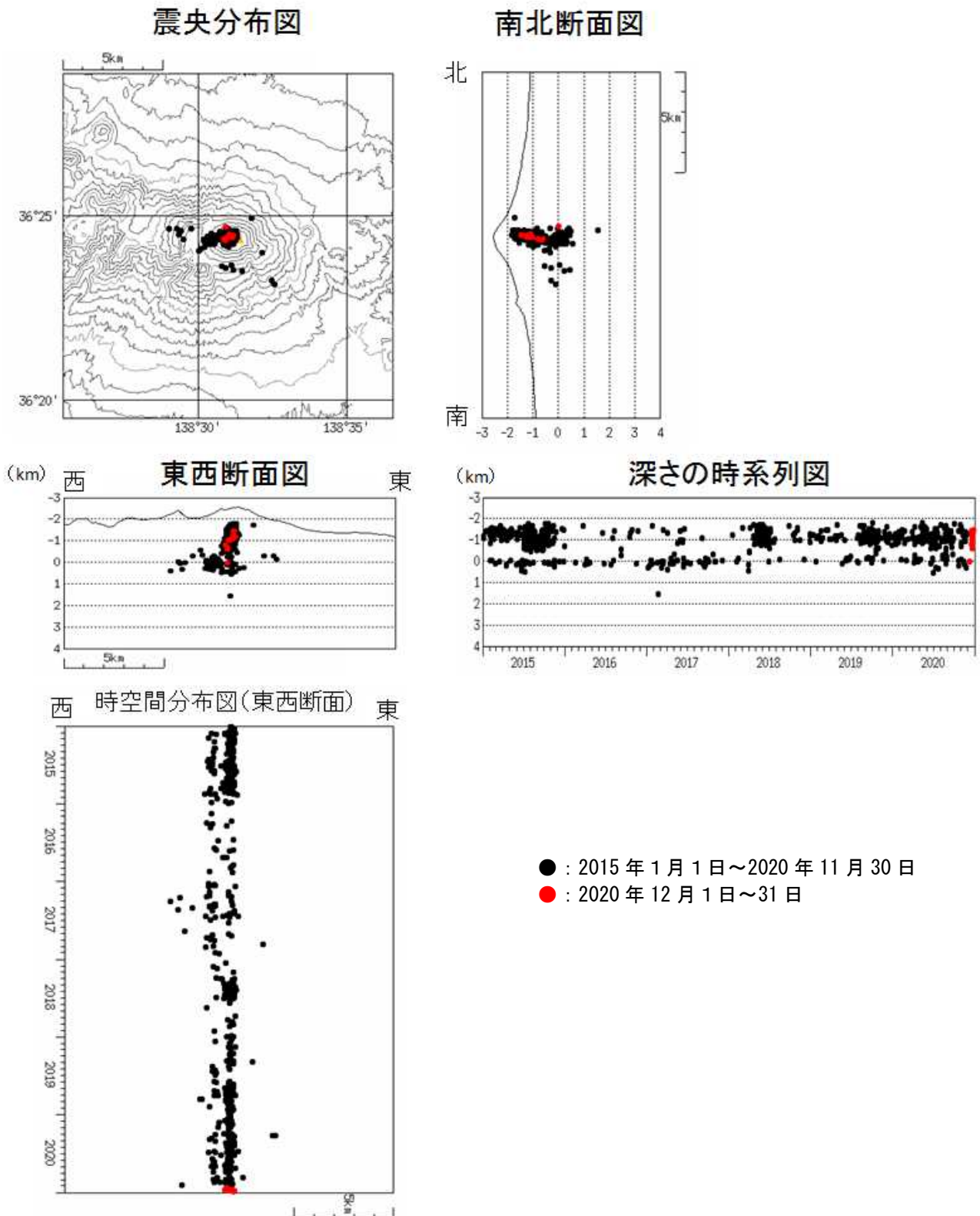
図6 浅間山 震源分布図（2015年1月1日～2020年12月31日）
