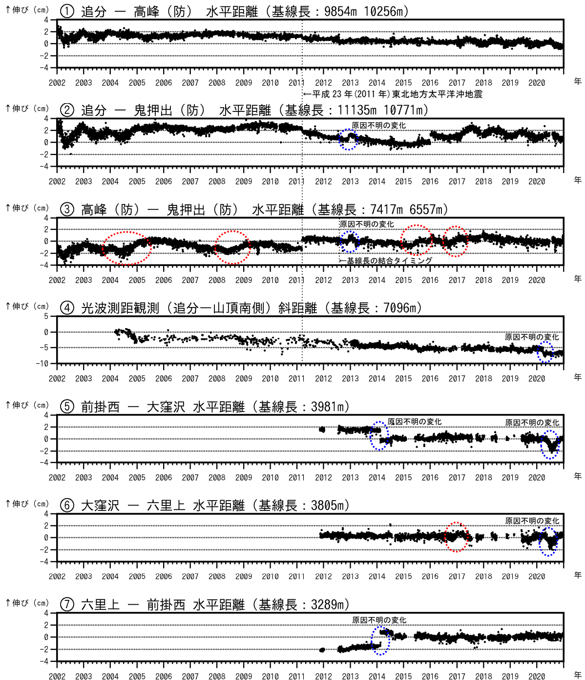
図7-1 浅間山 GNSS 連続観測及び光波測距観測の結果(2002年1月1日～2020年12月31日) 2010年10月及び2016年1月に、解析方法を変更しています。
