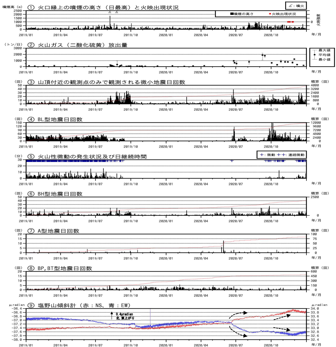
図3 浅間山 火山活動経過図（2019年1月1日～2020年12月31日）
