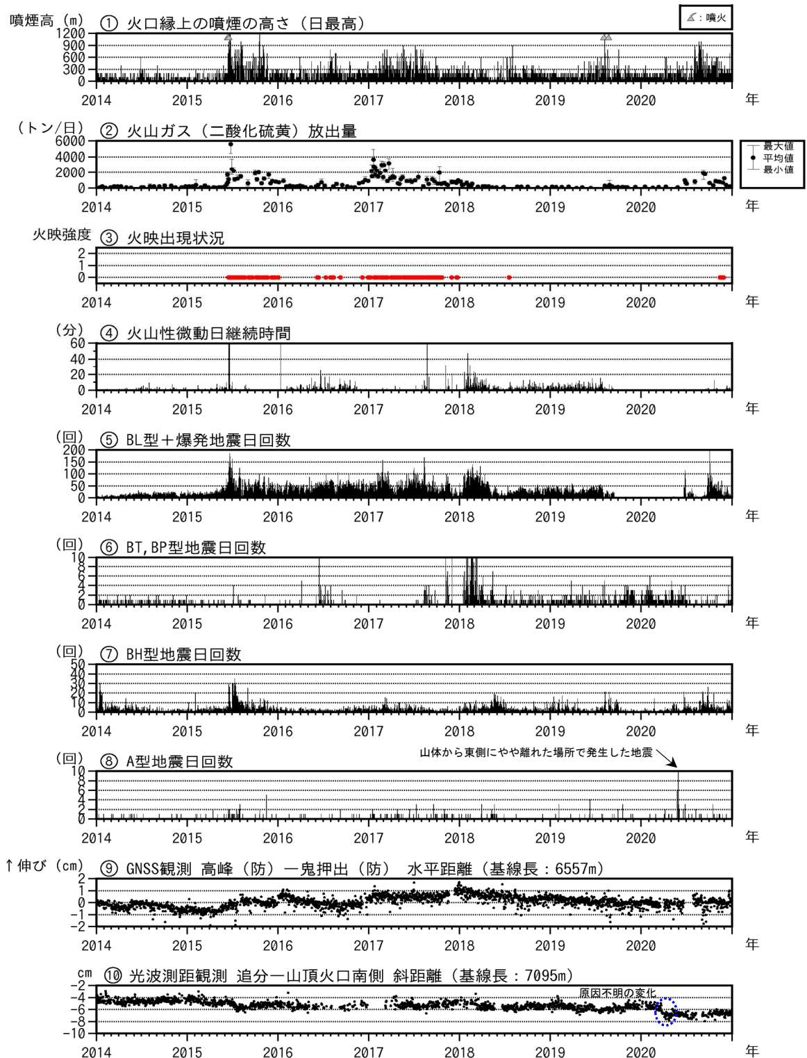
図5 浅間山 最近の火山活動経過図 (2014年1月1日～2020年12月31日)
