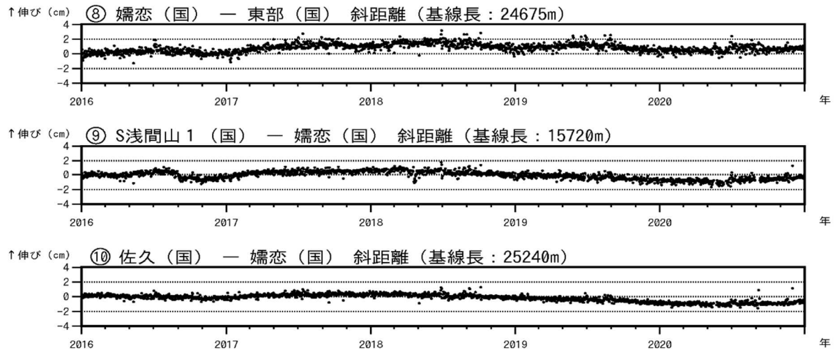
図7-2 浅間山 GNSS 連続観測結果(2016年1月1日～2020年12月31日)
