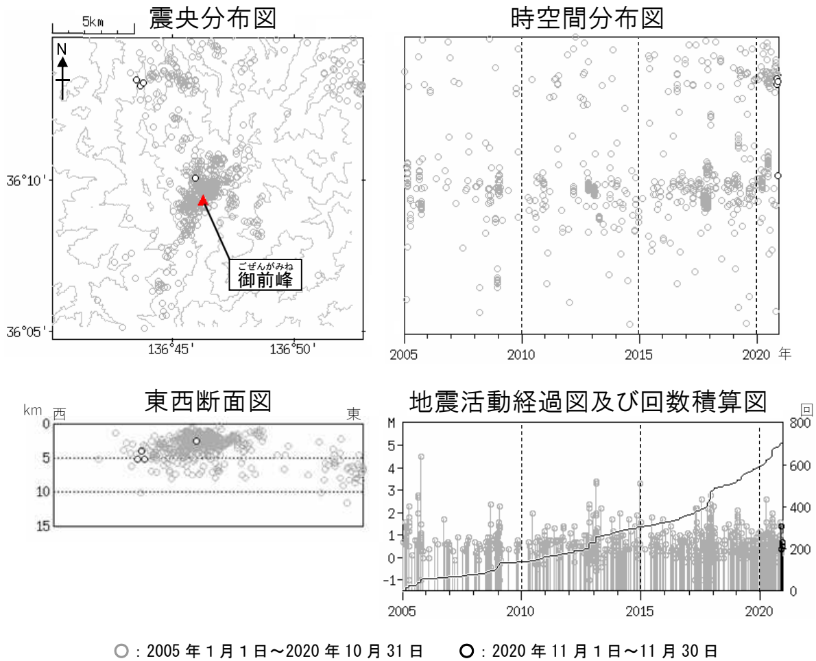
図4 白山 広域地震観測網による山体・周辺の地震活動（2005年1月1日～2020年11月30日）
