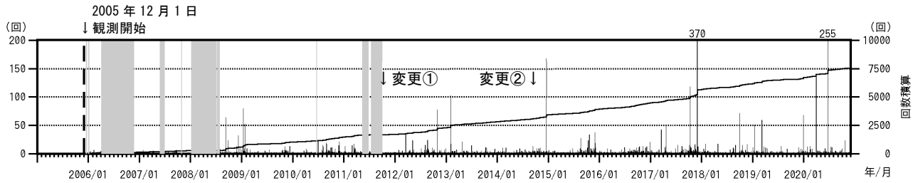
図3 白山 日別地震回数と積算回数（2005年12月1日～2020年11月30日）
