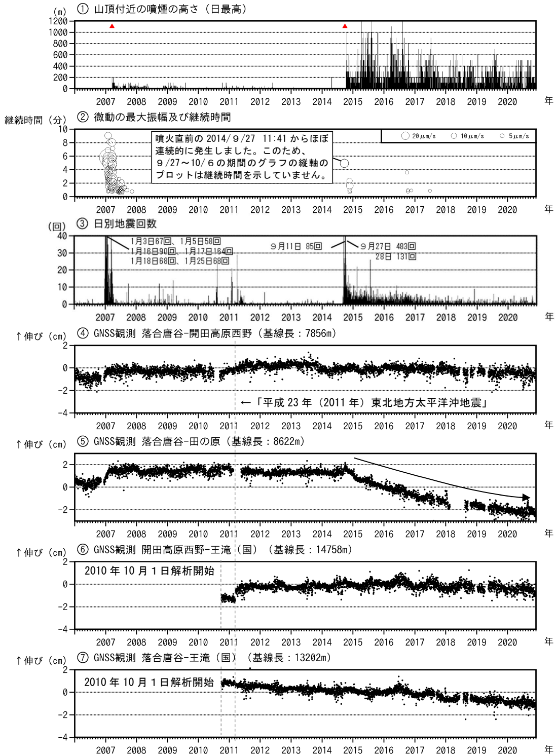
図5 御嶽山 長期間の火山活動経過図（2006年1月1日～2020年11月30日） ①監視カメラによる噴煙の高さ 噴煙の高さは日最大値。赤三角シンボルは噴火発生を示します。 ②火山性微動の最大振幅は田の原上観測点の上下振幅です（火山性微動の発生した2015年7月20日、2016年5月19日は欠測です）。 ④～⑦GNSS連続観測による基線長変化。（国）：国土地理院 2010年10月及び2016年1月以降のデータについては、解析方法を変更しています。空白部分は欠測を示します。 ⑤の基線では、2014年10月以降山体の収縮によると考えられる縮みの傾向が続いています。 ⑥には「平成23年（2011年）東北地方太平洋沖地震」に伴うステップ状の変化がみられます。 図中④～⑦は図6のGNSS基線④～⑦に対応します。
