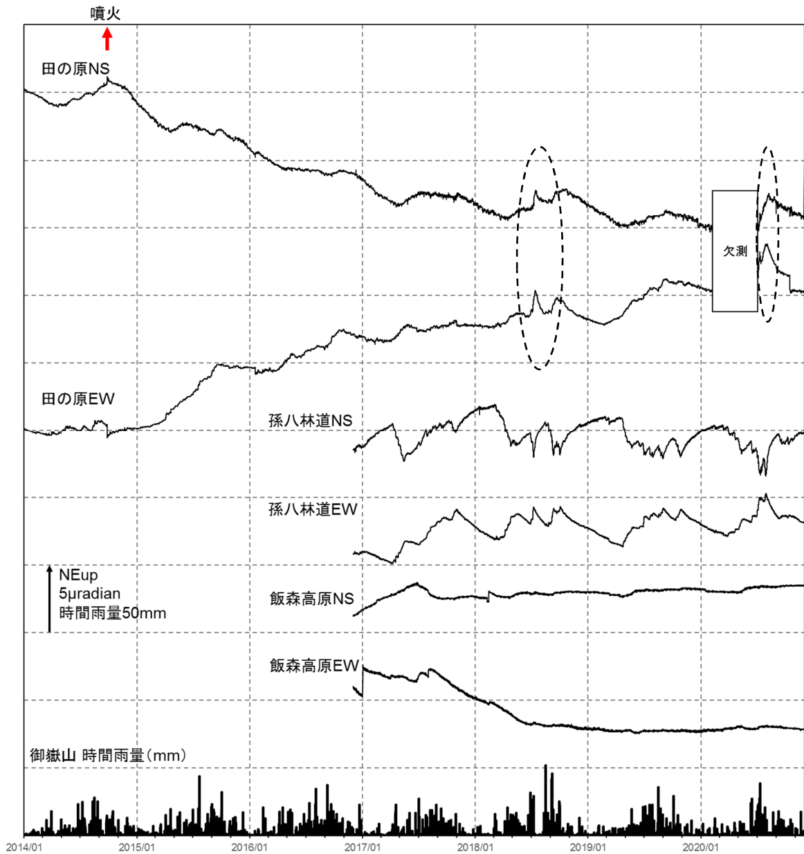
図7 御嶽山 傾斜変動（2014年1月1日～2020年11月30日）
