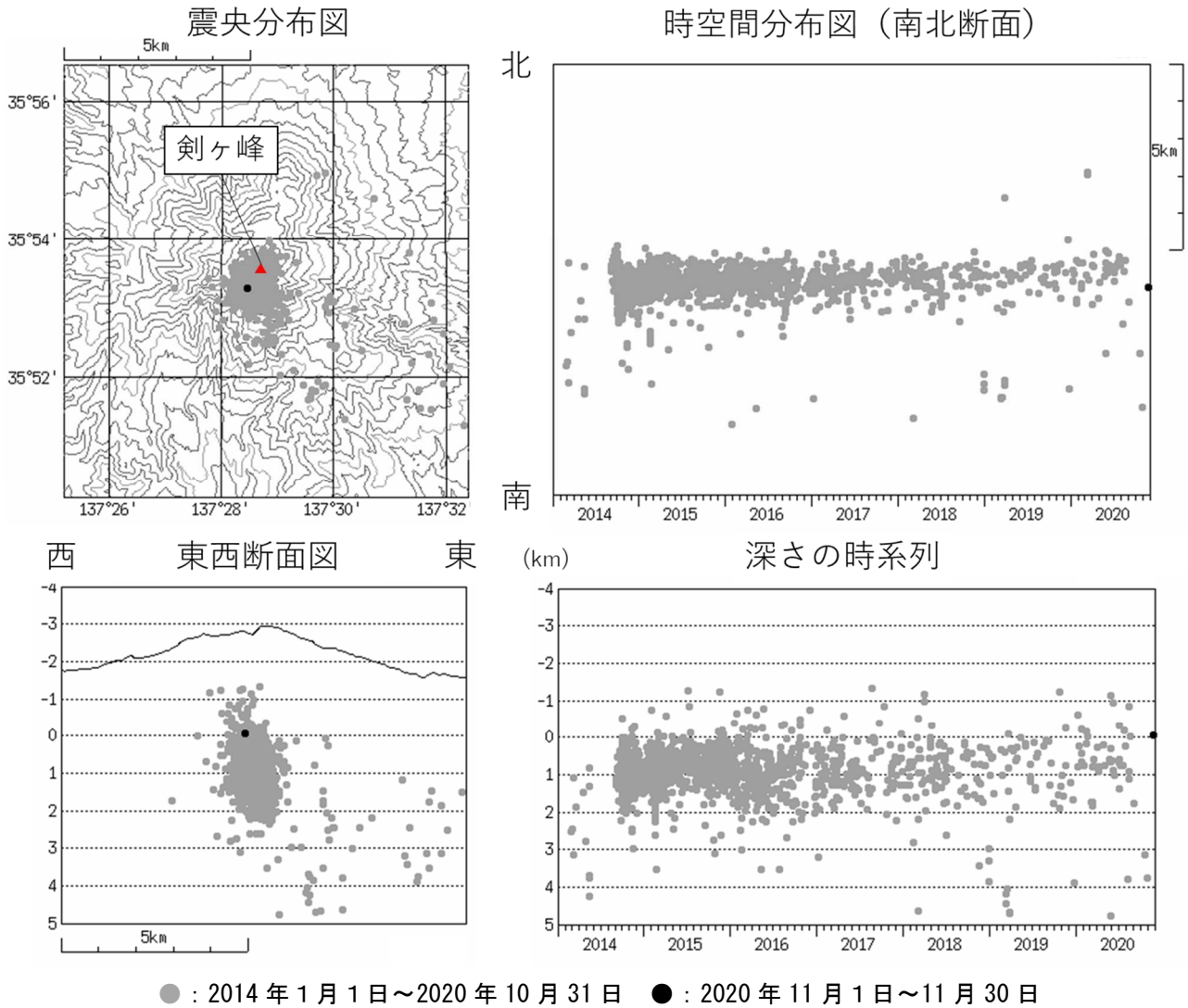
図3 御嶽山 震源分布図（2014年1月1日～2020年11月30日）
