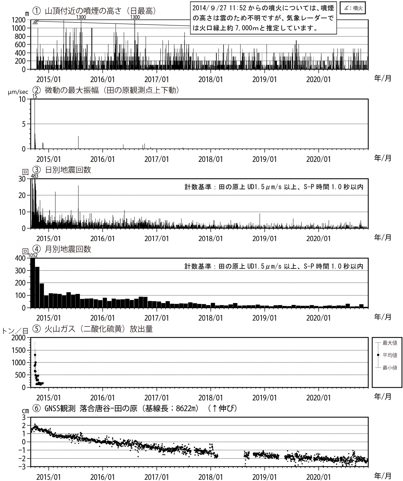
図4 御嶽山 最近の火山活動経過図（2014年9月1日～2020年11月30日）
