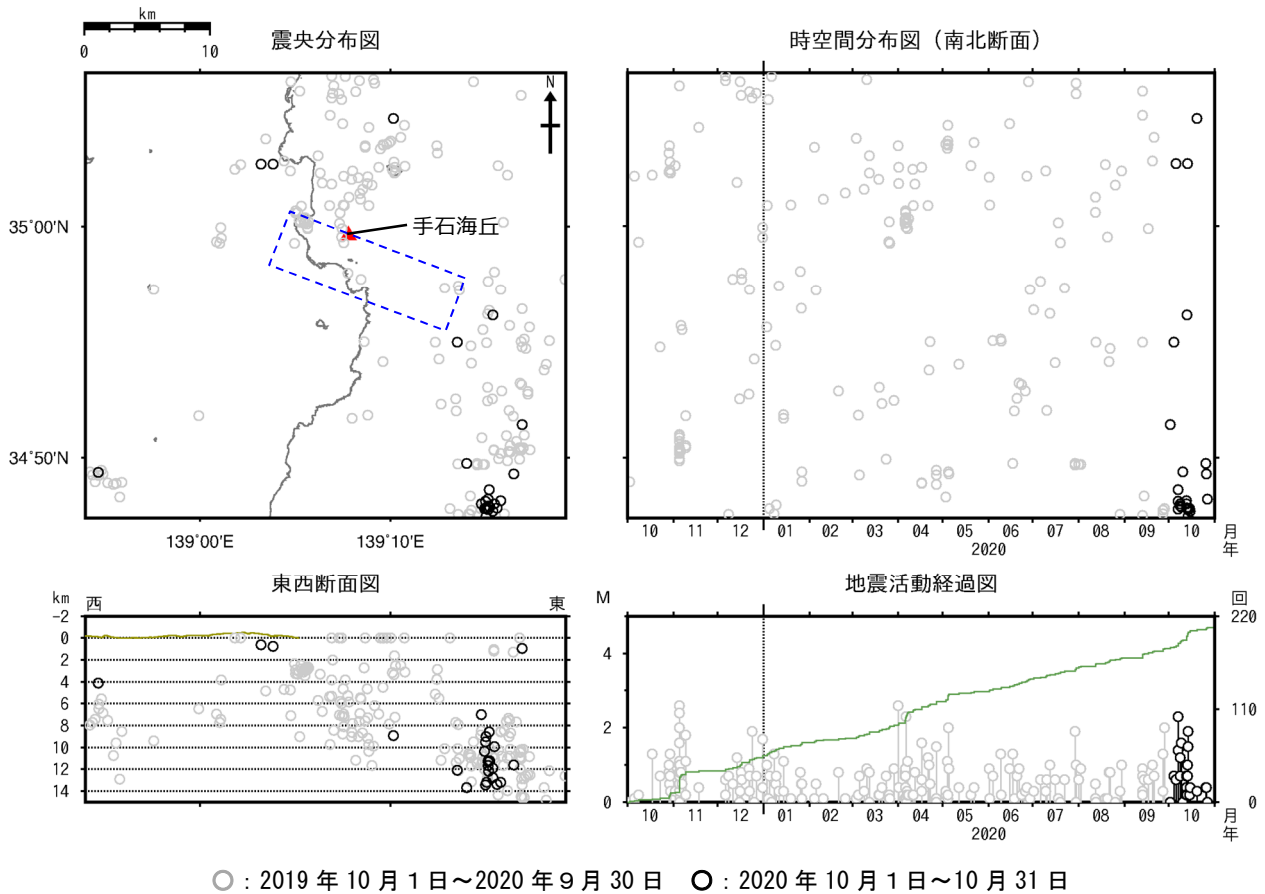
図2 伊豆東部火山群 広域地震観測網による震源分布図（2019年10月1日～2020年10月31日） □の領域は群発地震活動の発生する可能性がある範囲（火口が発生する可能性のある範囲）を示しています。 https://www.data.jma.go.jp/svd/vois/data/tokyo/STOCK/level/PDF/level_316.pdf 広域地震観測網により震源決定したもので、深さは全て海面以下として決定しています。 M（マグニチュード）は地震の規模を表し、M0.0以上を表示しています。 図中の震源要素は一部暫定値が含まれており、後日変更することがあります。 2020年11月10日現在、2020年4月18日から10月23日までの地震について、暫定的に震源精査の基準を変更しているため、その前後の期間と比較して微小な地震での震源決定数の変化（増減）が見られます。 2020年9月以降の震源は、地震観測点の標高を考慮する等した新手法で求められています。
