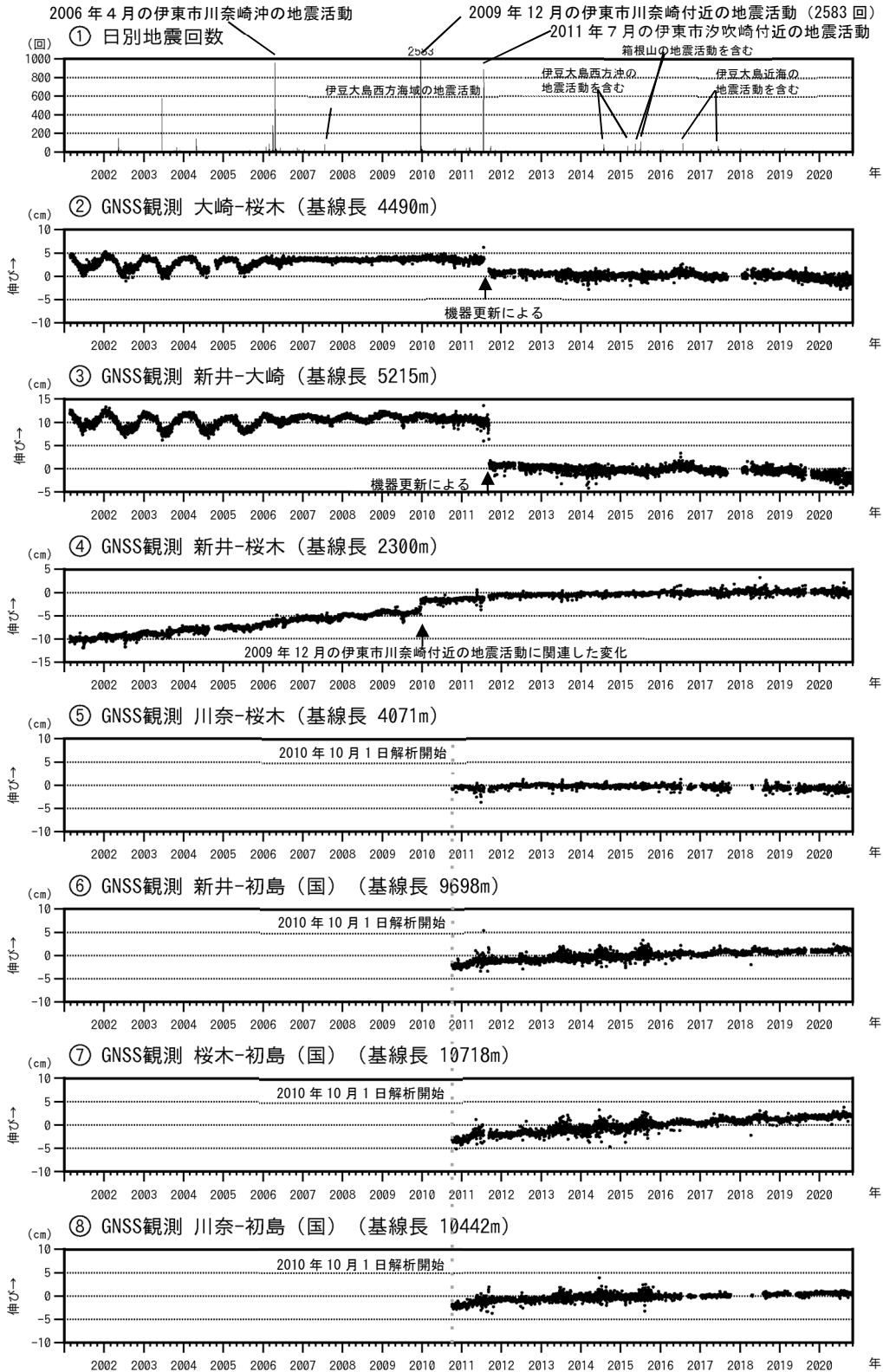
図3 伊豆東部火山群 火山活動経過図 (2001年1月1日～2020年10月31日)
