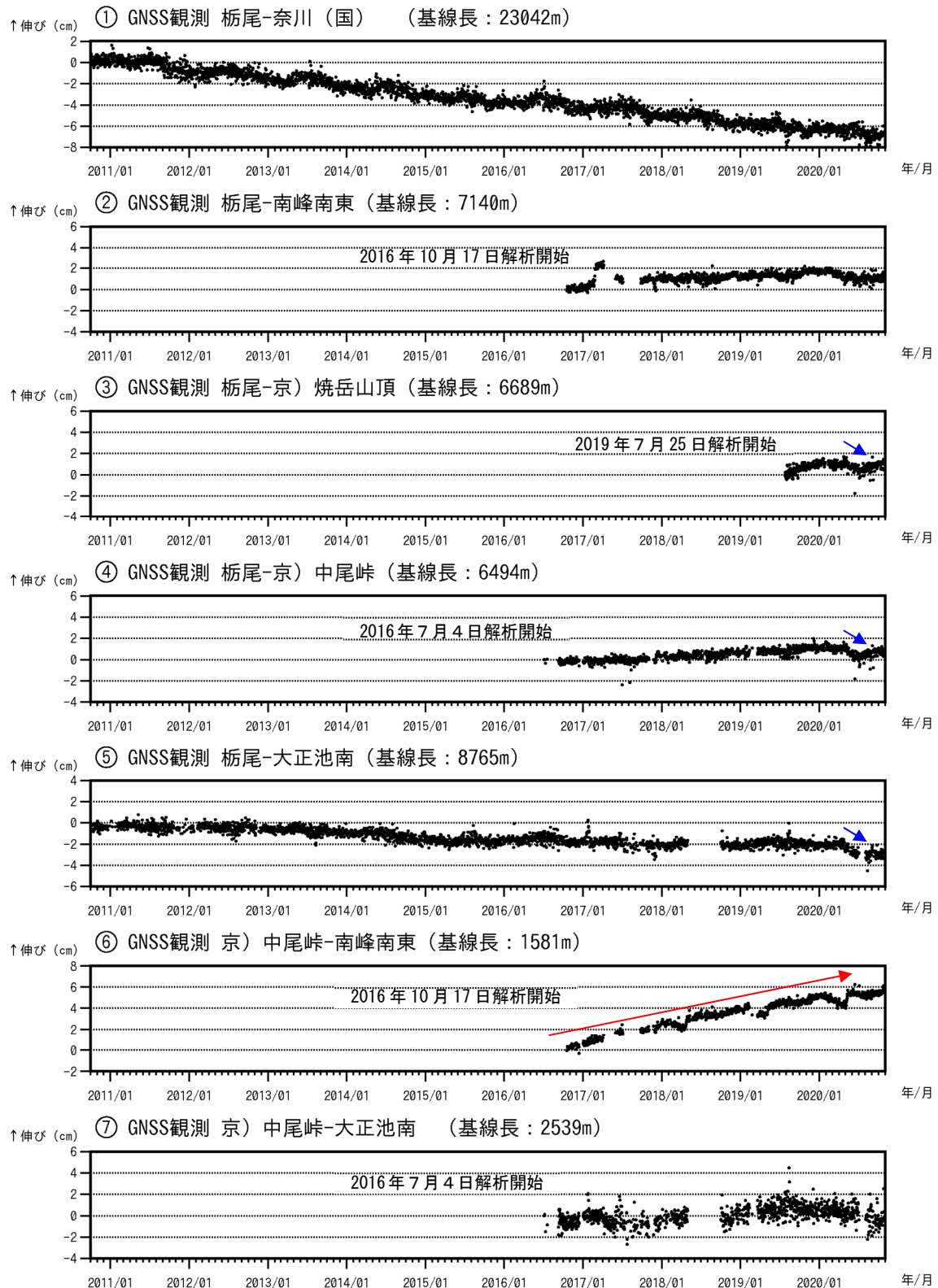
図7 焼岳 GNSS連続観測による基線長変化 (2010年10月1日~2020年10月31日)
