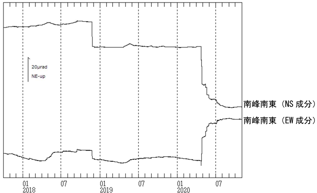
図9 焼岳 南峰南東観測点における傾斜データ（2017年10月1日～2020年10月31日）
