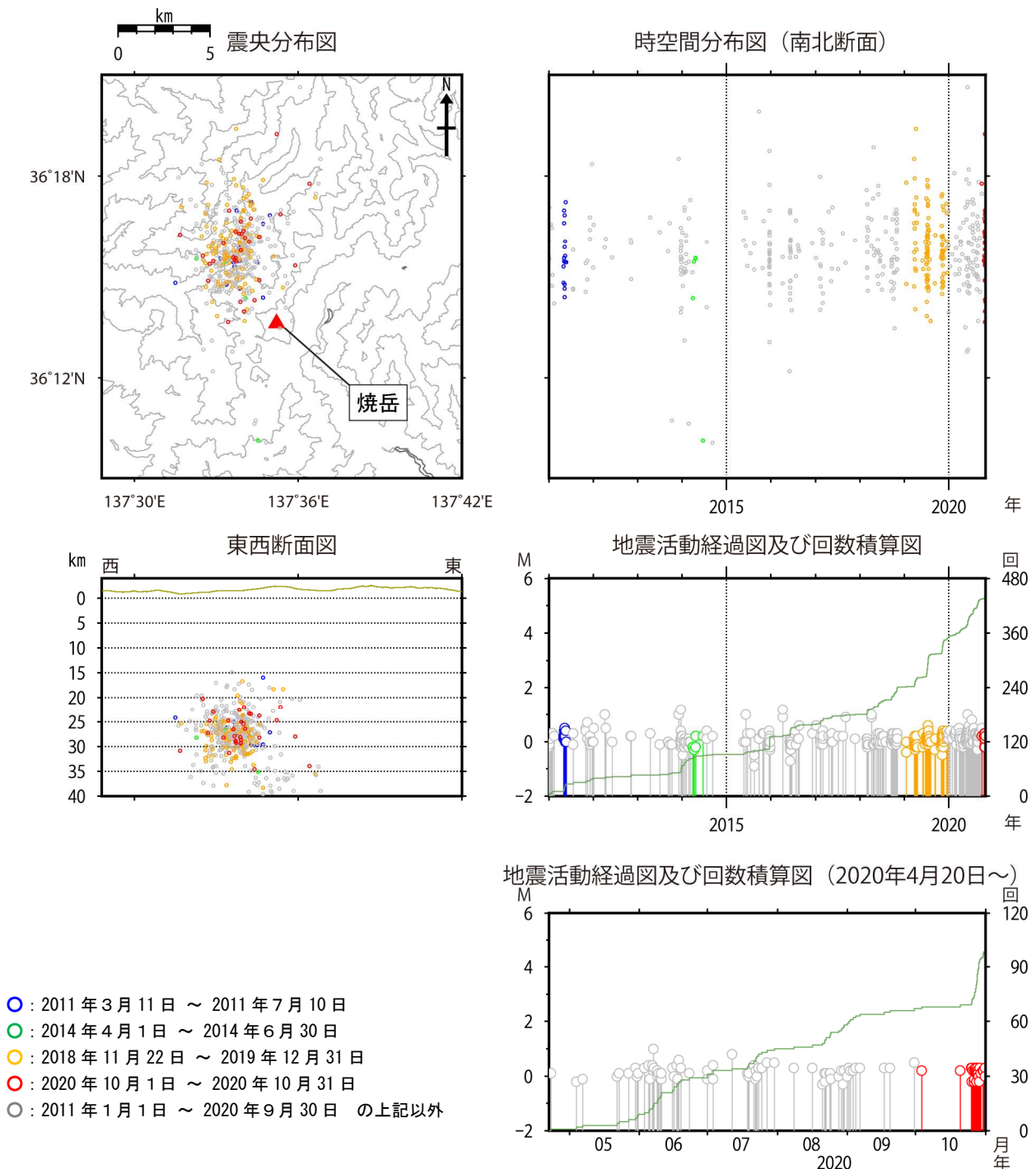
図3 焼岳 深部低周波地震の震源分布図（広域地震観測網による）（2011年1月1日～2020年10月31日）
