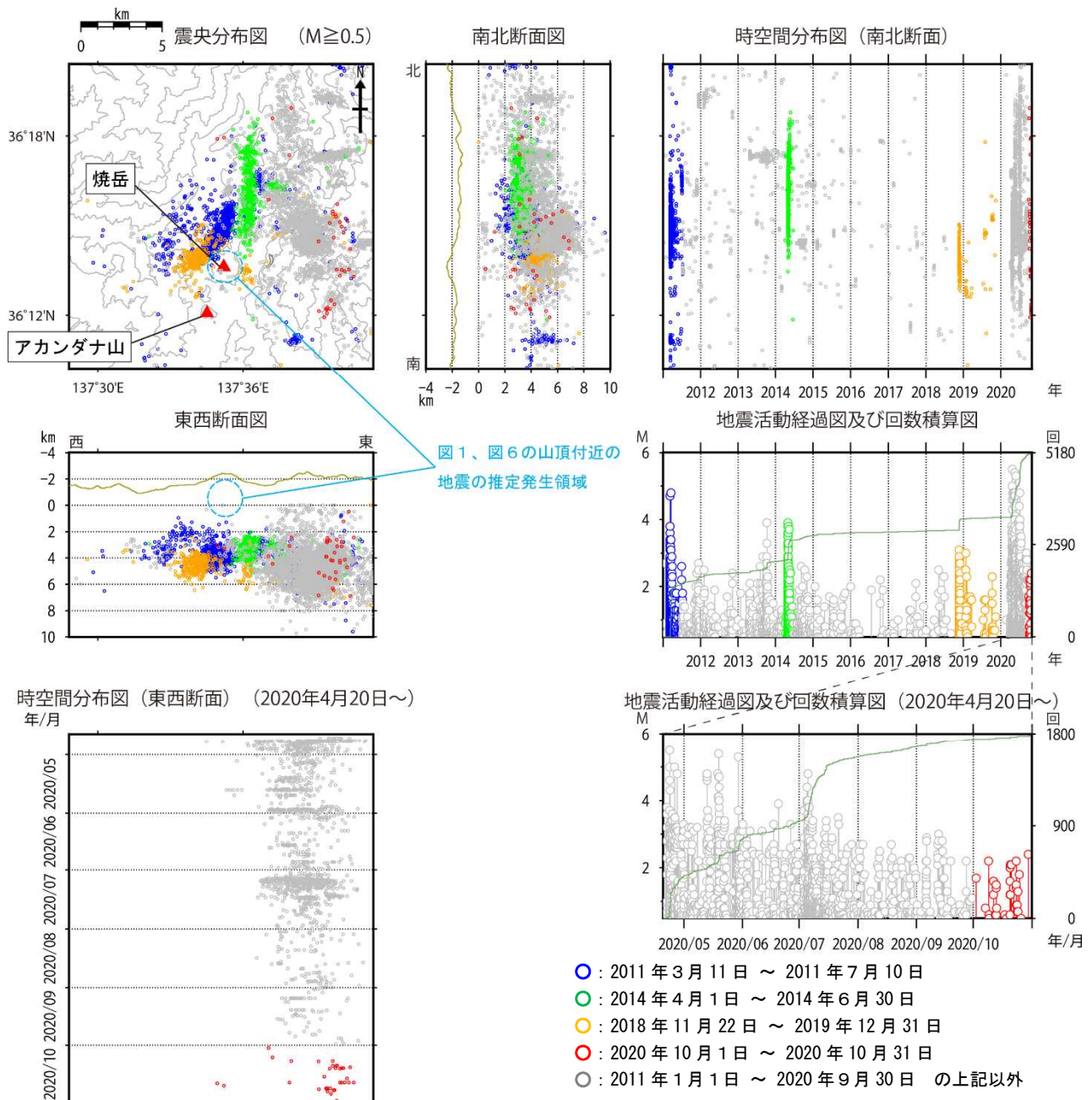
図2 焼岳 広域地震観測網による山体及び周辺の地震活動(2011年1月1日～2020年10月31日)
