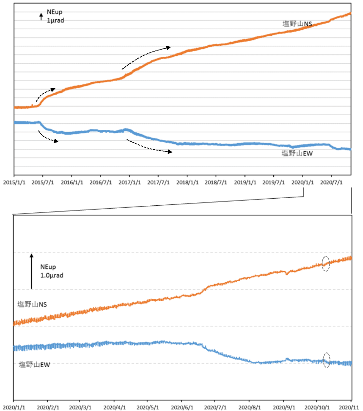
図8 浅間山 塩野山観測点における傾斜データ（2015年1月1日～2020年10月31日）
