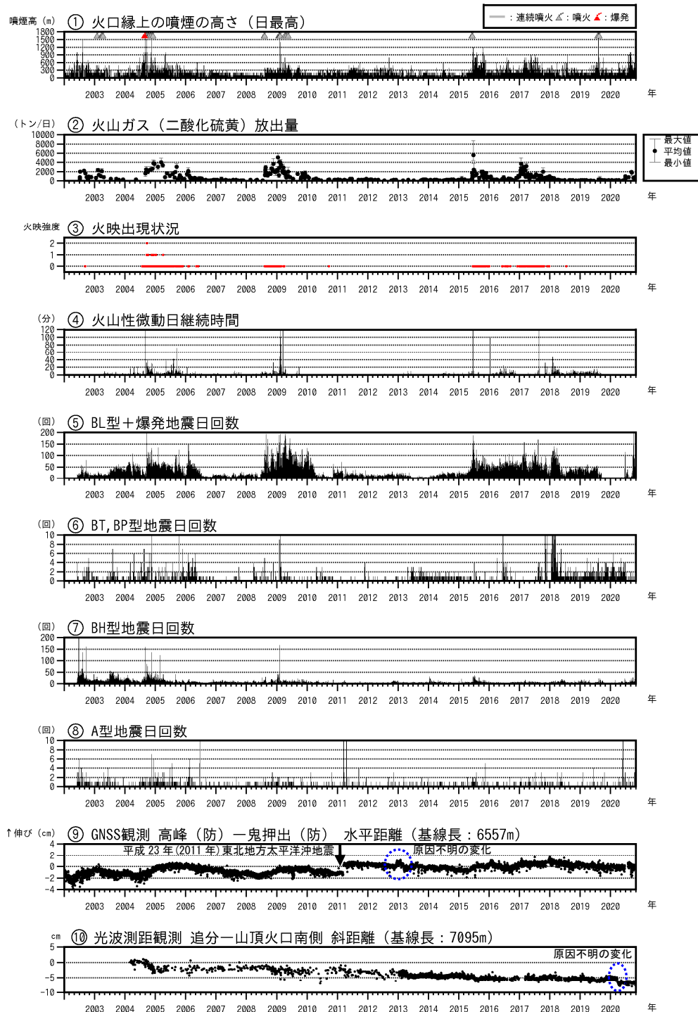
図3 浅間山 火山活動経過図（2002年1月1日～2020年10月31日）
