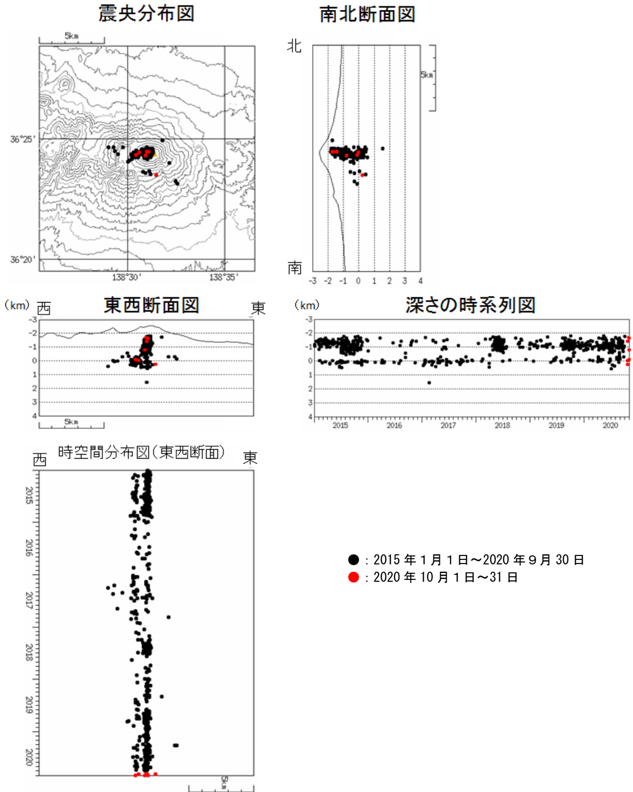
図5 浅間山 震源分布図（2015 年 1 月 1 日～2020 年 10 月 31 日） ・火山性地震の震源は、従来から見られている山頂直下の海拔 1 ～ 2 km 付近と山頂のやや西側の海拔 0 km 付近に分布しています。
