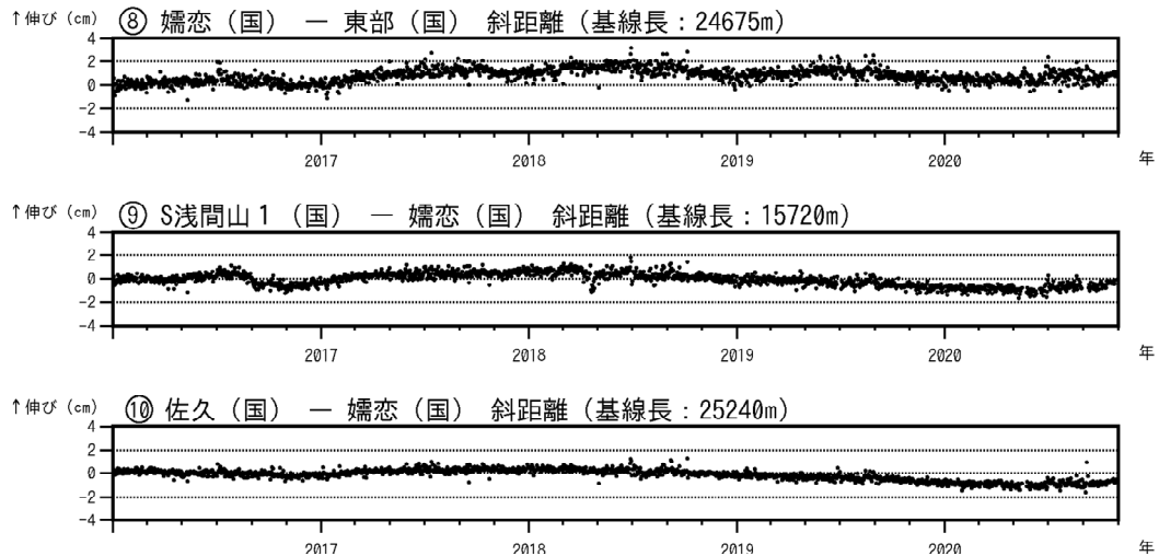
図6-2 浅間山 GNSS 連続観測結果(2016年1月1日~2020年10月31日)
