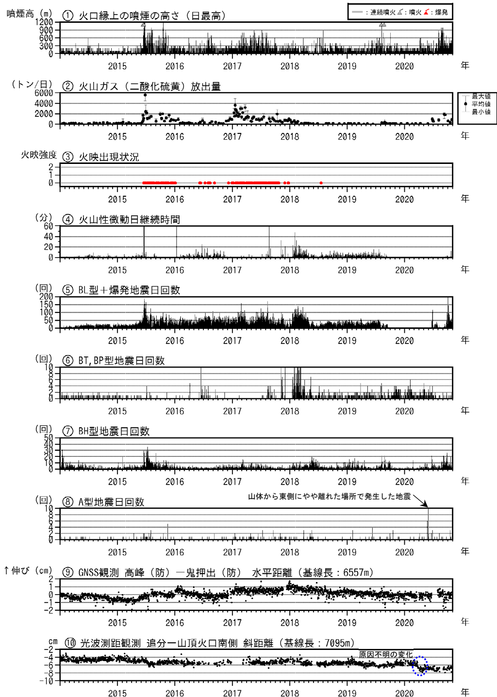
図4 浅間山 最近の火山活動経過図（2014年1月1日～2020年10月31日）
