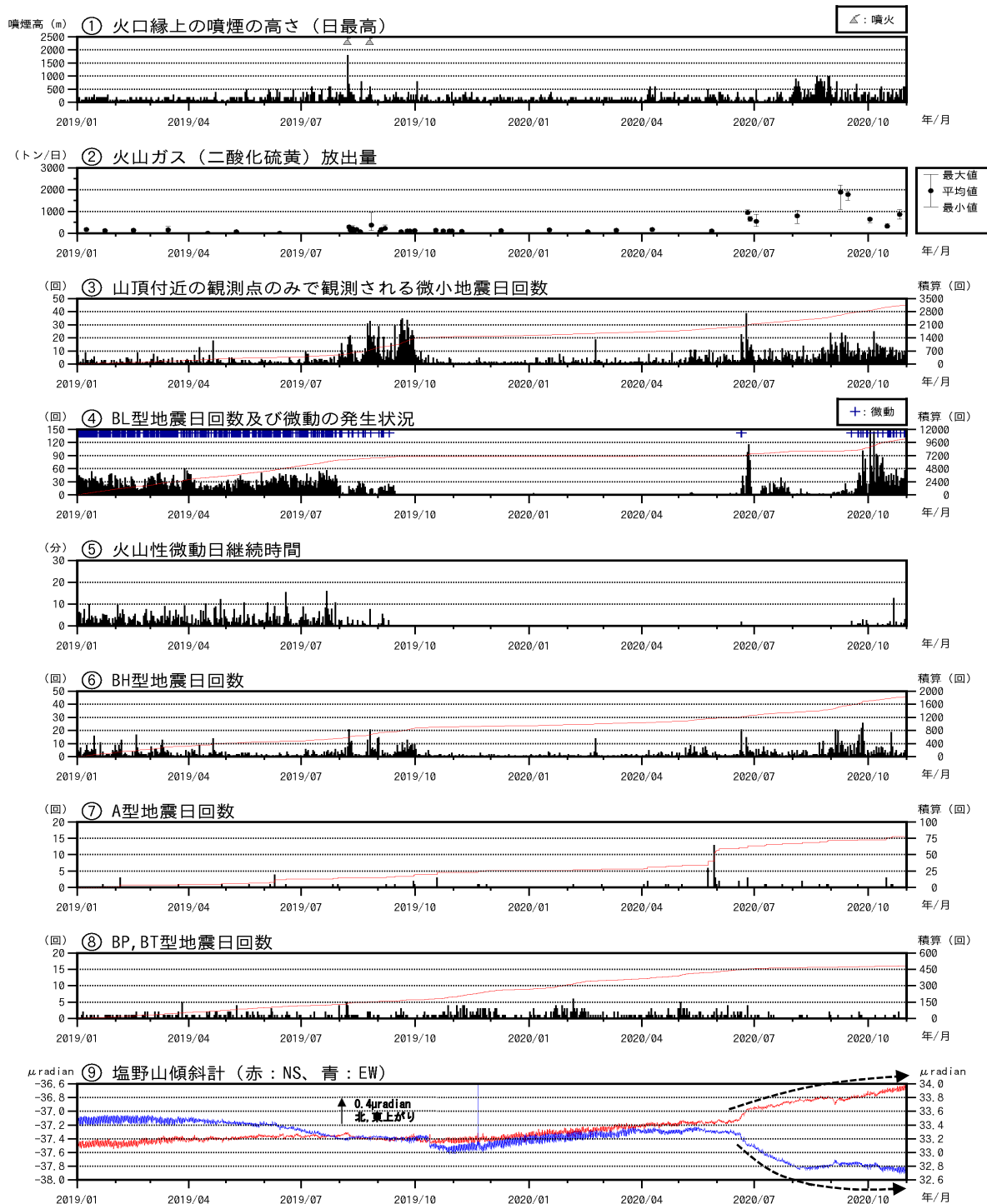
図2 浅間山 火山活動経過図（2019年1月1日～2020年10月31日）
