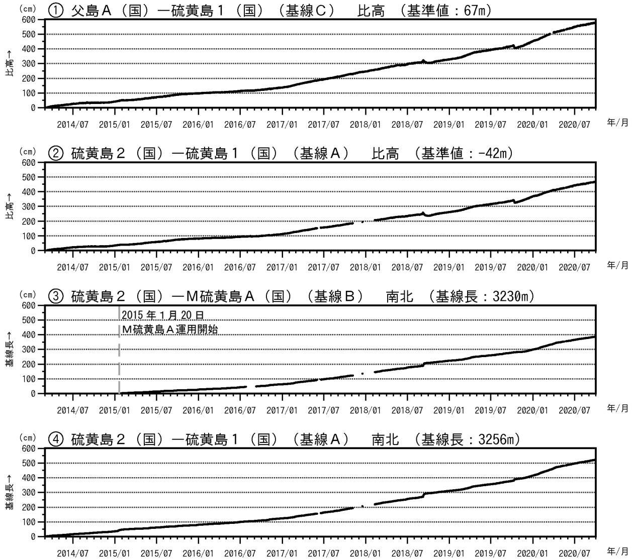
図5 硫黄島 GNSS 連続観測結果（2014年3月1日～2020年9月30日）
