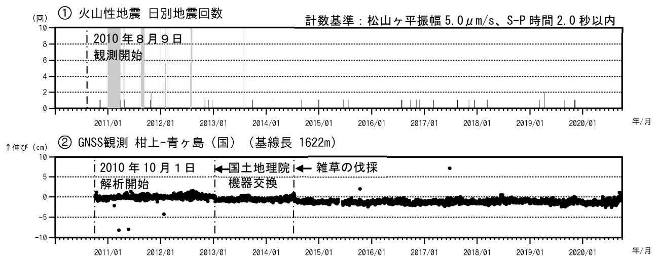
図3 青ヶ島 火山活動経過図（2010年8月9日～2020年9月30日）
