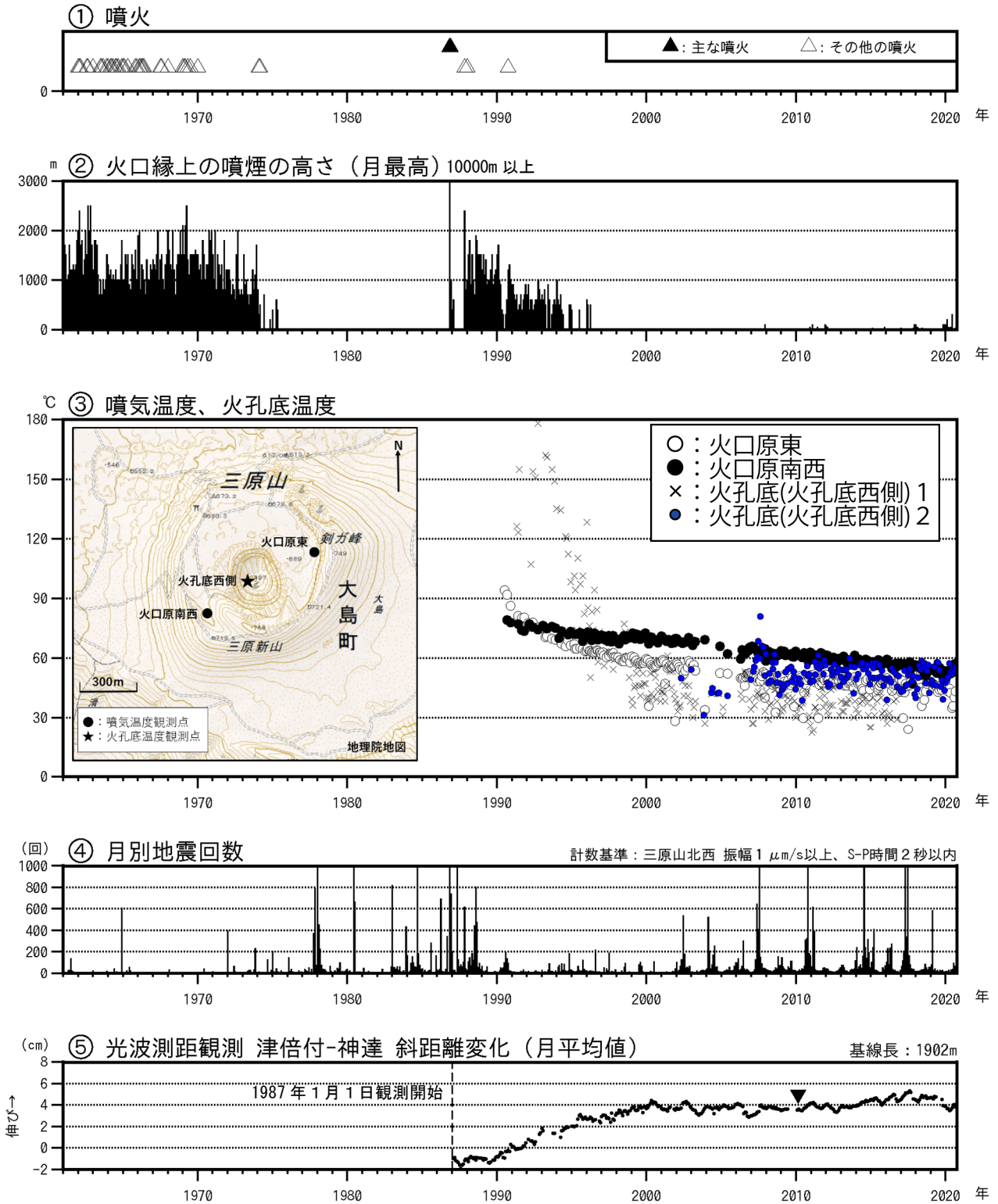
図1 伊豆大島 長期間の火山活動経過図（1961年1月～2020年9月30日）
