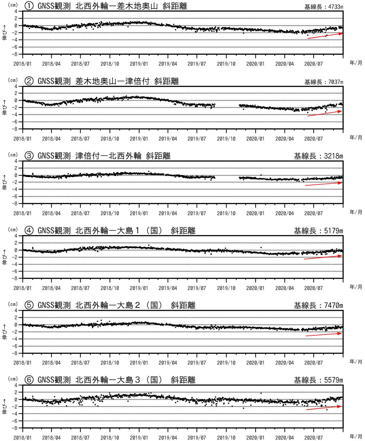
図3-2 伊豆大島 GNSS連続観測による基線長変化(2018年1月~2020年9月30日)
