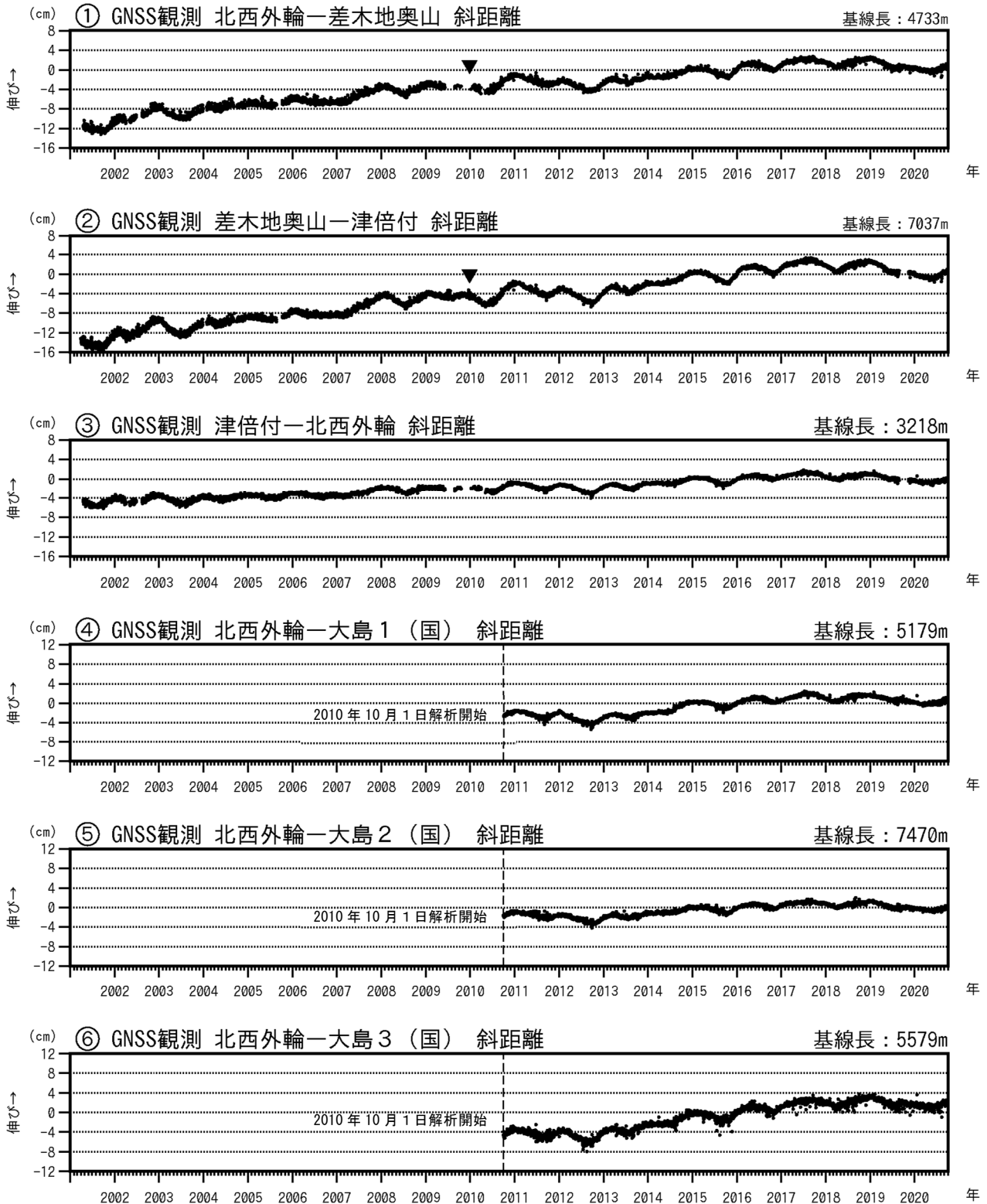
図3-1 伊豆大島 GNSS連続観測による基線長変化(2001年1月～2020年9月30日)
