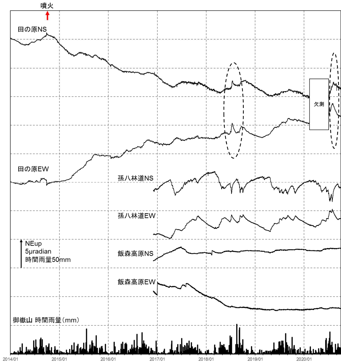
図7 御嶽山 傾斜変動（2014年1月1日～2020年9月30日）
