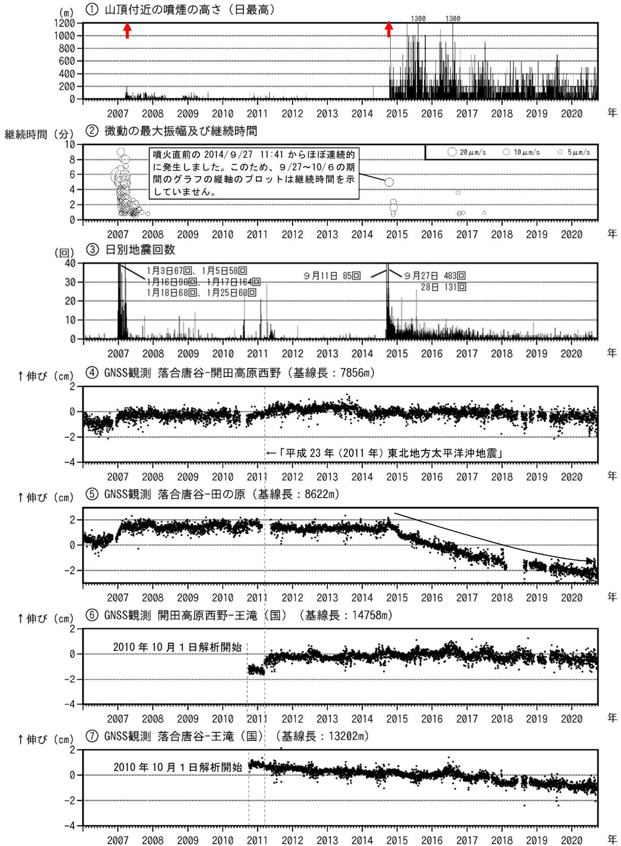
図5 御嶽山 長期間の火山活動経過図（2006年1月1日～2020年9月30日）
