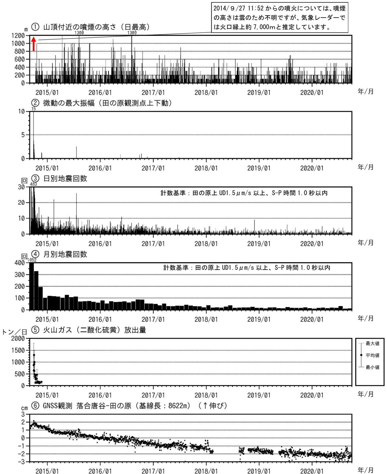
図4 御嶽山 最近の火山活動経過図（2014年9月1日～2020年9月30日）
