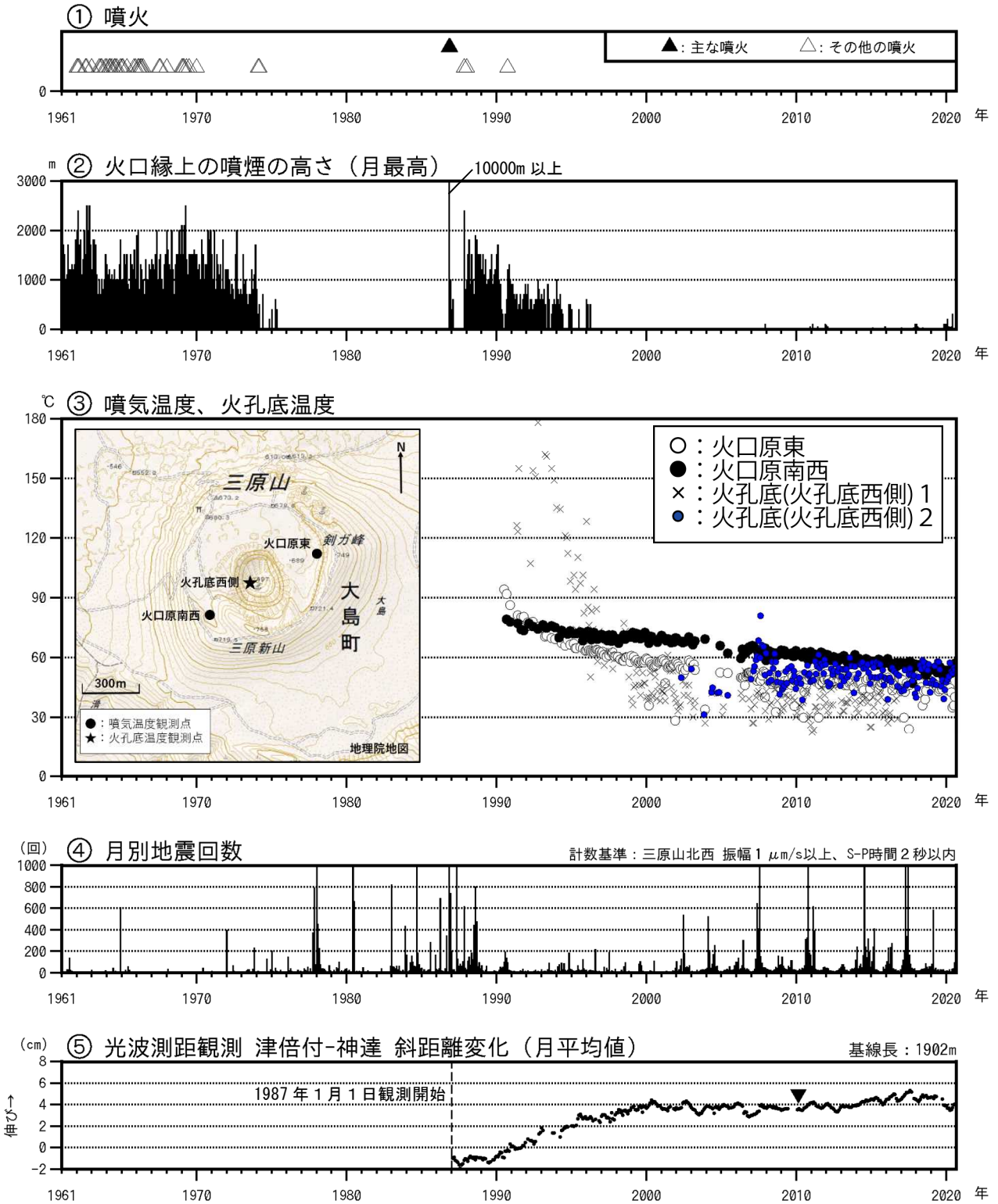
図1 伊豆大島 長期間の火山活動経過図（1961年1月～2020年8月31日）
