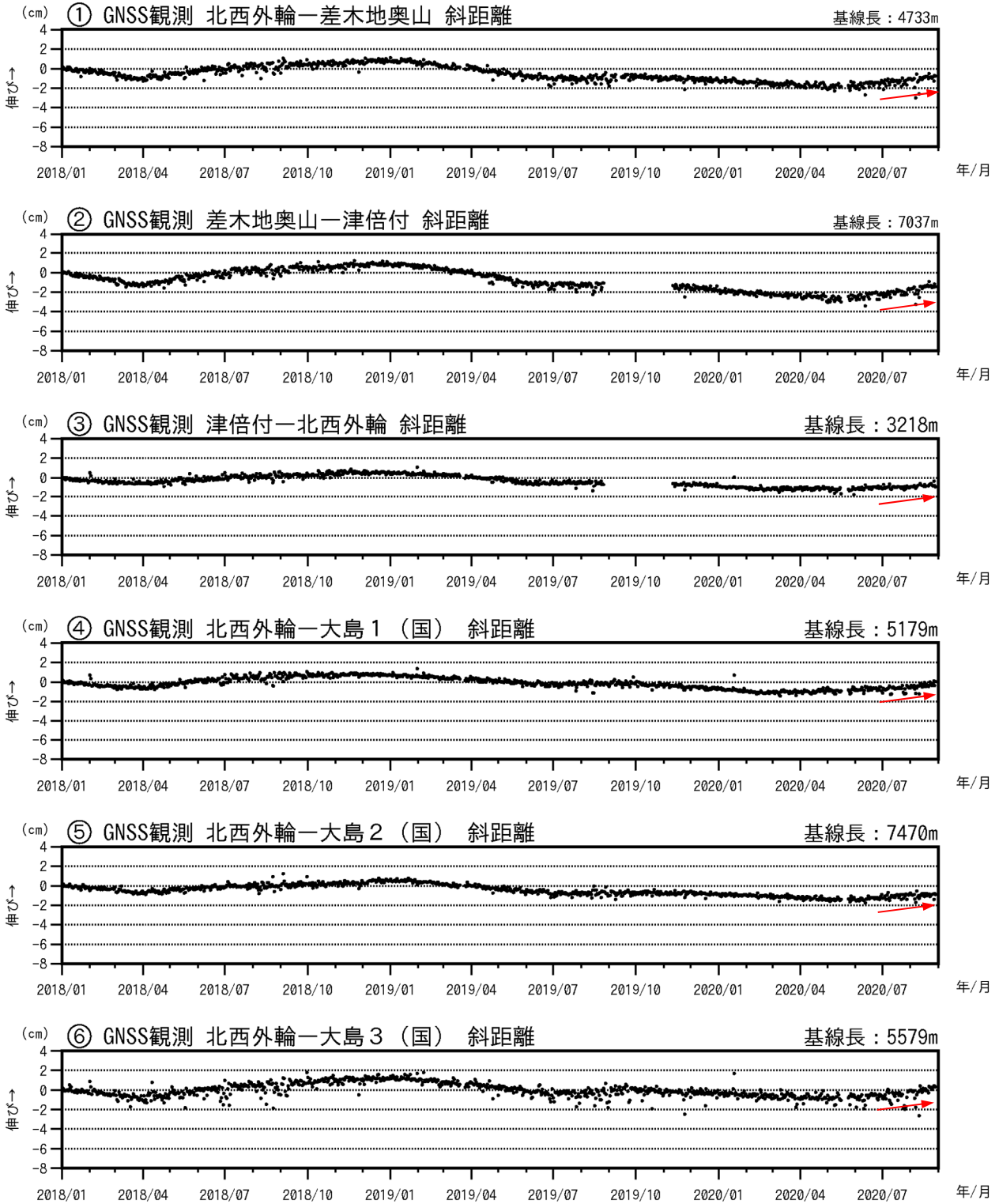
図3-2 伊豆大島 GNSS連続観測による基線長変化(2018年1月~2020年8月31日)
