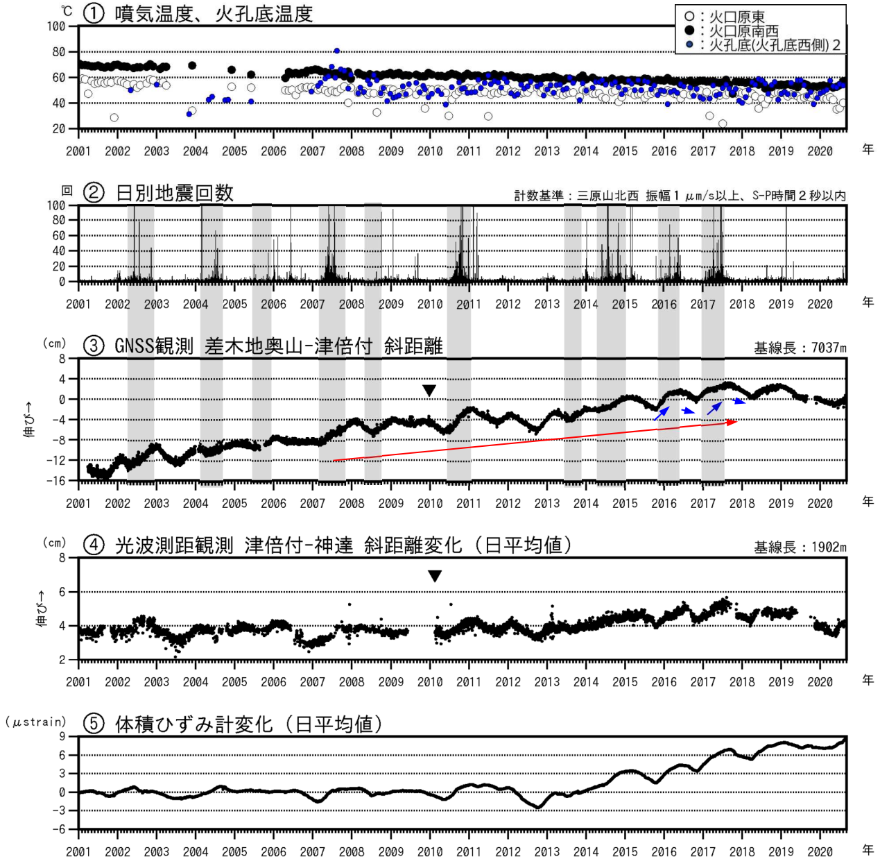
図2 伊豆大島 最近の火山活動経過図（2001年1月～2020年8月31日）
