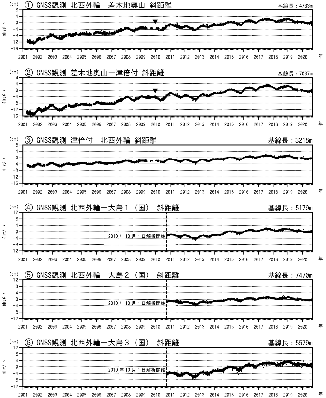
図3-1 伊豆大島 GNSS連続観測による基線長変化(2001年1月~2020年8月31日)
