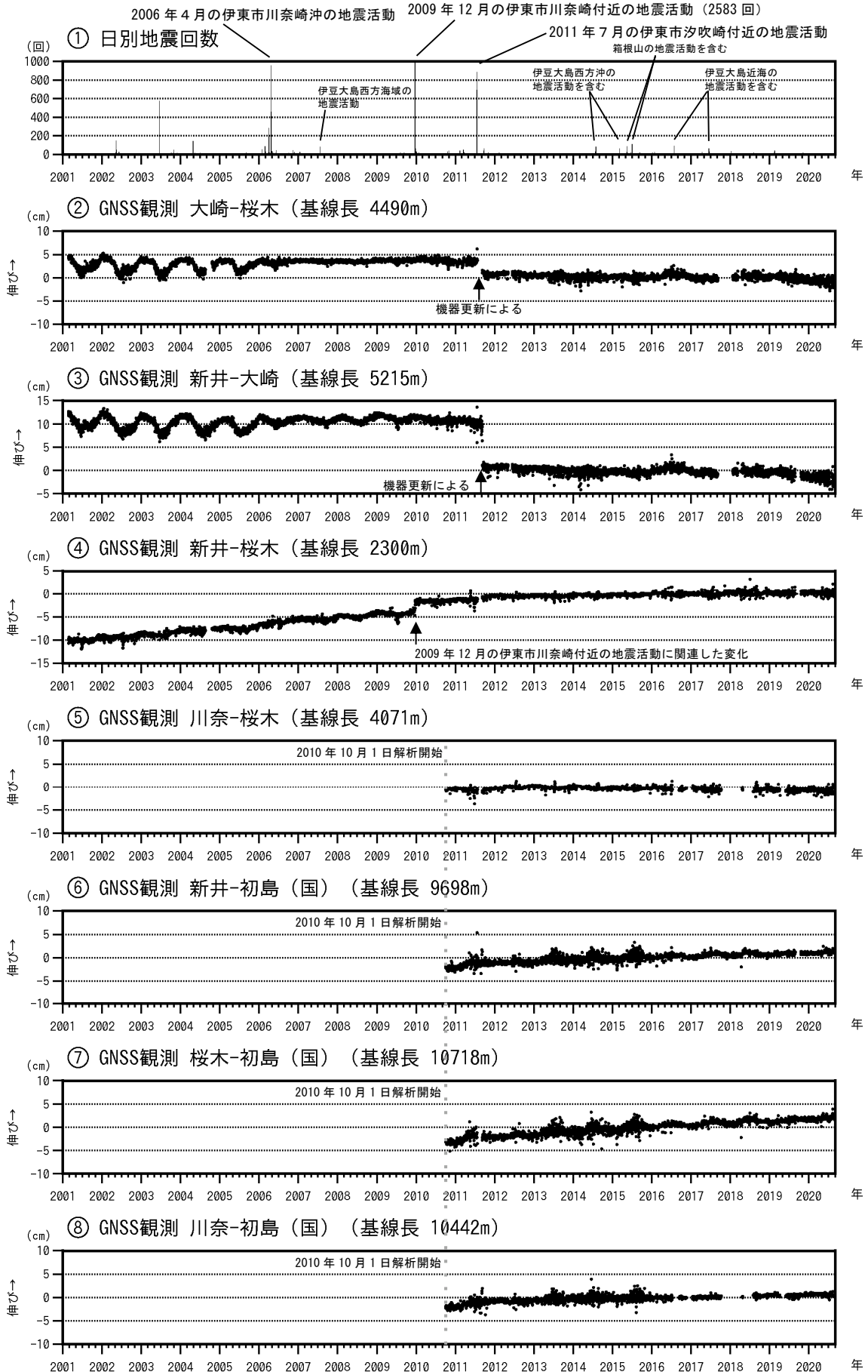
図3 伊豆東部火山群 火山活動経過図（2001年1月1日～2020年8月31日）
