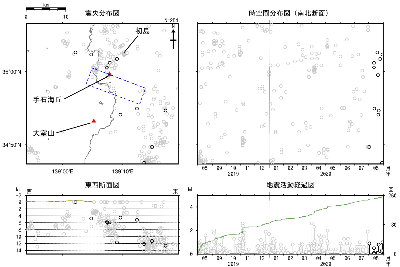
図2 伊豆東部火山群 広域地震観測網による震源分布図（2019年8月1日～2020年8月31日）
