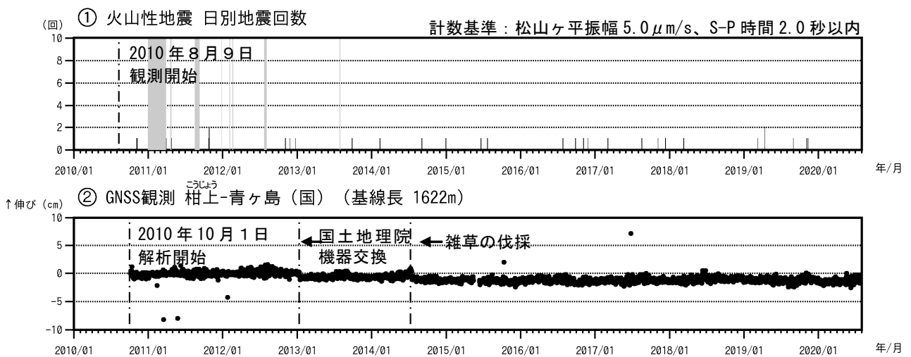
図3 青ヶ島 火山活動経過図（2010年8月9日～2020年7月31日）
