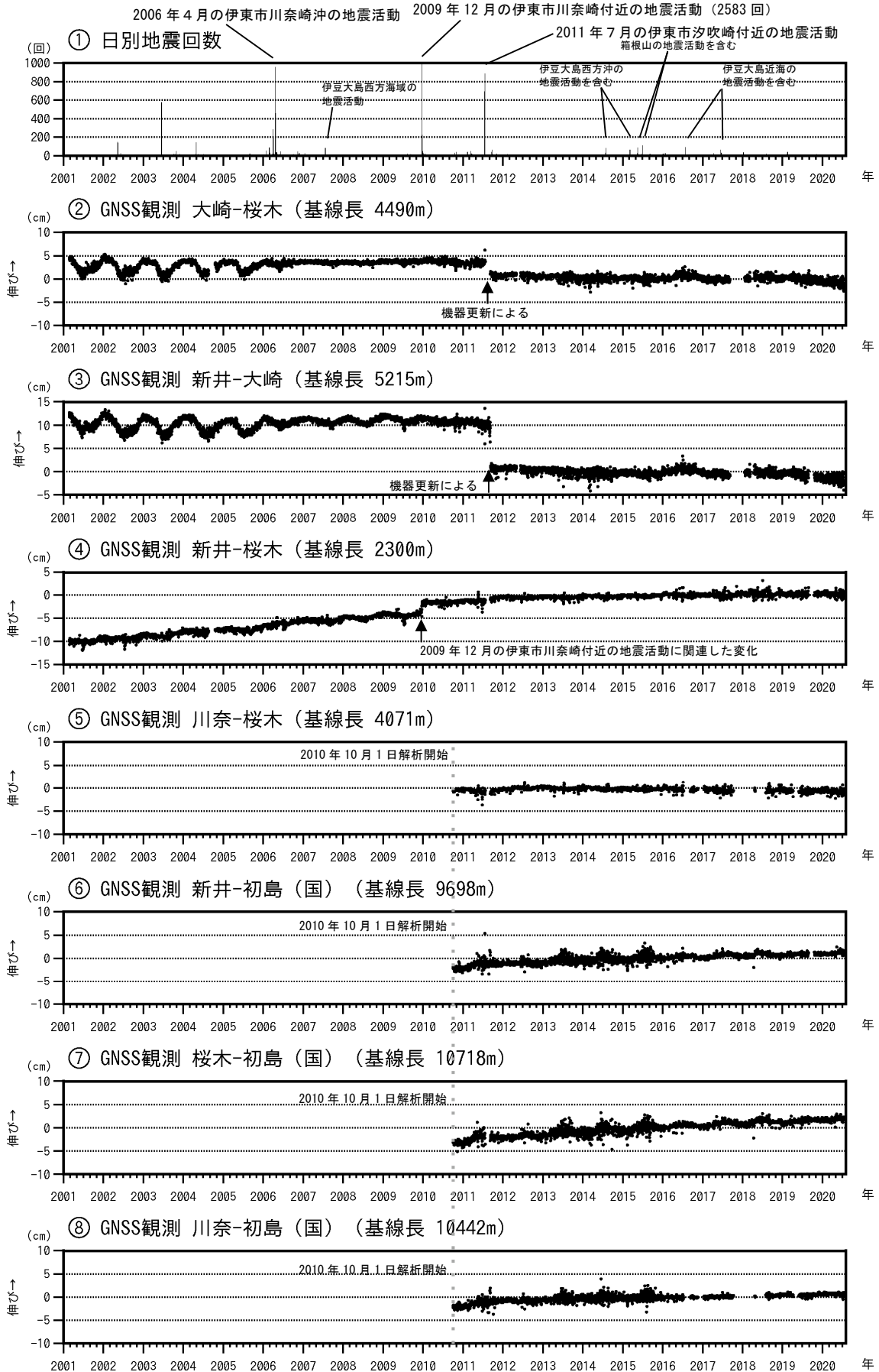
図3 伊豆東部火山群 火山活動経過図 (2001年1月1日~2020年7月31日)
