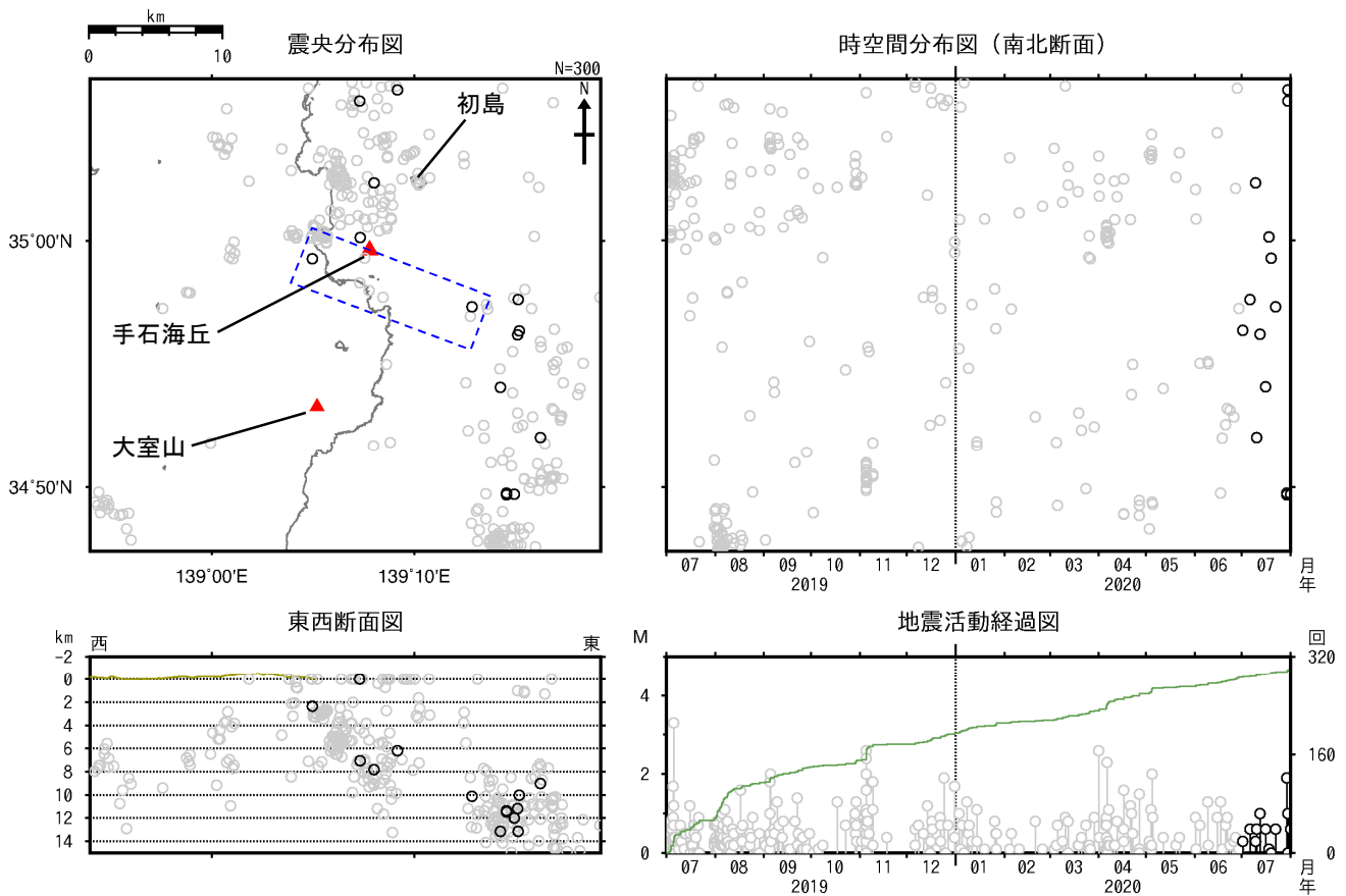
図2 伊豆東部火山群 広域地震観測網による震源分布図（2019年7月1日～2020年7月31日）
