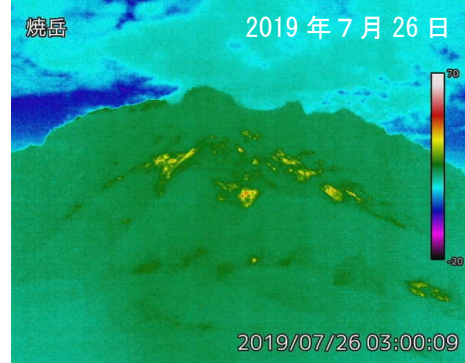
図5 焼岳 中尾峠赤外熱映像カメラによる焼岳の北側斜面の地表面温度分布と可視画像 撮影場所と撮影方向は図10を参照下さい。 ・前月（左下図）及び前年（右下図）と比較して、噴気の状態や地表面温度分布に特段の変化は認められません。
