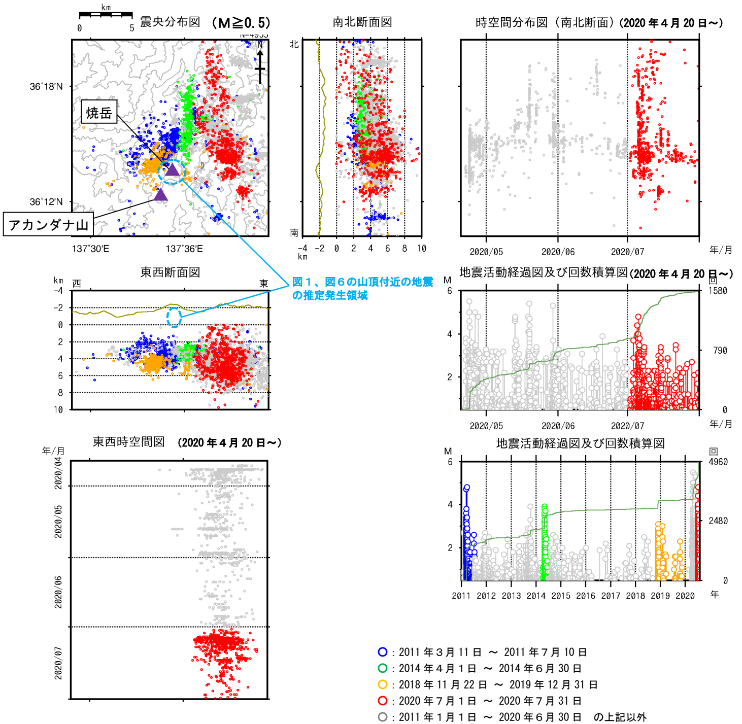
図2 焼岳 広域地震観測網による山体及び周辺の地震活動(2011年1月1日～2020年7月31日)
