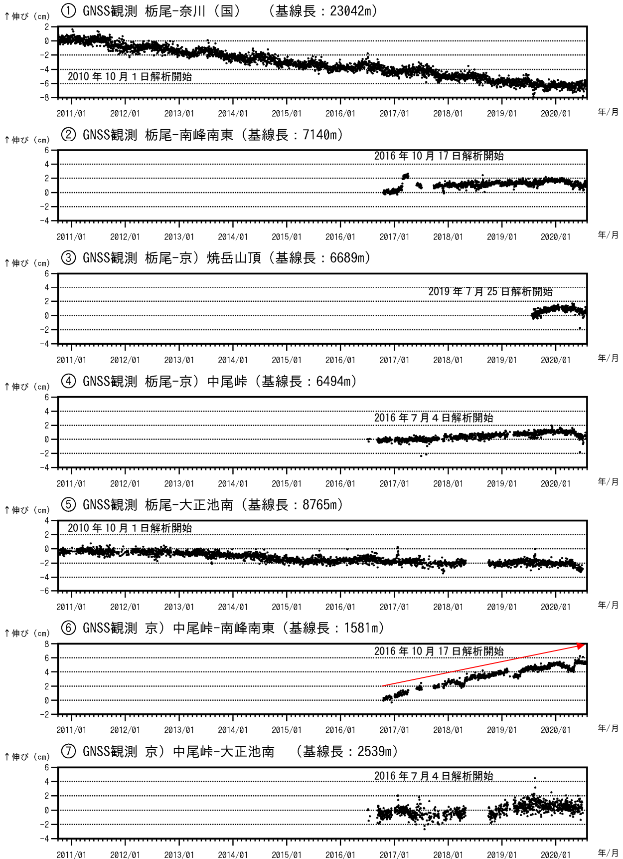
図7 焼岳 GNSS 連続観測による基線長変化 (2010年10月1日~2020年7月31日)
