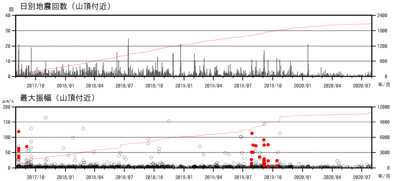
図1 焼岳 山頂付近の地震回数、および南峰南東観測点上下動最大振幅 (2017年8月1日～2020年7月31日)
