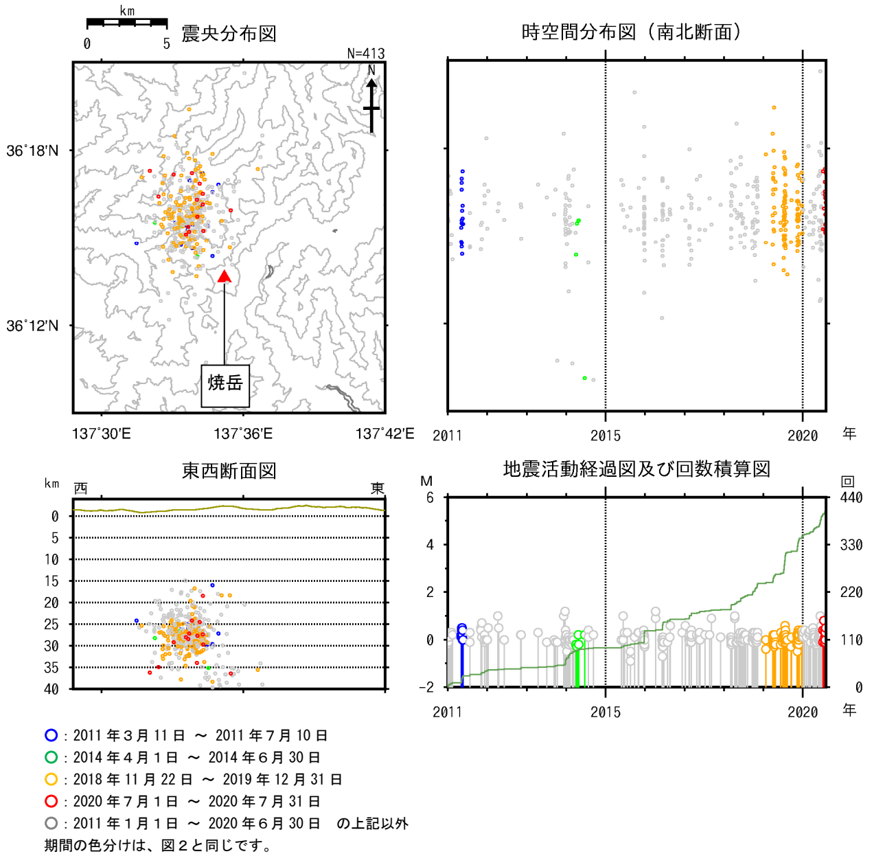
図3 焼岳 深部低周波地震の震源分布図（広域地震観測網による）（2011年1月1日～2020年7月31日）
