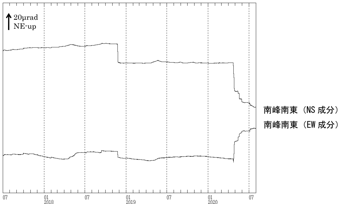
図9 焼岳 南峰南東観測点における傾斜データ（2017年7月1日～2020年7月31日）
