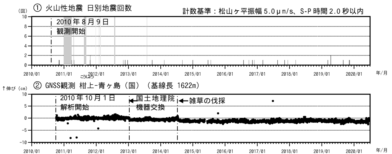
図3 青ヶ島 火山活動経過図（2010年8月9日～2020年6月30日） グラフの灰色部分は機器障害による欠測。 （国）：国土地理院、図4のGNSS基線 に対応。グラフの空白部分は欠測。
