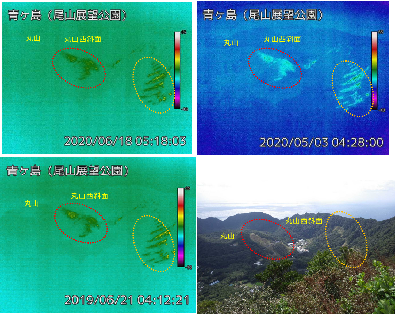
図2 青ヶ島 カルデラ内の地表面温度の状況（左上，右上，左下：尾山展望公園監視カメラによる、右下：2016年3月15日に撮影した同場所からの写真） ・地熱活動（赤点線及び黄色点線で示した範囲）に変化は認められません。
