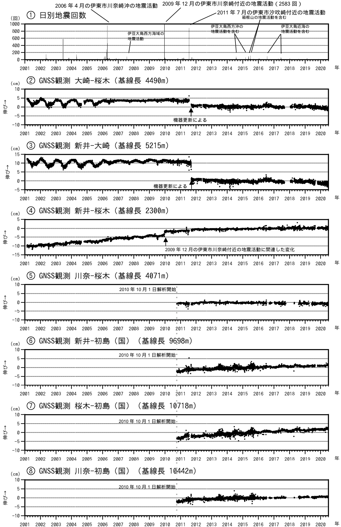
図3 伊豆東部火山群 火山活動経過図（2001年1月1日～2020年6月30日）
