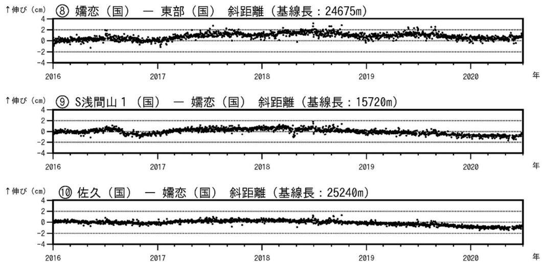
図8-2 浅間山 GNSS 連続観測結果(2016年1月1日~2020年6月30日)
