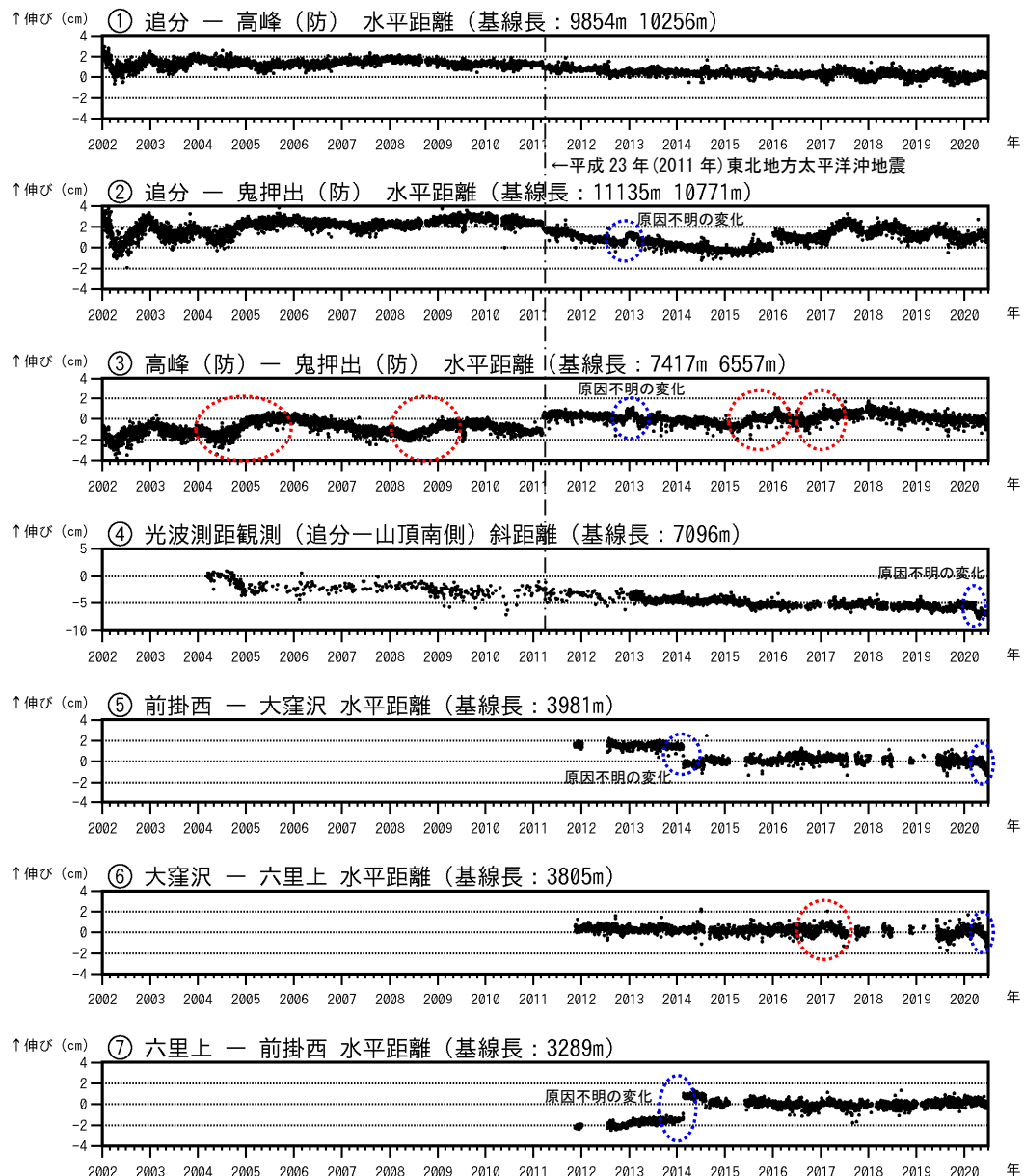
図8-1 浅間山 GNSS 連続観測及び光波測距観測の結果
