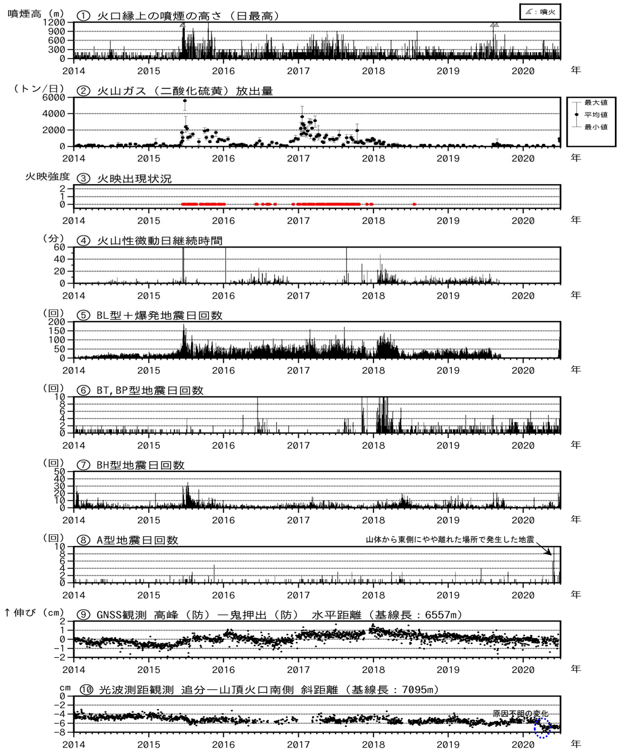
図6 浅間山 最近の火山活動経過図 (2014年1月1日~2020年6月30日)
