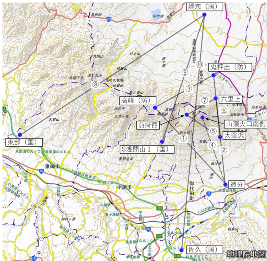
図9 浅間山 地殻変動連続観測点配置図
