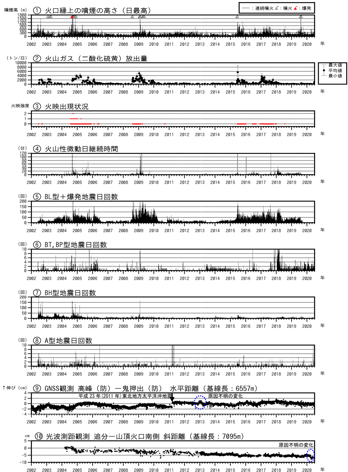
図5 浅間山 火山活動経過図（2002年1月1日～2020年6月30日）
