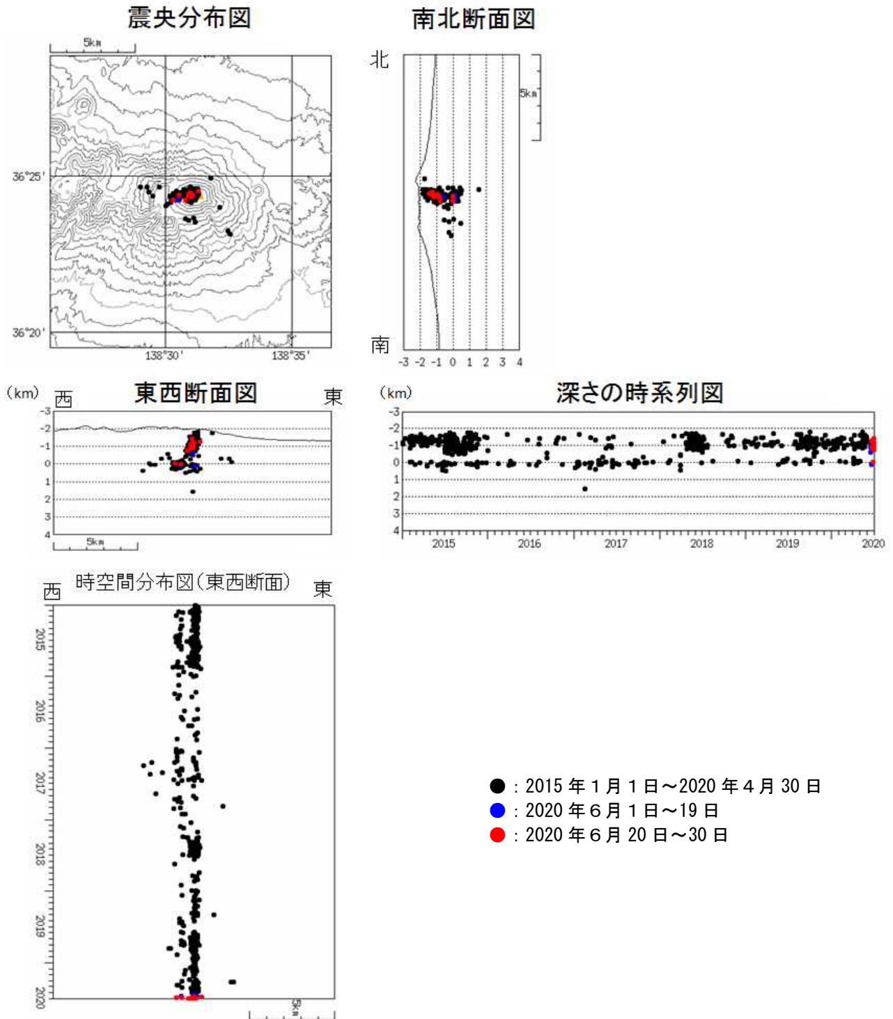
図7 浅間山 震源分布図（2015 年 1 月 1 日～2020 年 6 月 30 日）
