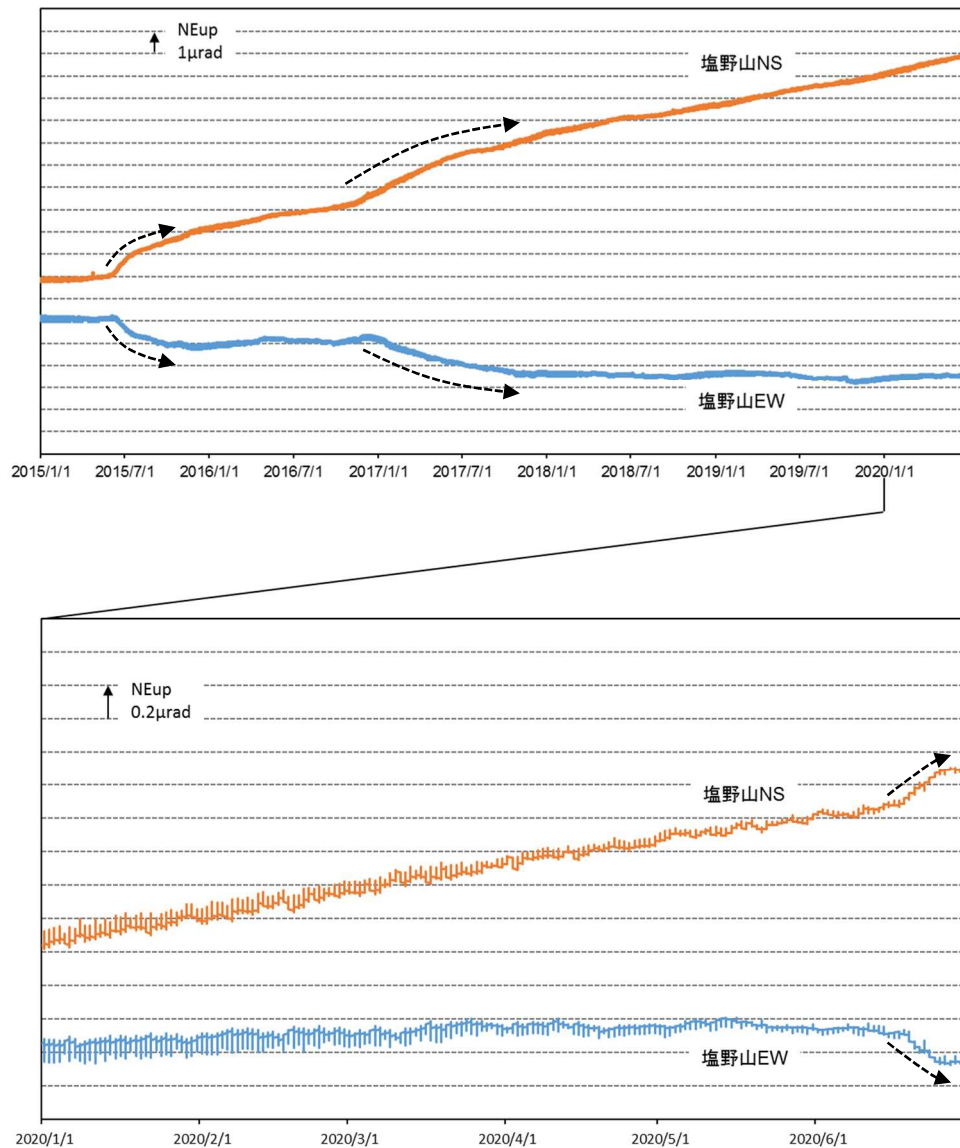
図 10 浅間山 塩野山観測点における傾斜データ（2015 年 1 月 1 日～2020 年 6 月 30 日） データは時間平均値を使用しており、長期にわたるトレンドを補正しています。
