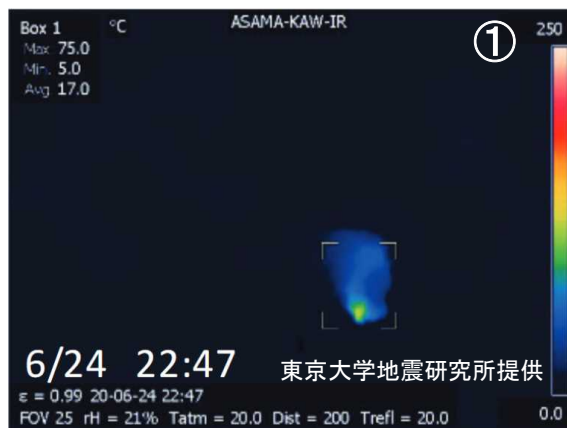
図3 浅間山 赤外熱映像による火口底温度の観測結果（2020年6月20日～30日）
