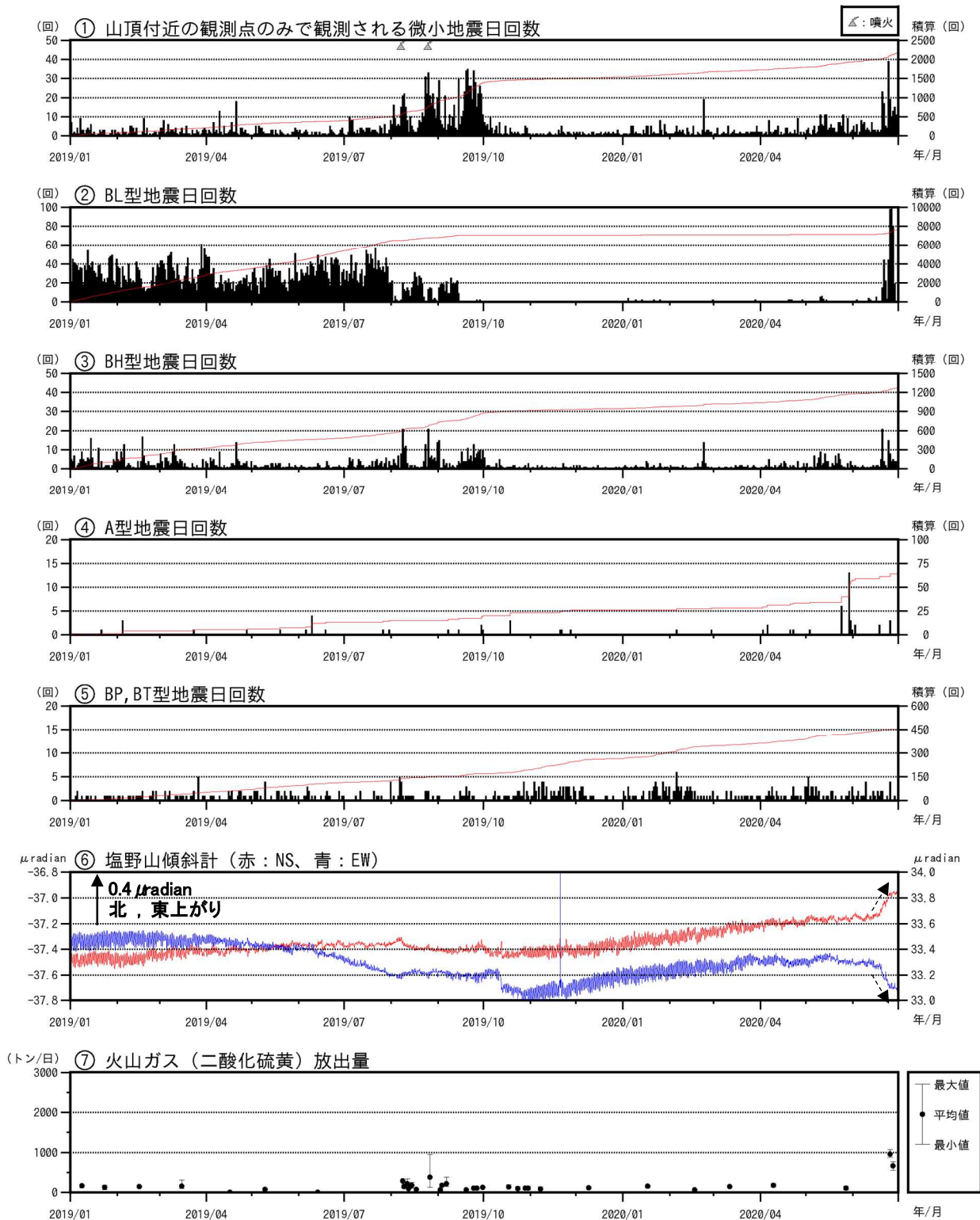
図4 浅間山 火山活動経過図（2019年1月1日～2020年6月30日）
