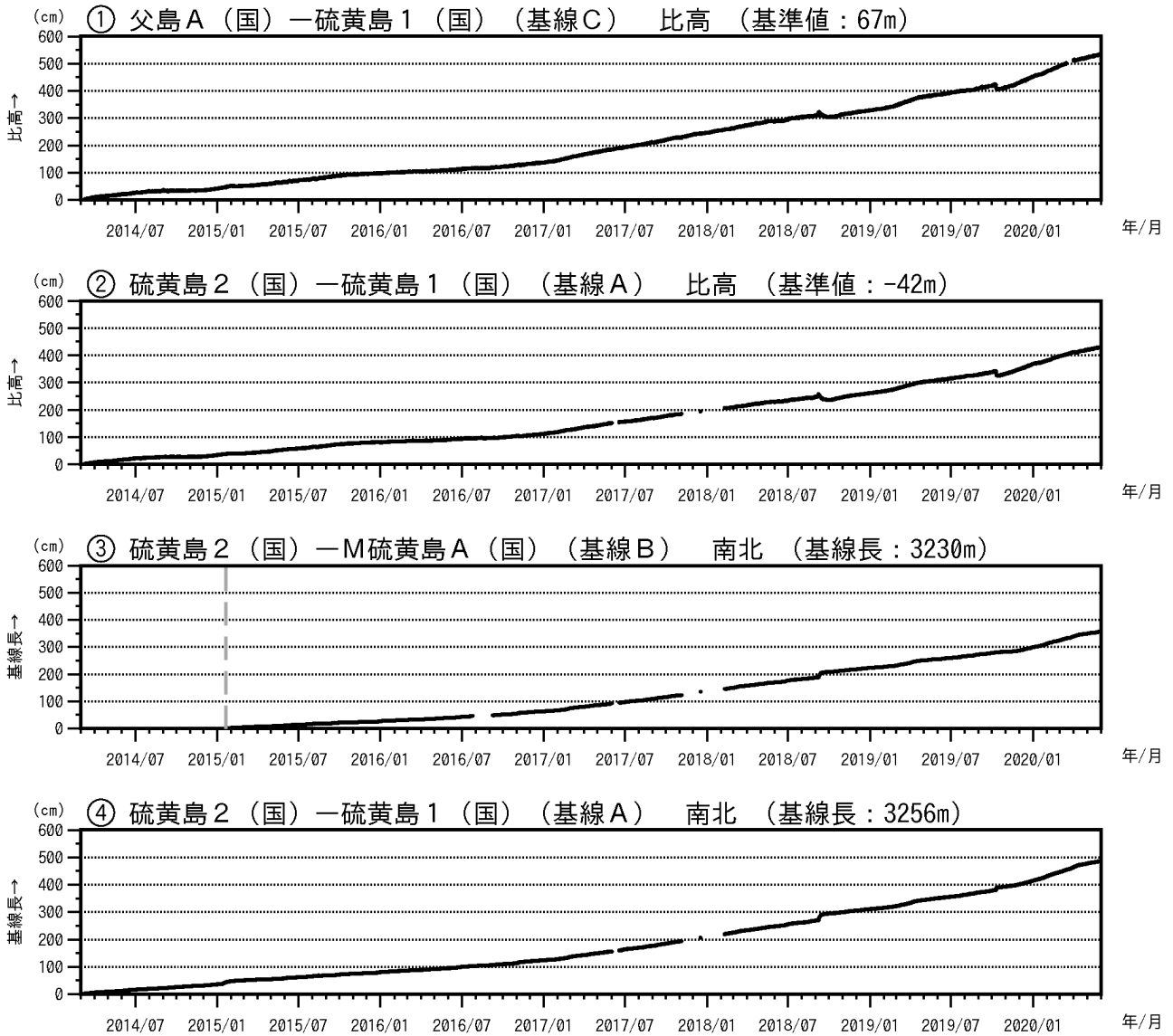
図5 硫黄島 GNSS 連続観測結果（2014年3月1日～2020年5月31日）
