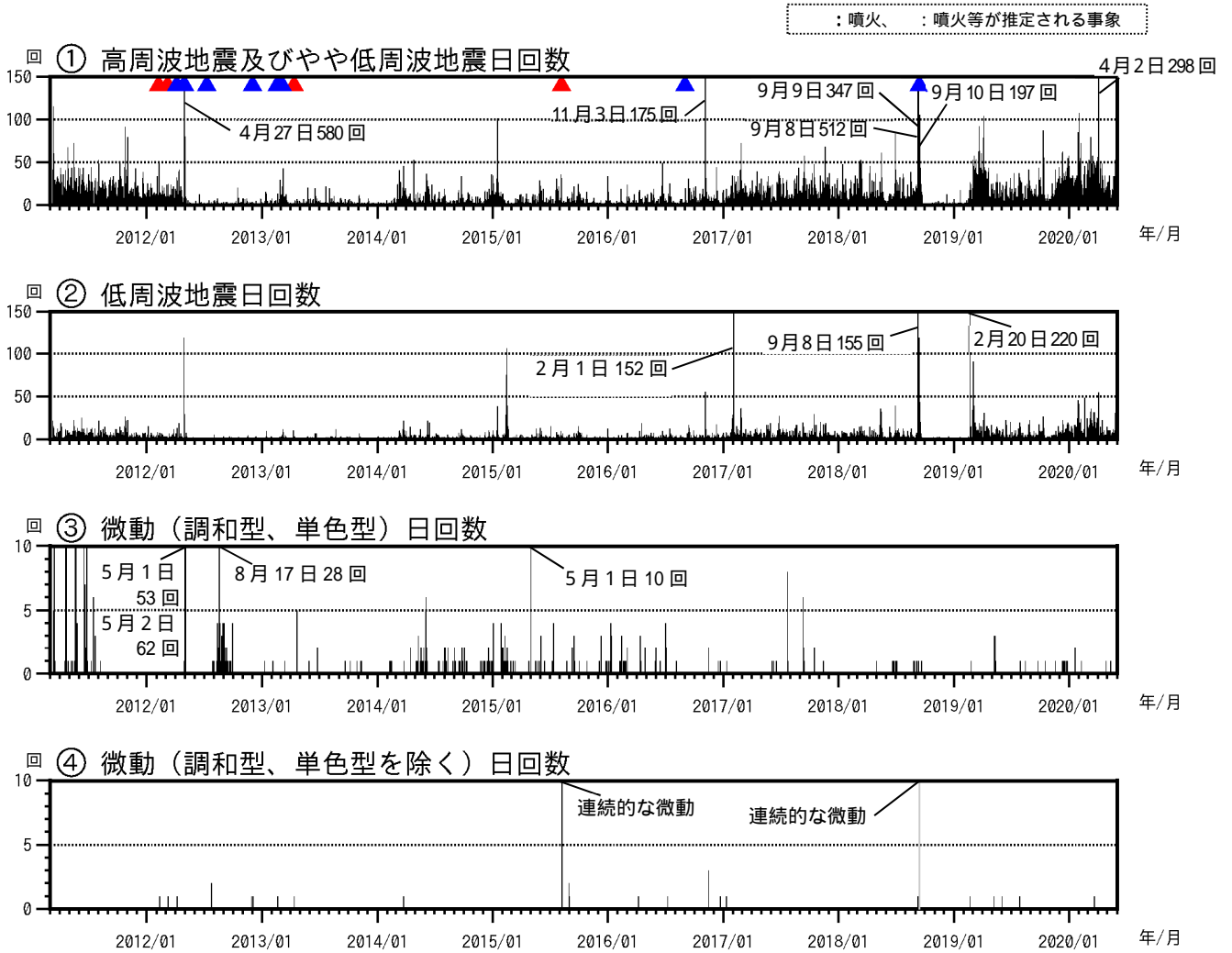
図4 硫黄島 火山活動経過図（2011年3月8日～2020年5月31日）
