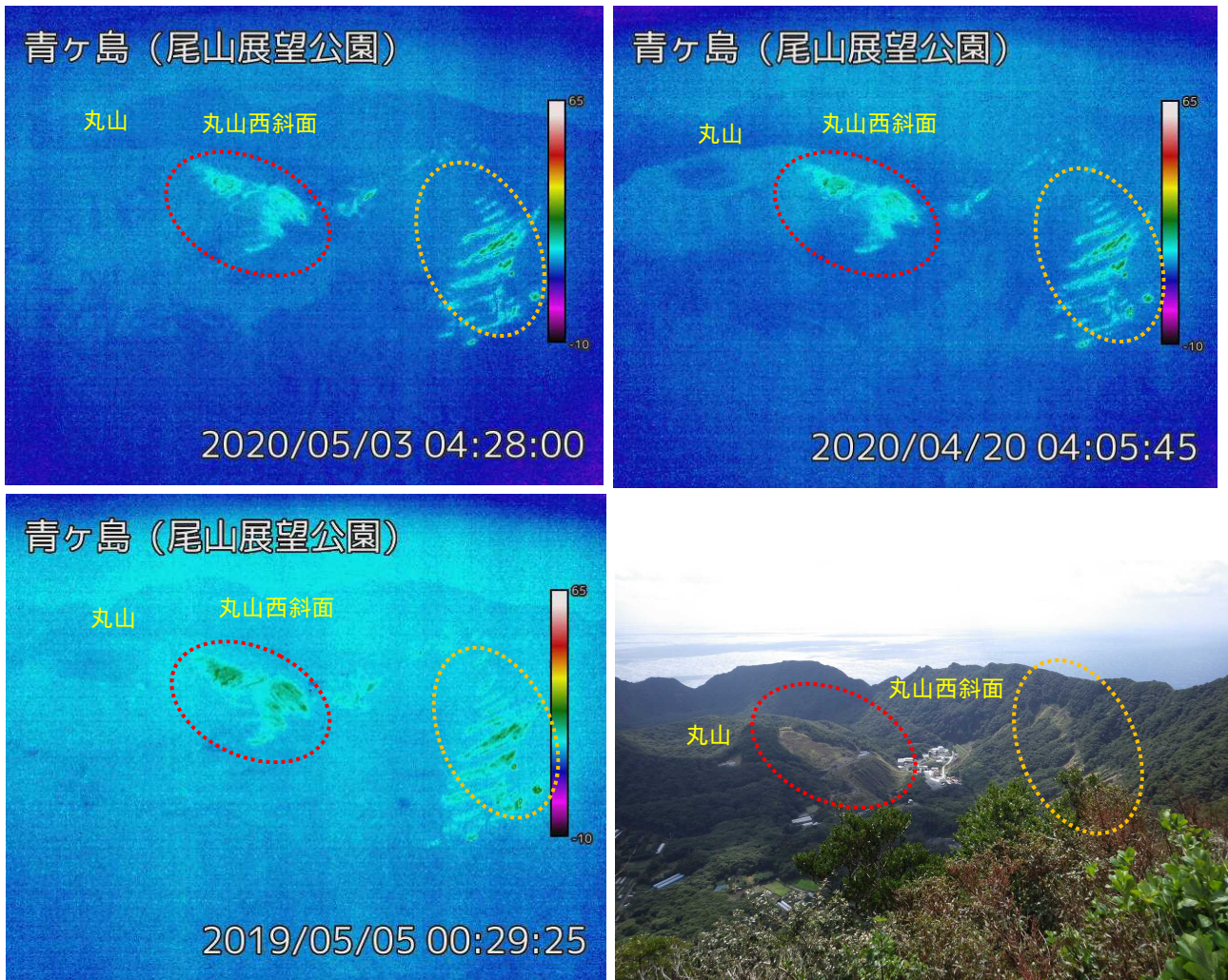
図2 青ヶ島 カルデラ内の地表面温度の状況（左上, 右上, 左下：尾山展望公園監視カメラによる、右下：2016年3月15日に撮影した同場所からの写真）
