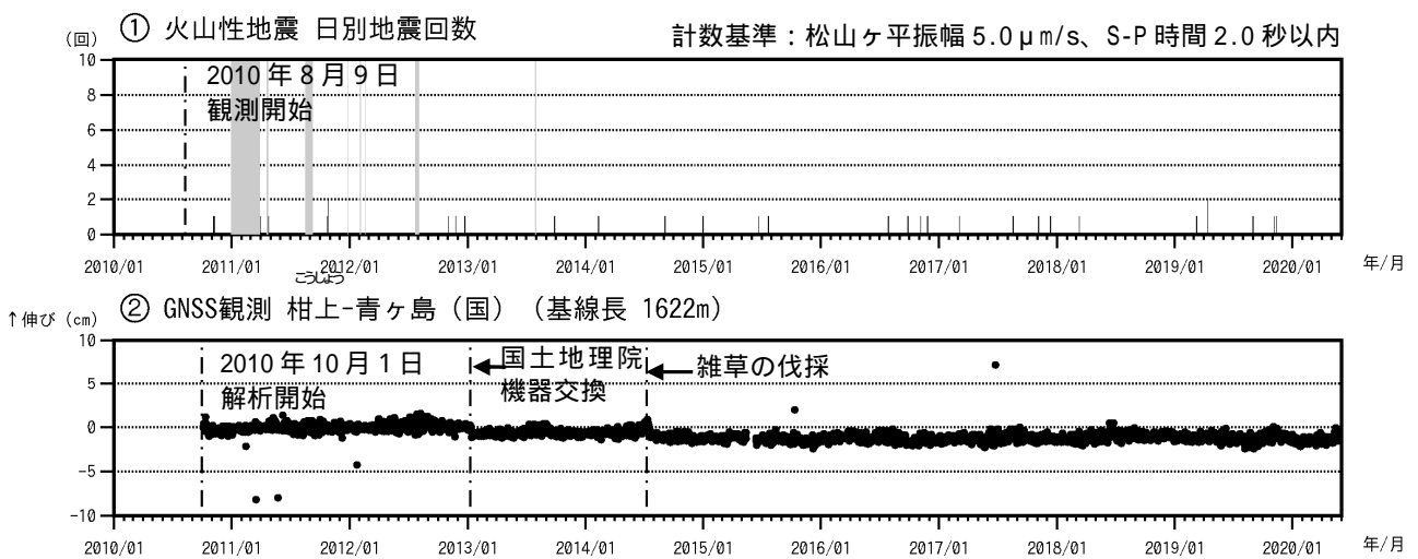
図3 青ヶ島 火山活動経過図（2010年8月9日～2020年5月31日）
