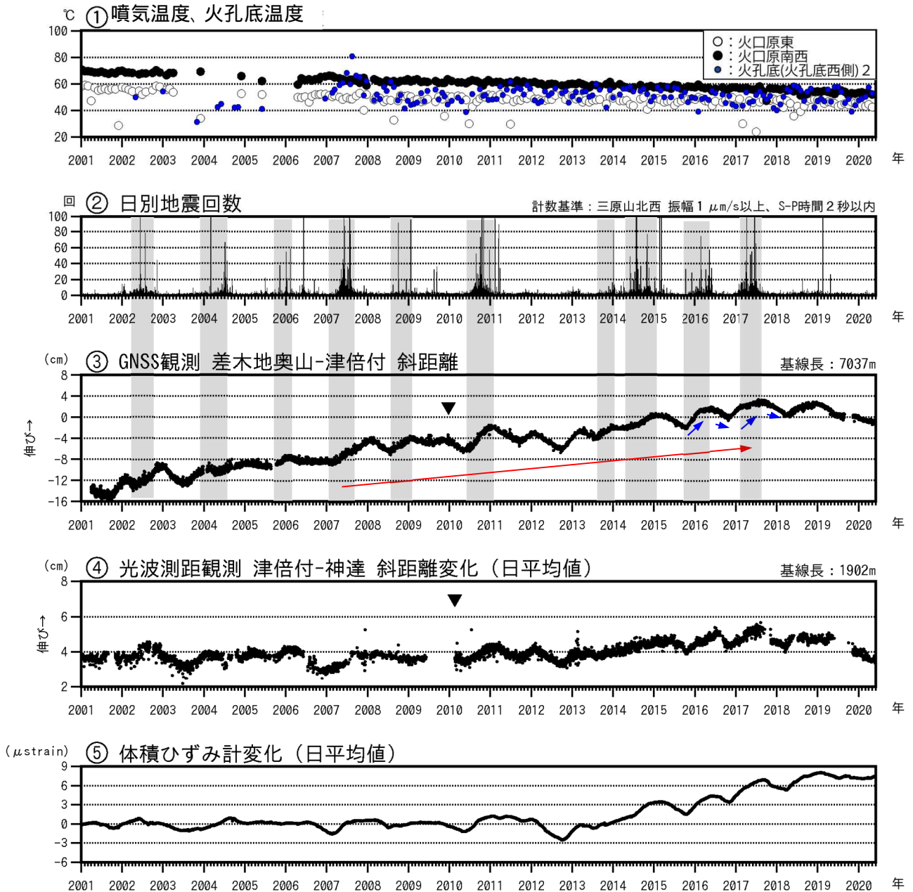
図2 伊豆大島 最近の火山活動経過図（2001年1月～2020年5月31日）
