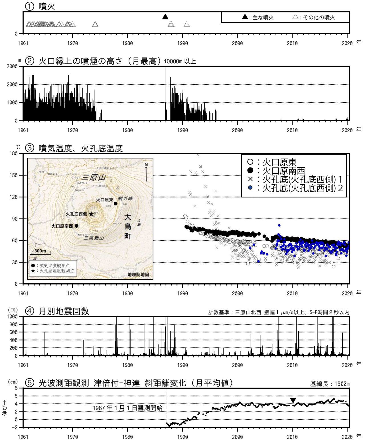
図1 伊豆大島 長期間の火山活動経過図（1961年1月～2020年5月31日）
