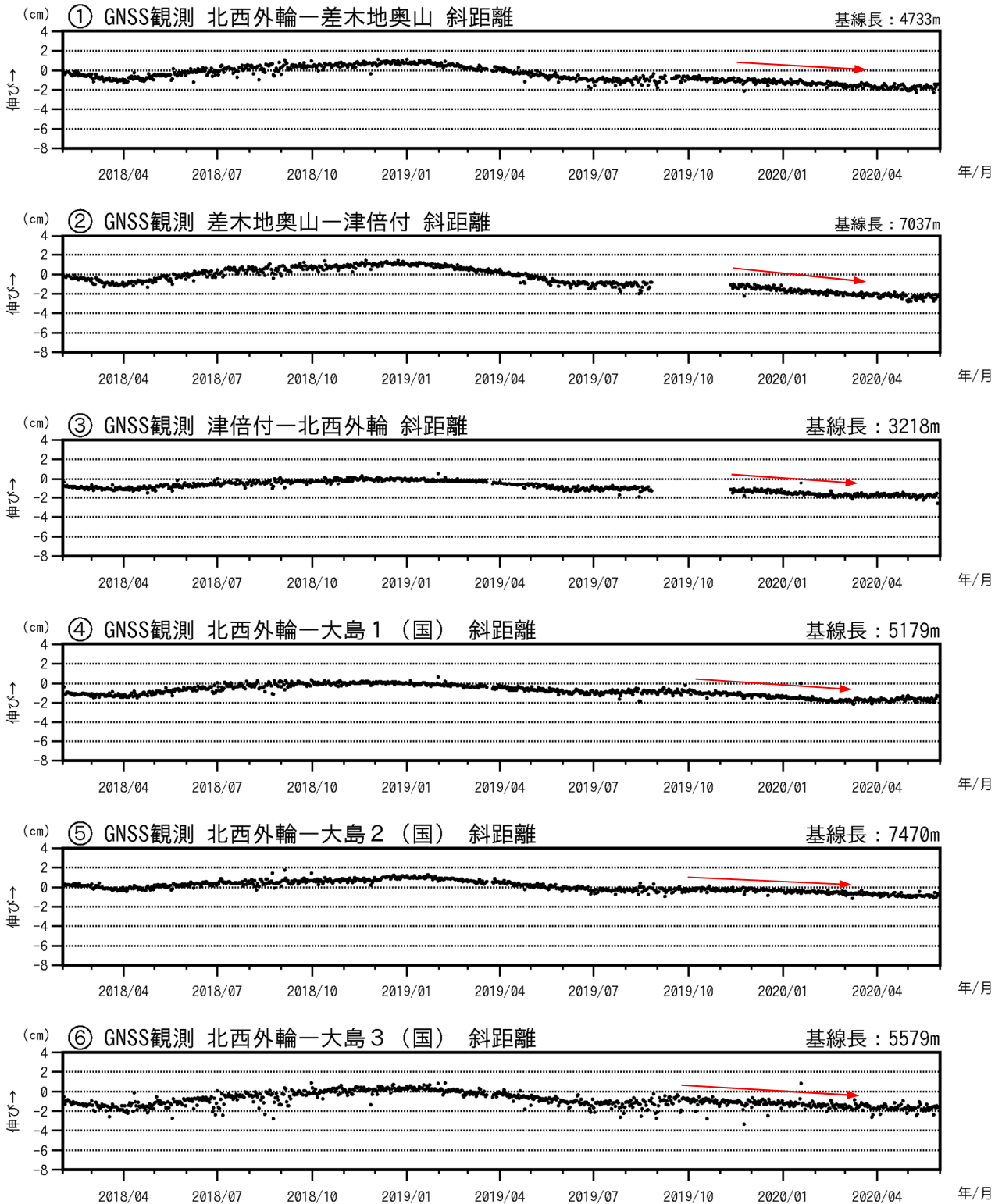
図3-2 伊豆大島 GNSS連続観測による基線長変化(2018年2月~2020年5月31日)
