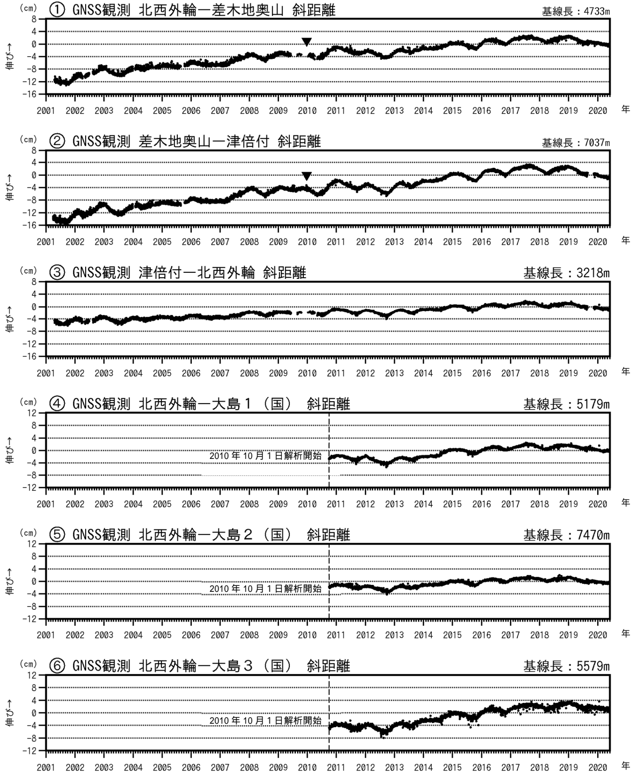
図3-1 伊豆大島 GNSS連続観測による基線長変化(2001年1月～2020年5月31日)
