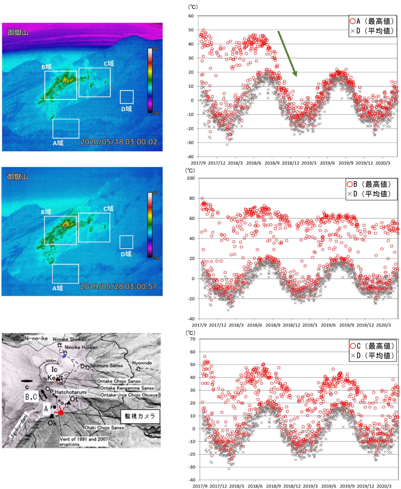
図3 御嶽山 奥の院赤外熱映像カメラによる剣ヶ峰南西側における最高温度の推移（2017年9月13日～2020年5月31日）と同カメラの位置（左下図はOikawa et al., 2016に加筆） A～Cは地熱域、Dは非地熱域を示します。 ・年周変化はみられるものの、B及びC領域については長期的な低下傾向となっています。 ・A領域の温度は2018年秋頃から明瞭に低下し、非地熱域と同程度の温度となっています（緑矢印）。
