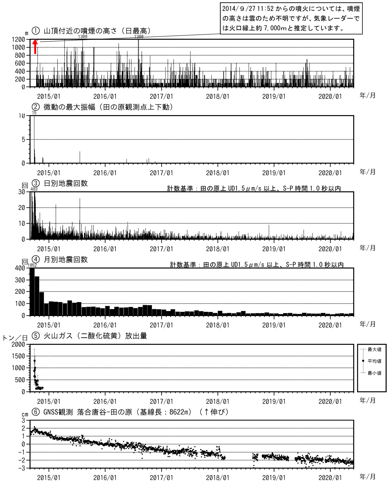
図4 御嶽山 最近の火山活動経過図（2014年9月1日～2020年5月31日）
