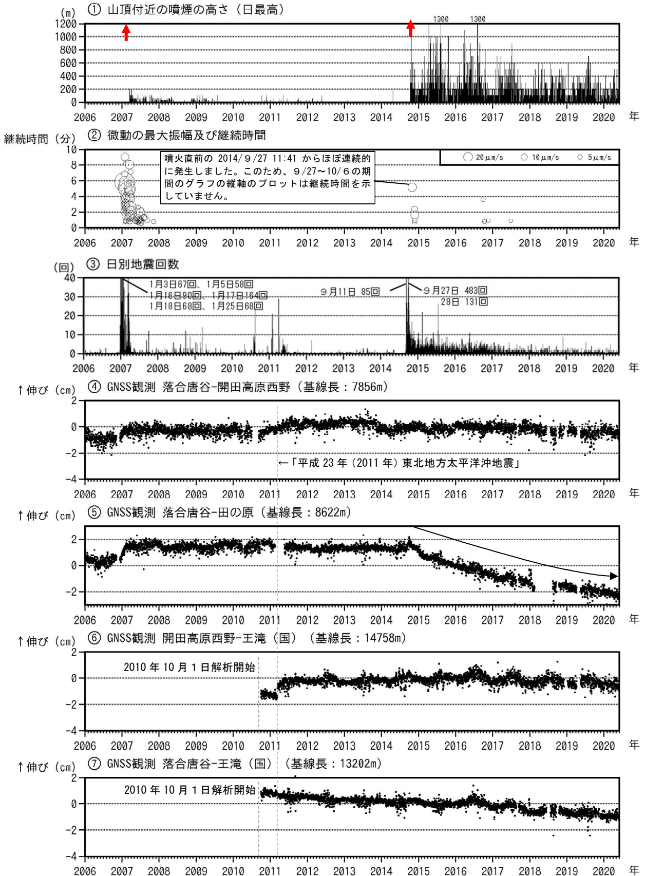
図5 御嶽山 長期間の火山活動経過図（2006年1月1日～2020年5月31日）
