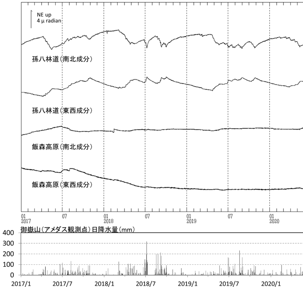
図7 御嶽山 傾斜変動（2017年1月1日～2020年5月31日）
