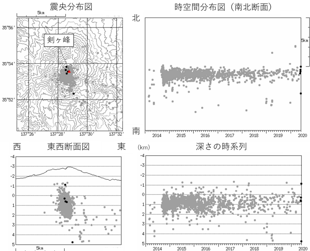
図2 御嶽山 震源分布図（2014年1月1日～2020年5月31日）
