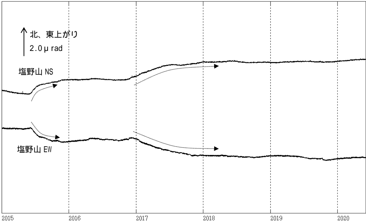
図9 浅間山 塩野山観測点における傾斜データ（2015年1月1日～2020年5月31日）
