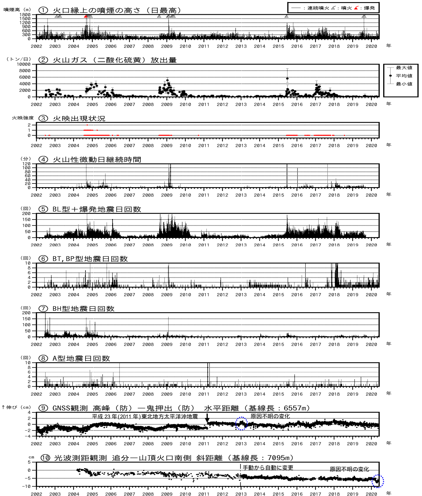
図3 浅間山 火山活動経過図(2002年1月1日~2020年5月31日)
