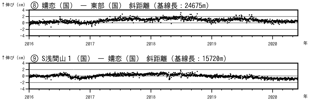
図7 - 2 浅間山 GNSS 連続観測結果(2016年1月1日~2020年5月31日)
