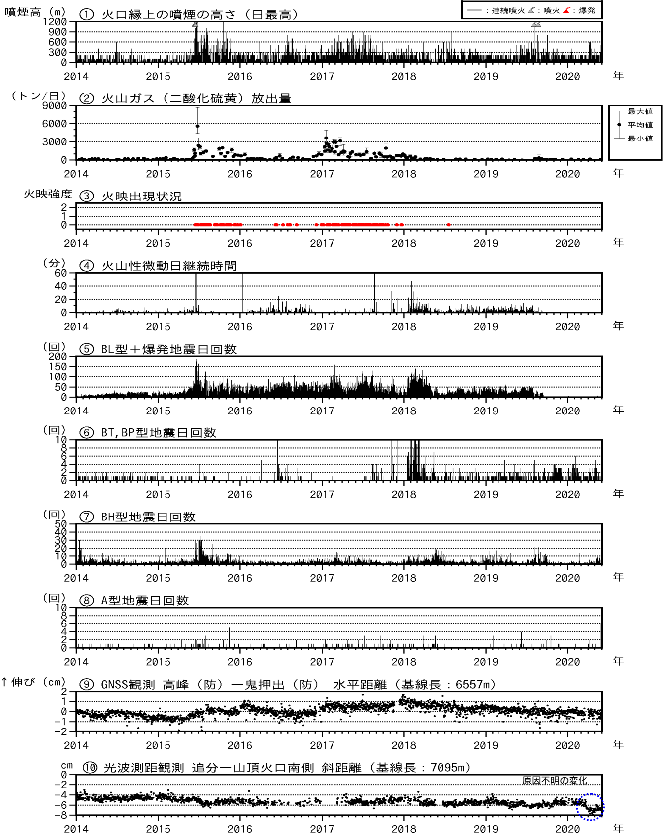
図4 浅間山 最近の火山活動経過図（2014年1月1日～2020年5月31日）
