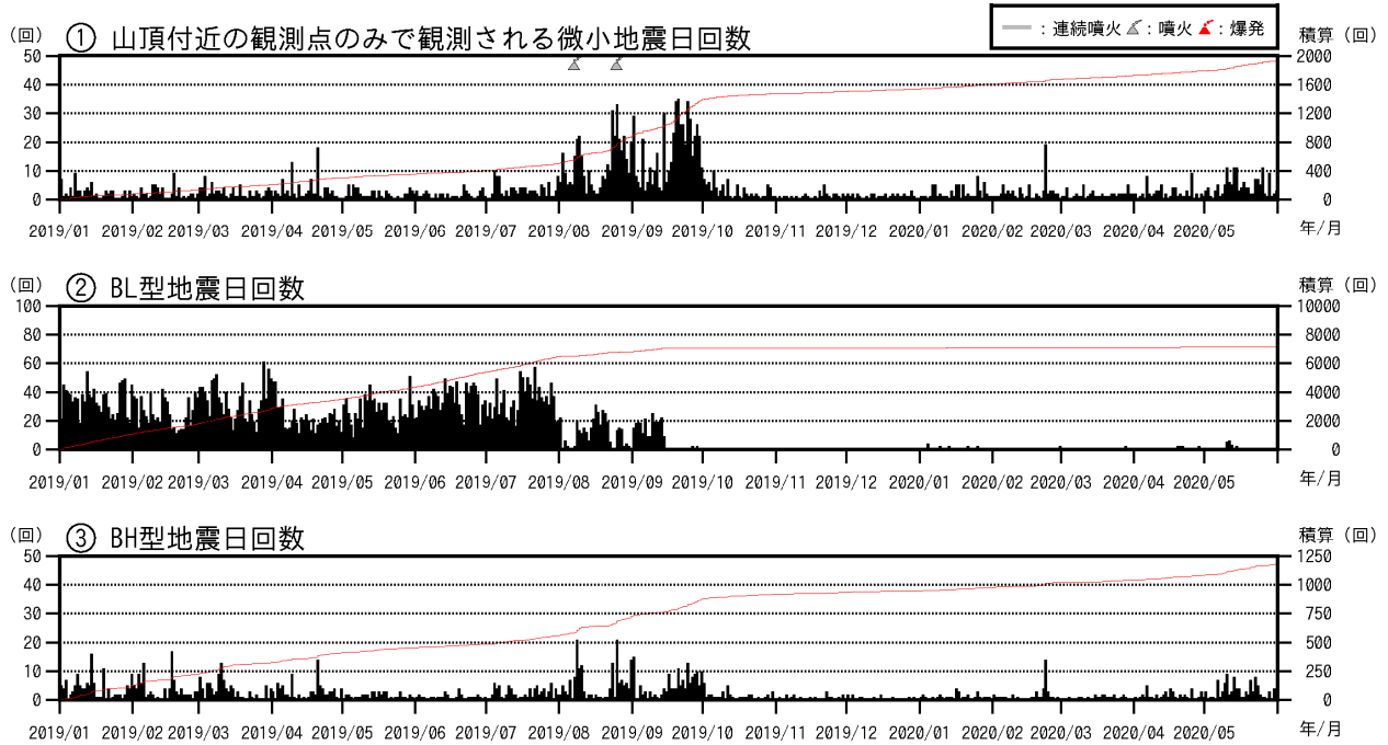
図5 浅間山 火山性地震の発生状況（2019年1月1日～2020年5月31日）
