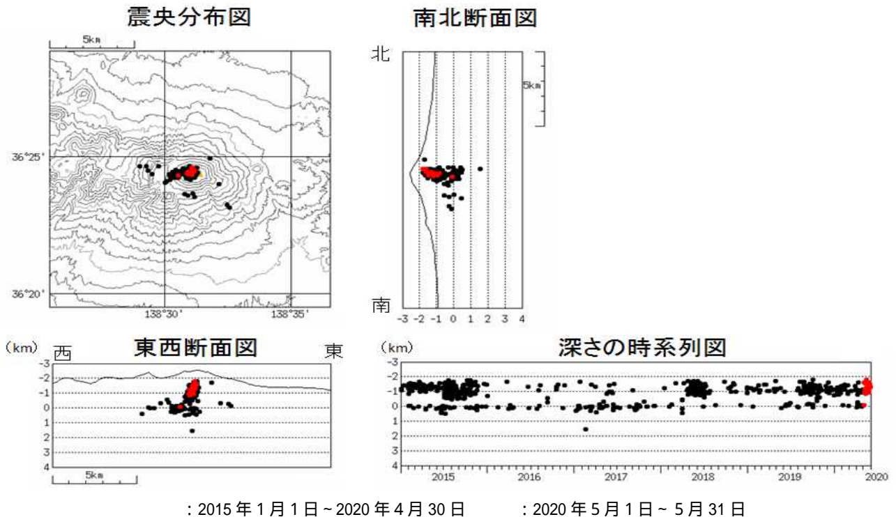
図6 浅間山 震源分布図（2015年1月1日～2020年5月31日）
