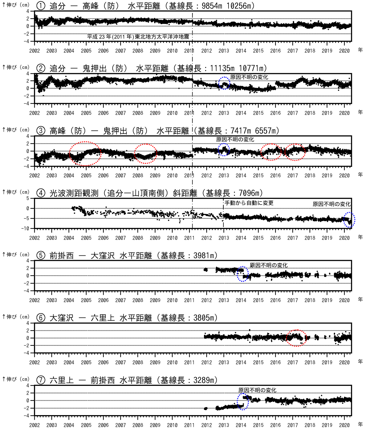
図7-1 浅間山 GNSS 連続観測及び光波測距観測の結果(2002年1月1日~2020年5月31日) 2010年10月及び2016年1月に、解析方法を変更しています。
