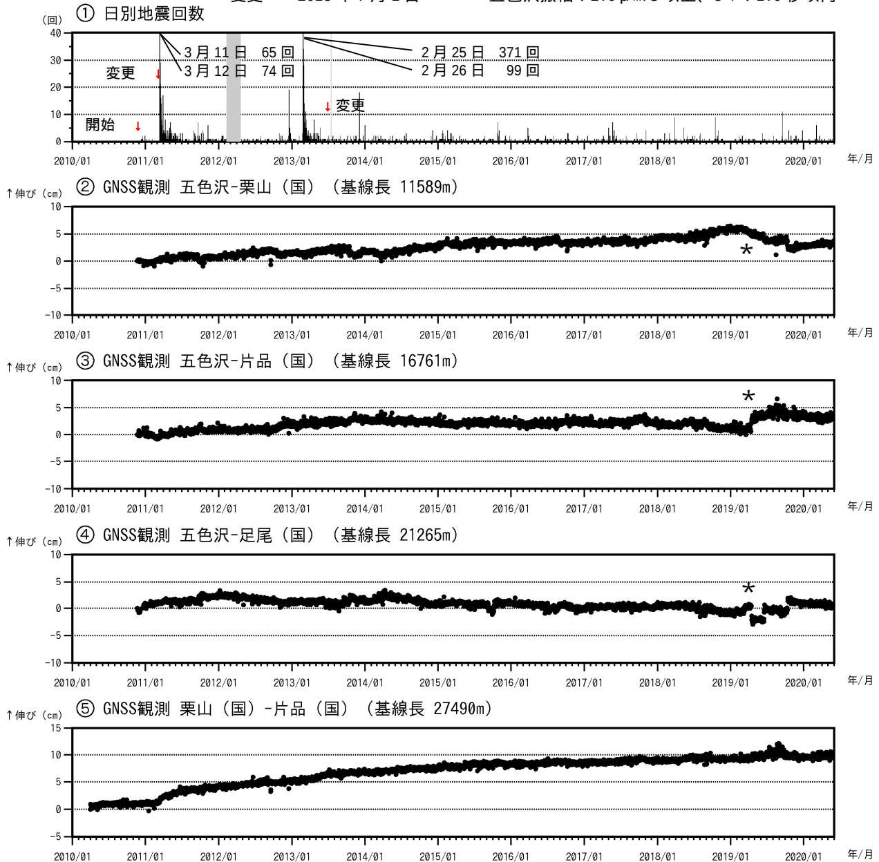
図2 日光白根山 火山活動経過図（2010年4月1日～2020年5月31日）
