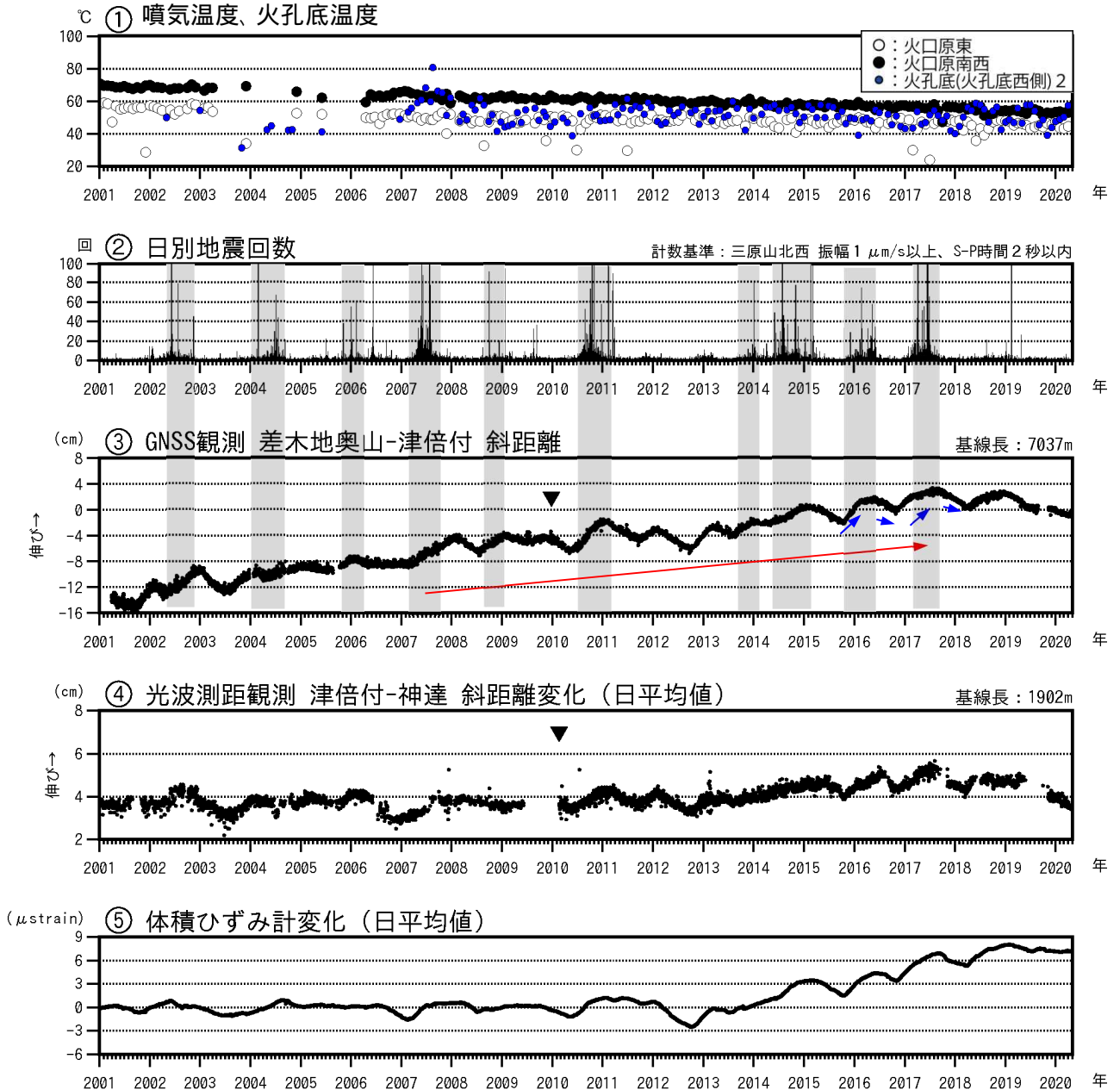
図2 伊豆大島 最近の火山活動経過図（2001年1月～2020年4月30日）
