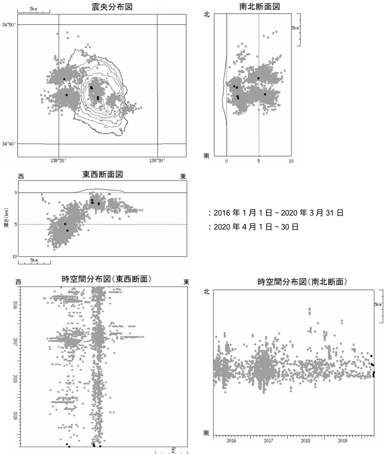
図4 伊豆大島 震源分布図（2016年1月1日～2020年4月30日）
