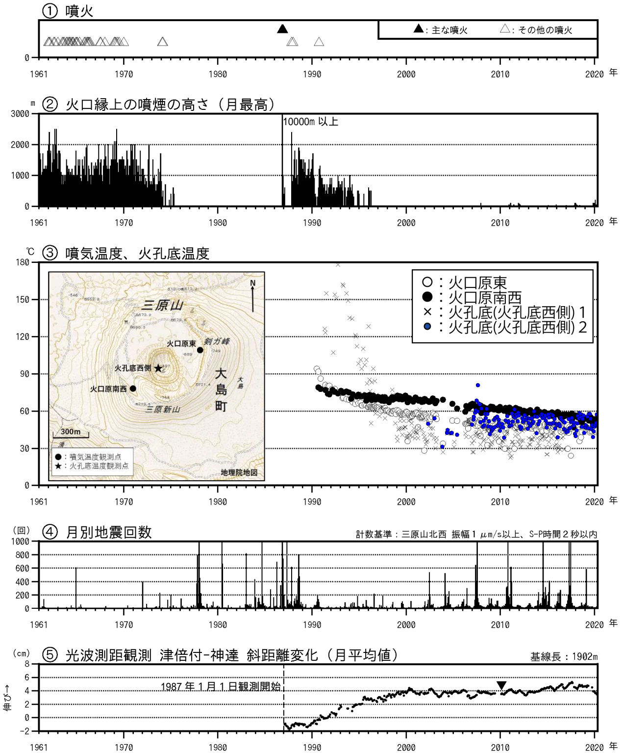
図1 伊豆大島 長期間の火山活動経過図（1961年1月～2020年4月30日） 1991年12月18日までは火口縁上130m以上、2002年2月28日までは火口縁上300m以上の噴煙の高さを観測していました。 火口原東、火口原南西：サーミスタ温度計により直接測定した噴気温度。 火口底（火口底西側）1：赤外放射温度計により離れた場所から測定した火口底温度。 火口底（火口底西側）2：赤外熱映像装置により離れた場所から測定した火口底温度。 地震回数には伊豆大島周辺海域で発生した地震も一部含まれています。 グラフの空白部分は欠測、△は機器更新。
