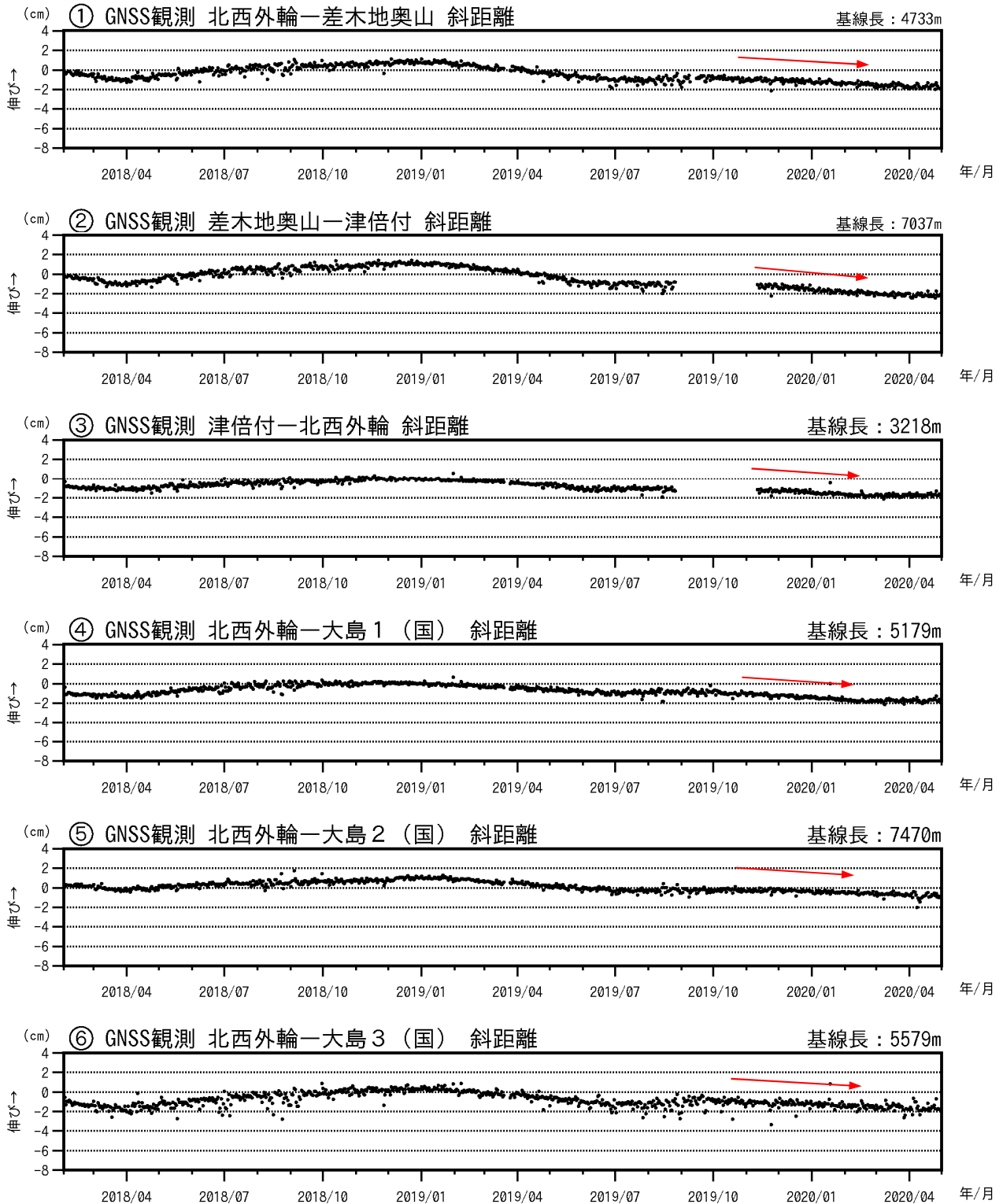
図3-2 伊豆大島 GNSS連続観測による基線長変化(2018年2月~2020年4月30日)
