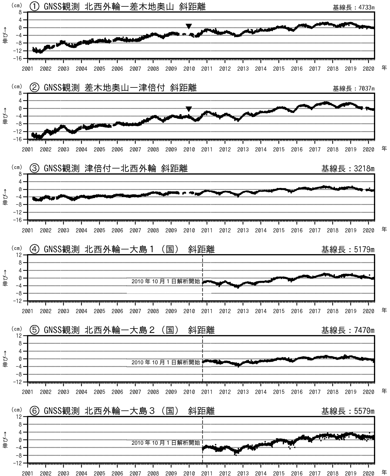
図3-1 伊豆大島 GNSS連続観測による基線長変化(2001年1月～2020年4月30日)
