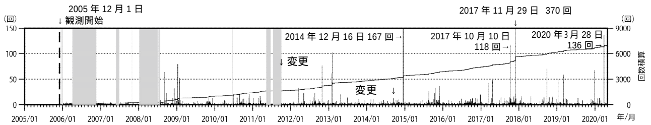
図3 白山 日別地震回数と積算回数（2005年12月1日～2020年4月30日）
