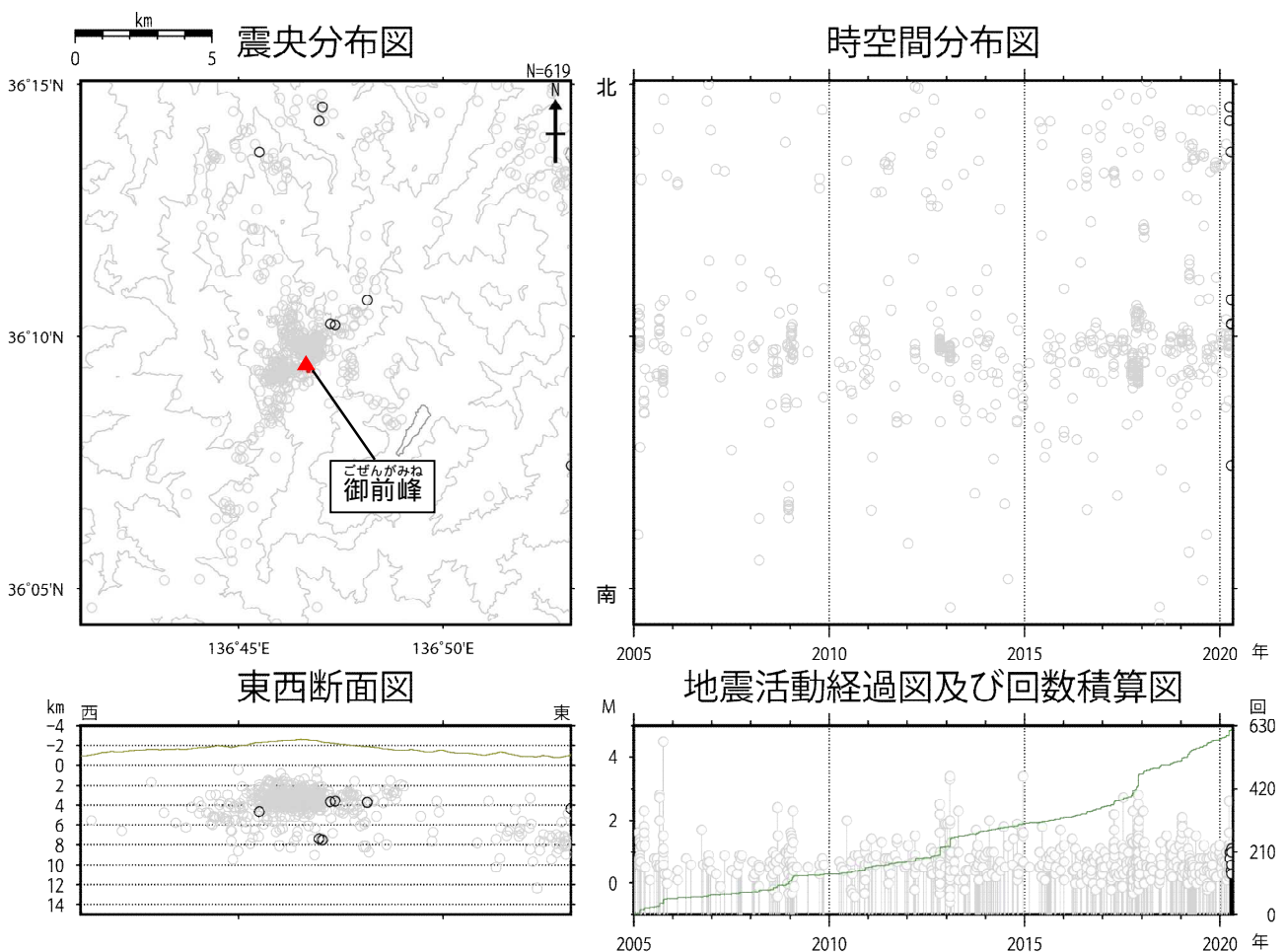
図4 白山 広域地震観測網による山体・周辺の地震活動（2005年1月1日～2020年4月30日）
