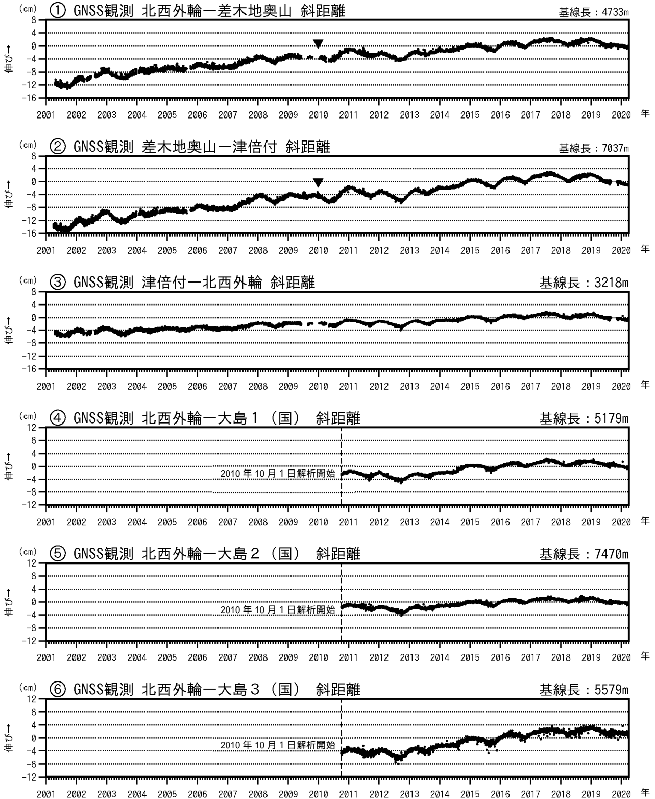
図3-1 伊豆大島 GNSS連続観測による基線長変化(2001年1月~2020年3月31日)
