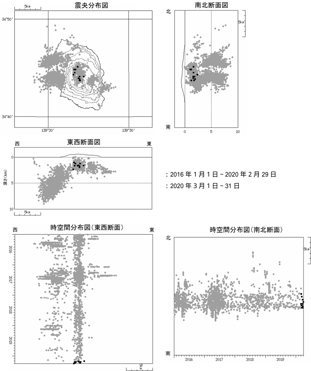
図4 伊豆大島 震源分布図（2016年1月1日～2020年3月31日） ・長期的には、地震活動は活発な時期と静穏な時期を繰り返しています。 ・今期間、震源は、三原山山頂付近の深さ1～2km付近に分布しました。
