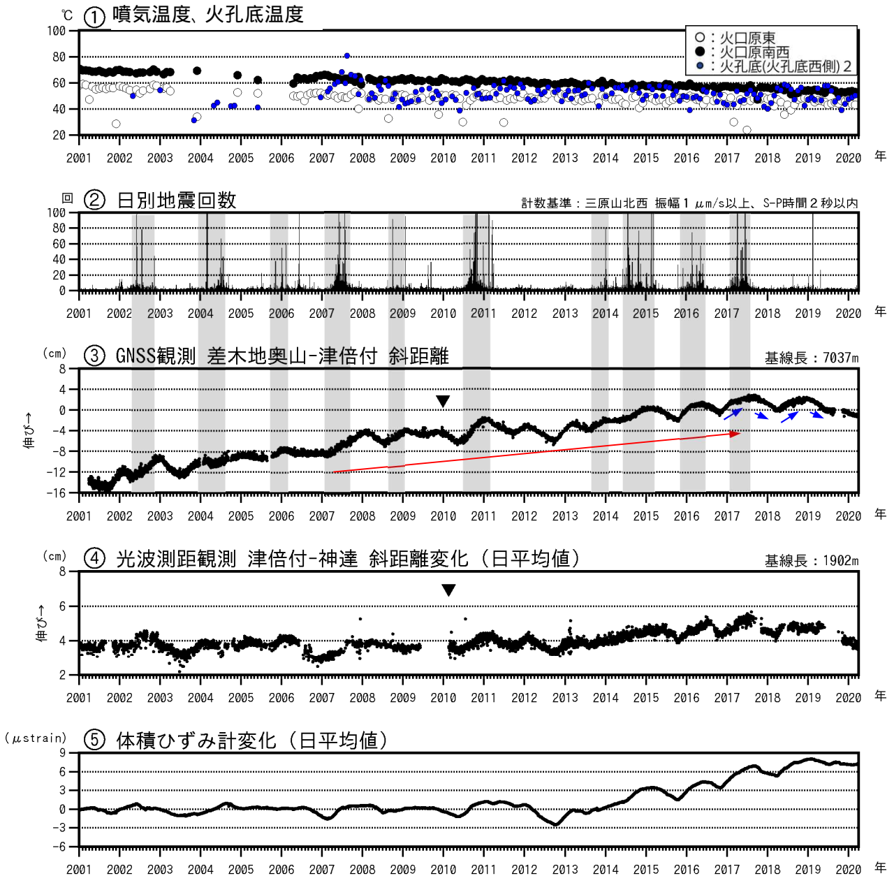
図2 伊豆大島 最近の火山活動経過図（2001年1月～2020年3月31日）
