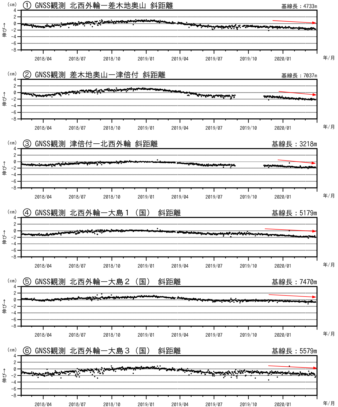
図3-2 伊豆大島 GNSS連続観測による基線長変化(2018年2月~2020年3月31日)
