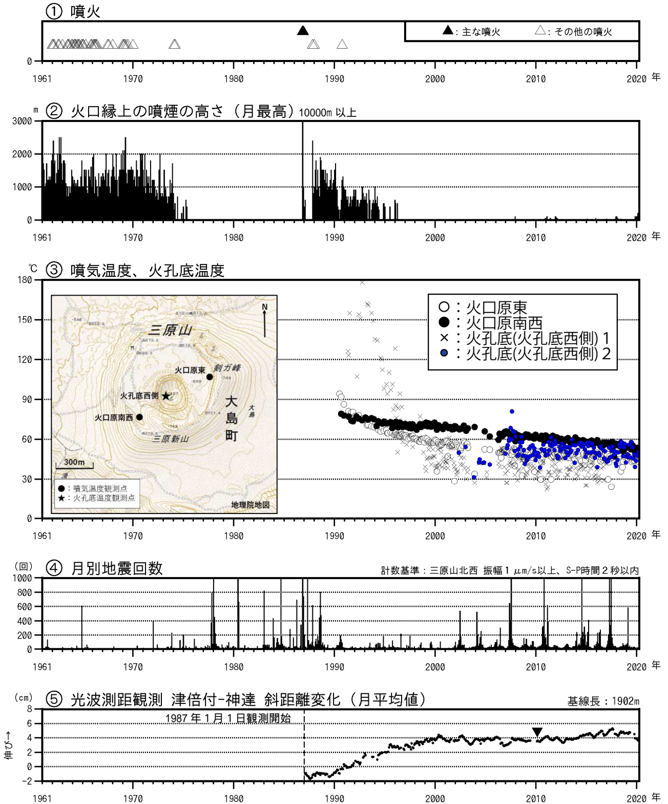
図1 伊豆大島 長期間の火山活動経過図（1961年1月～2020年3月31日）
