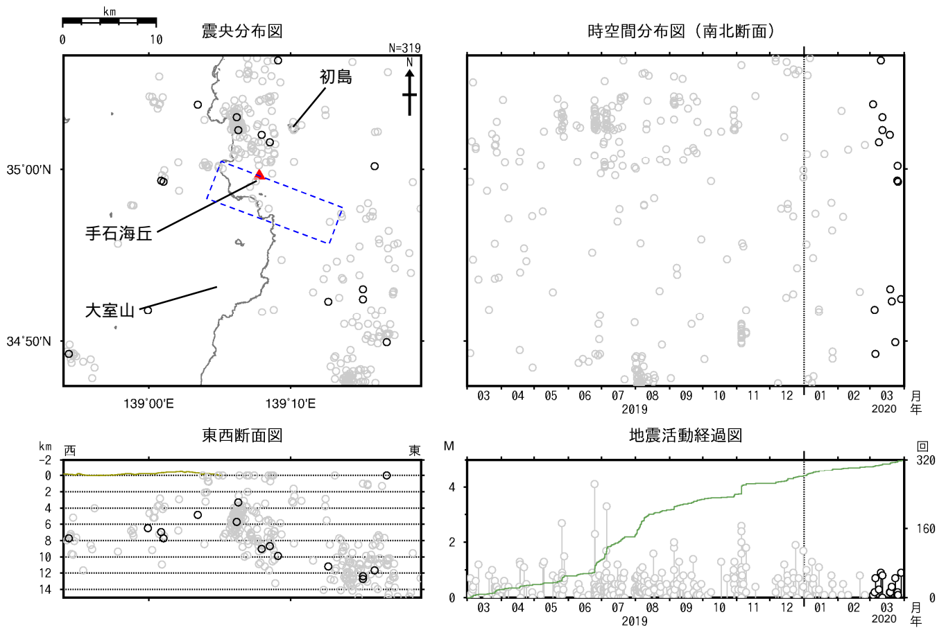
図2 伊豆東部火山群 広域地震観測網による震源分布図（2019年3月1日～2020年3月31日）
