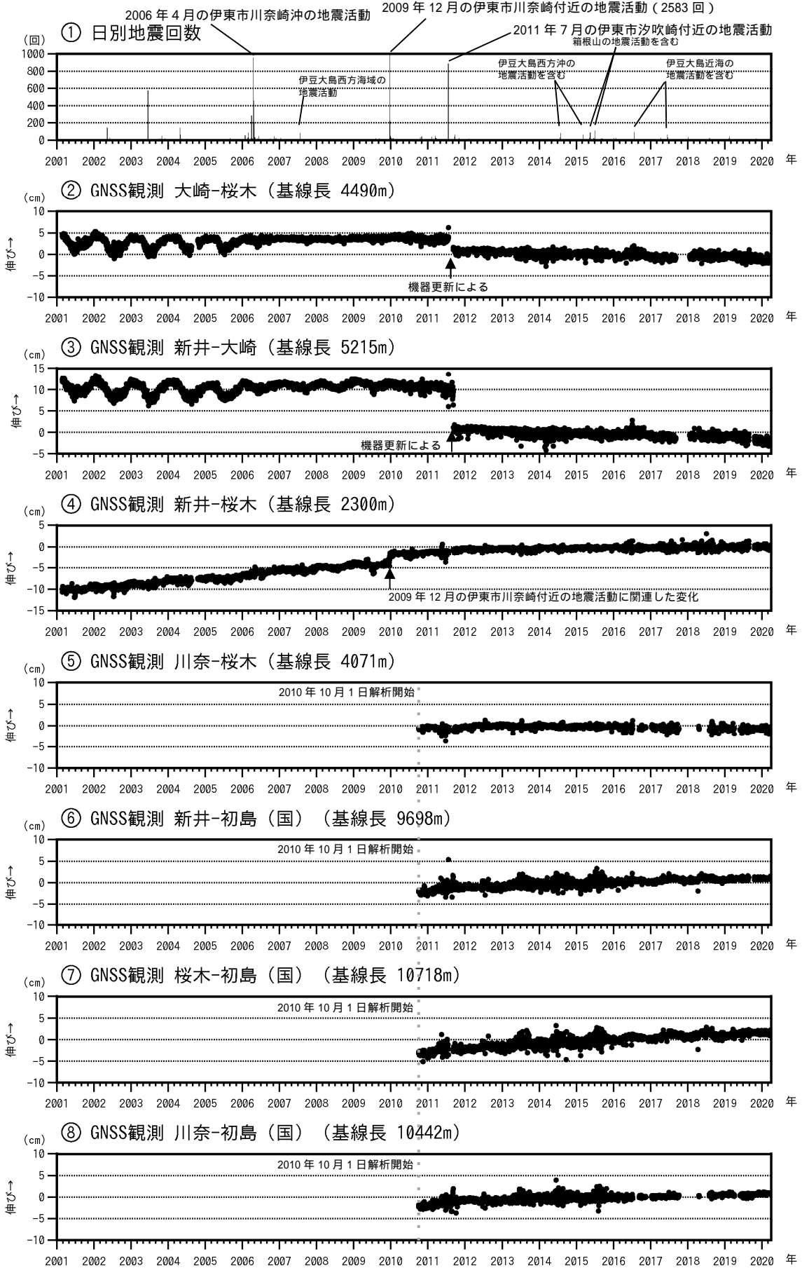
図3 伊豆東部火山群 火山活動経過図（2001年1月1日～2020年3月31日）
