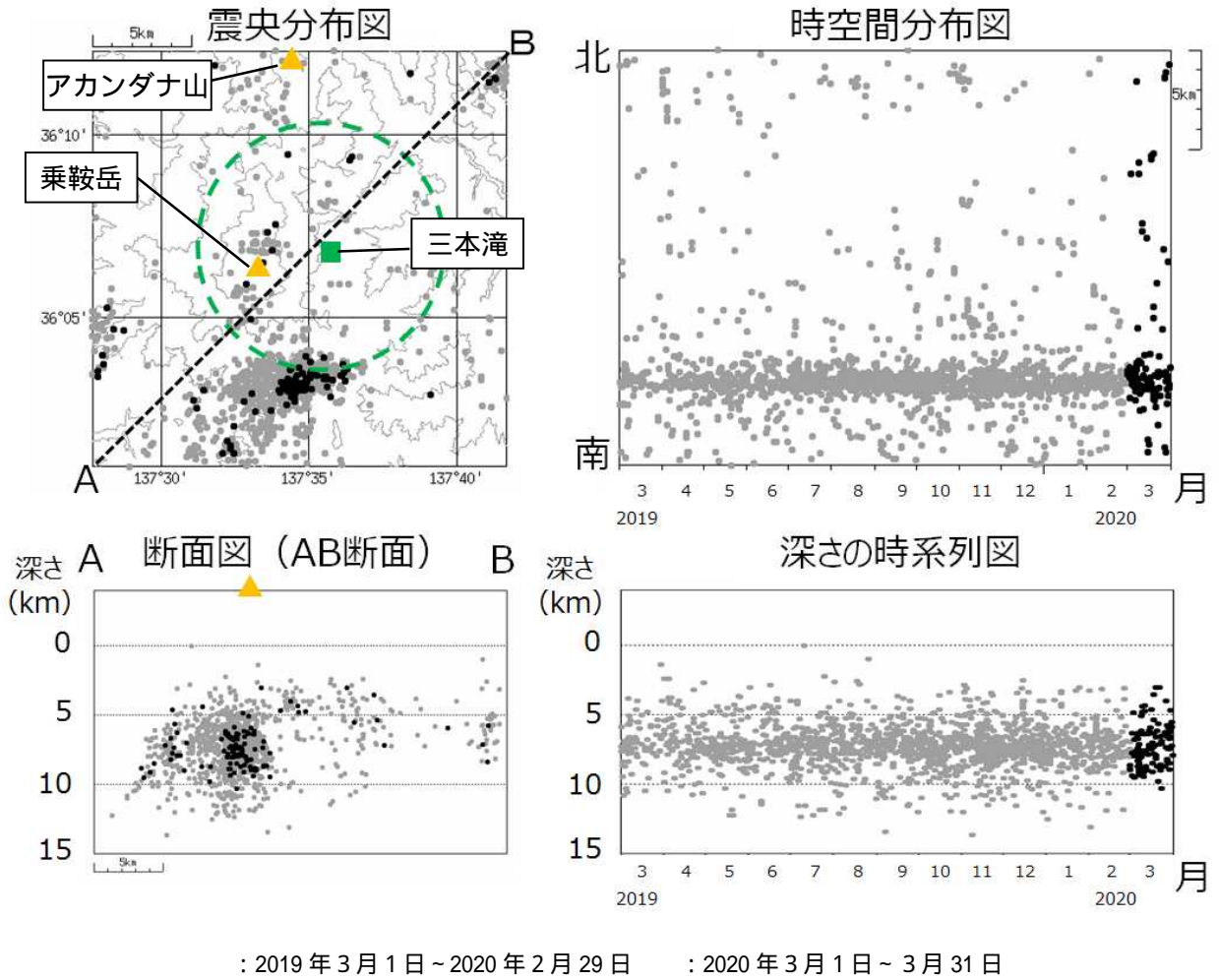
図3 乗鞍岳 広域地震観測網による山体・周辺の地震活動(2019年3月1日～2020年3月31日) 広域地震観測網により震源決定したもので、深さは全て海面以下として決定しています。図中の震源要素は一部暫定値が含まれており、後日変更することがあります。 震央分布図中の緑点線円は、図2 で計数される地震のおおよその範囲を示します。 ・乗鞍岳付近の地震活動は、低調に経過しています。
