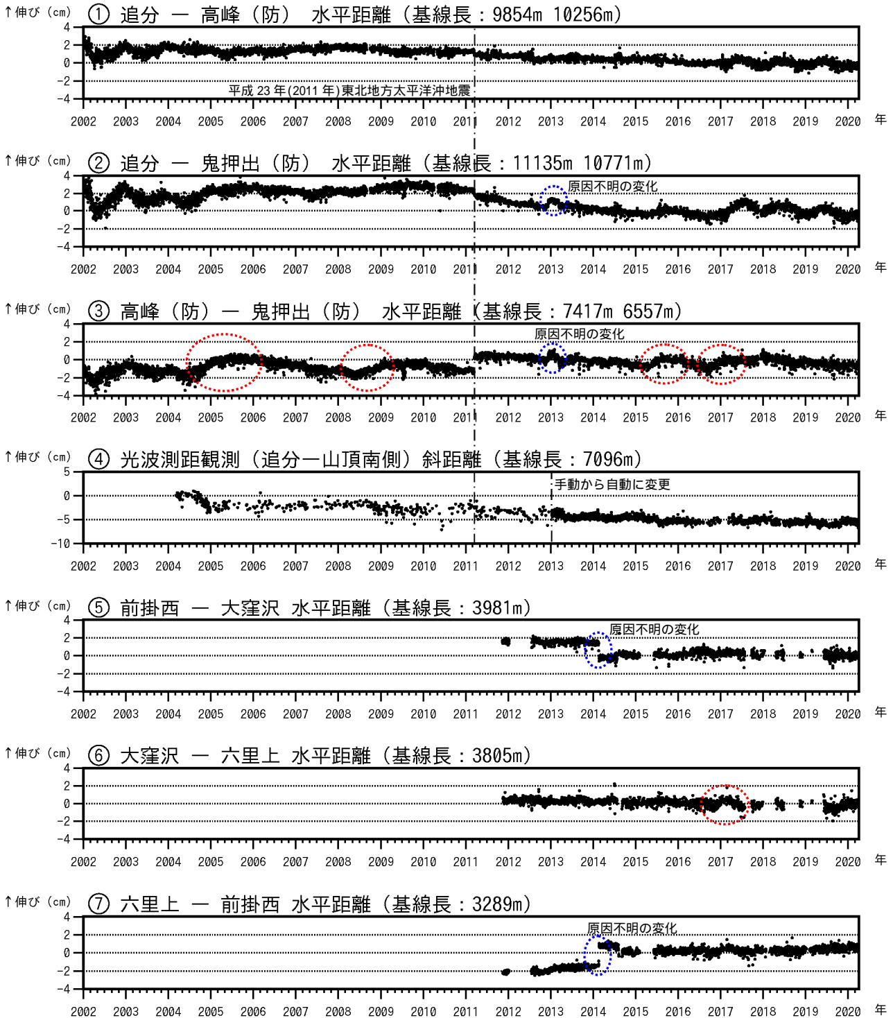
図7-1 浅間山 GNSS連続観測及び光波測距観測の結果(2002年1月1日~2020年3月31日) 2010年10月及び2016年1月に、解析方法を変更しています。
