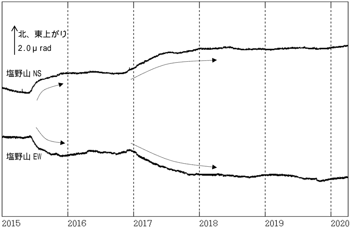
図9 浅間山 塩野山観測点における傾斜データ（2015年1月1日～2020年3月31日）
