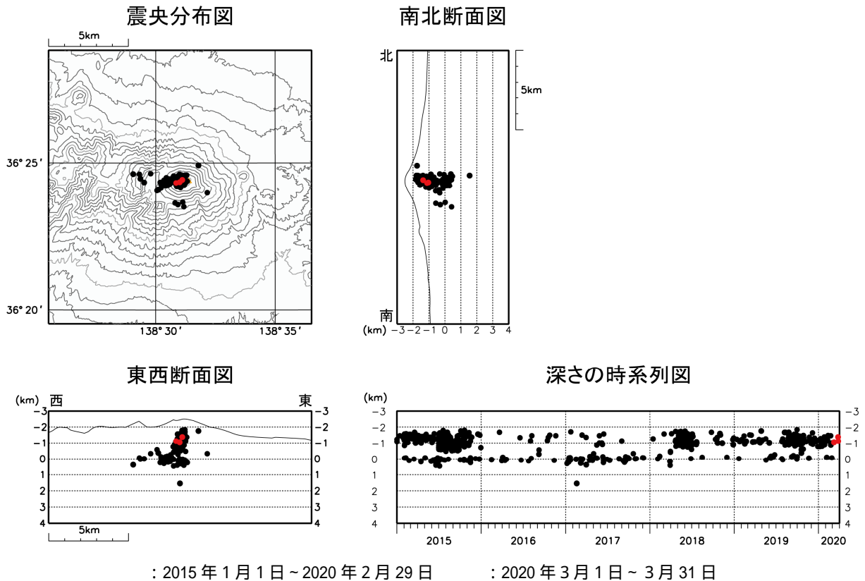
図6 浅間山 震源分布図（2015年1月1日～2020年3月31日）
