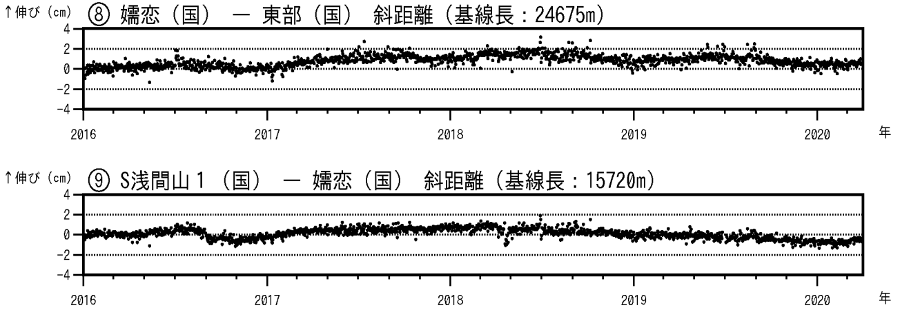
図7 - 2 浅間山 GNSS連続観測結果(2016年1月1日~2020年3月31日) (国): 国土地理院 、 は図8の にそれぞれ対応しています。 、 の空白部分は欠測を示します。
