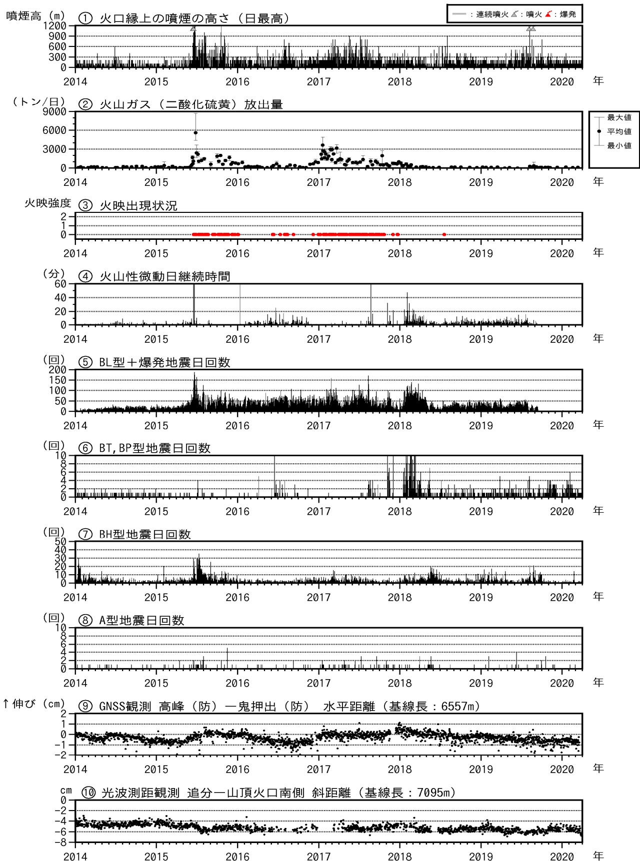
図4 浅間山 最近の火山活動経過図 (2014年1月1日~2020年3月31日)
