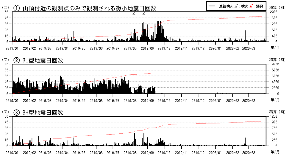
図5 浅間山 火山性地震の発生状況（2019年1月1日～2020年3月31日）
