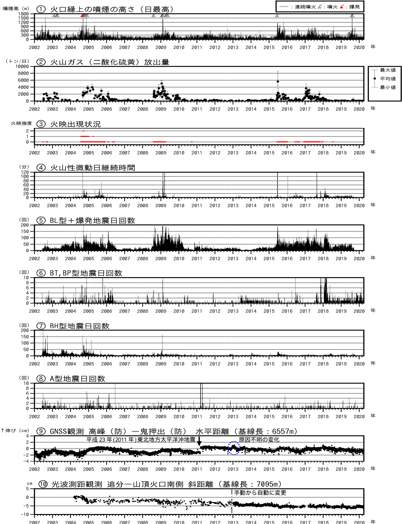
図3 浅間山 火山活動経過図（2002年1月1日～2020年3月31日）
