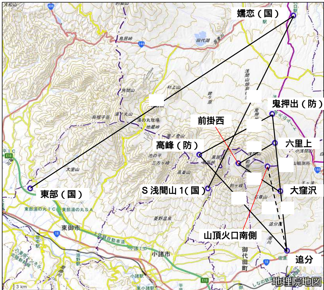
図8 浅間山 地殻変動連続観測点配置図 (防): 国立研究開発法人防災科学技術研究所、(国): 国土地理院 GNSS基線 は図3、図4の に対応しています。また、GNSS基線 ~ 及び ~ は図7の ~ 及び ~ にそれぞれ対応しています。 光波測距測線 は図3、図4の 、図7の に対応しています。
