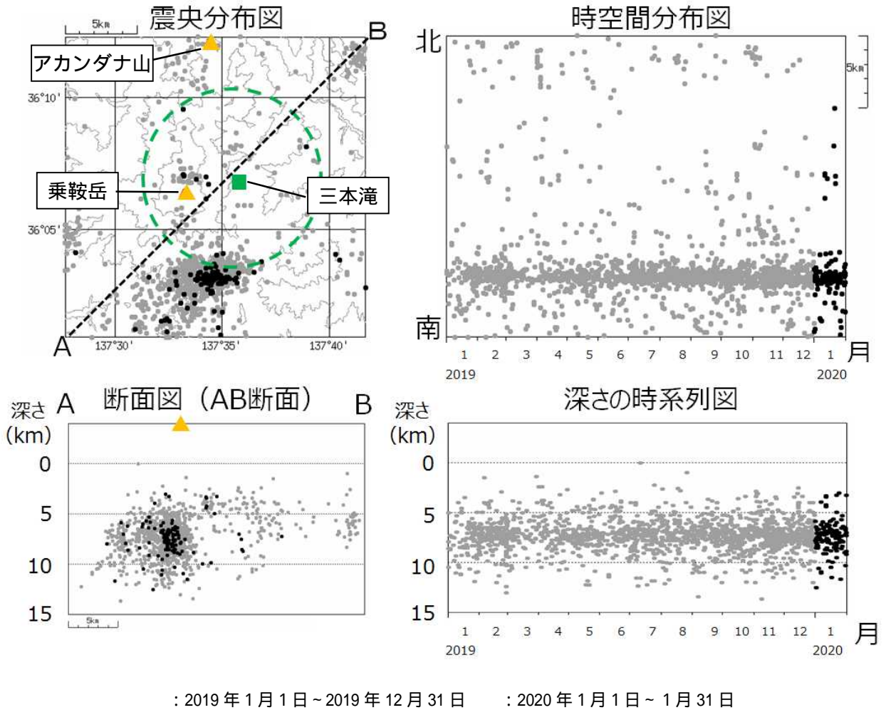
図3 乗鞍岳 広域地震観測網による山体・周辺の地震活動(2019年1月1日～2020年1月31日) 広域地震観測網により震源決定したもので、深さは全て海面以下として決定しています。図中の震源要素は一部暫定値が含まれており、後日変更することがあります。 震央分布図中の緑点線円は、図2 で計数される地震のおおよその範囲を示します。 ・乗鞍岳付近の地震活動は、低調に経過しています。 ・乗鞍岳から南方へ約6km離れたところでまとまった地震活動がみられますが、乗鞍岳の火山活動とは関係ないとみています。
